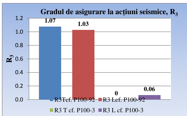
Figura 3 Gradul de asigurare la acțiuni seismice
