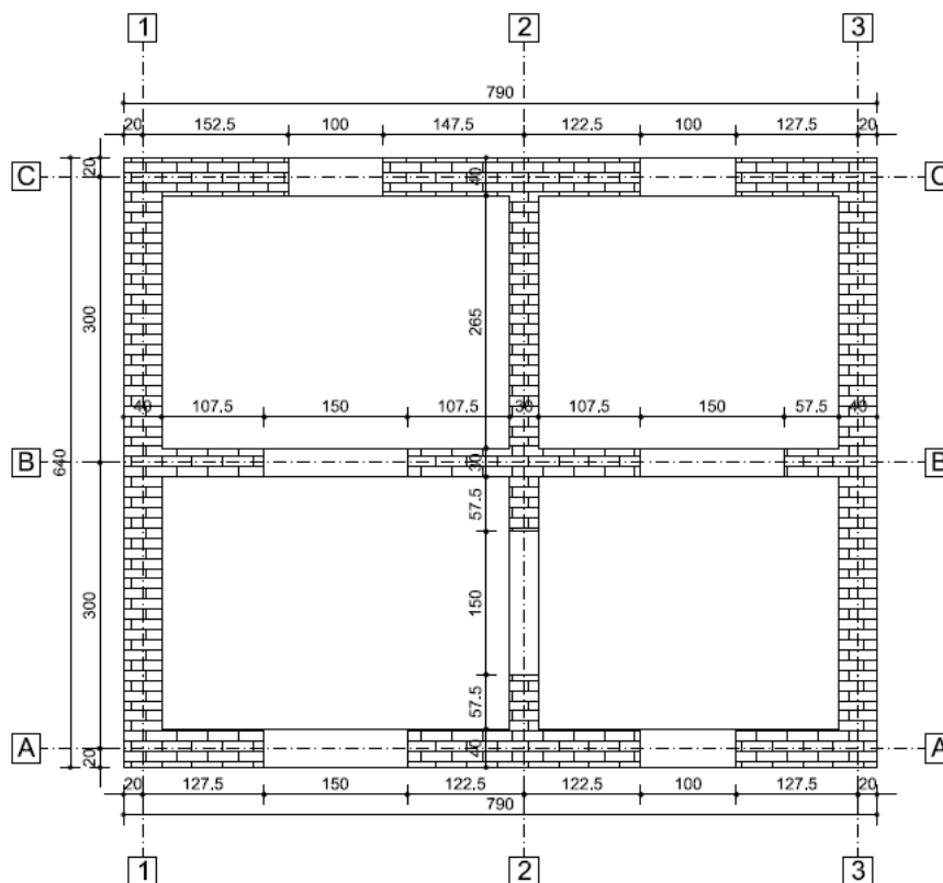
Figura 2. Plan nivel curent
