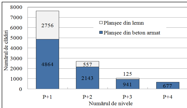
Figura 1. Municipiul București - repartitia clădirilor cu structura din zidărie de cărămidă în funcție de regimul de înălțime 7
