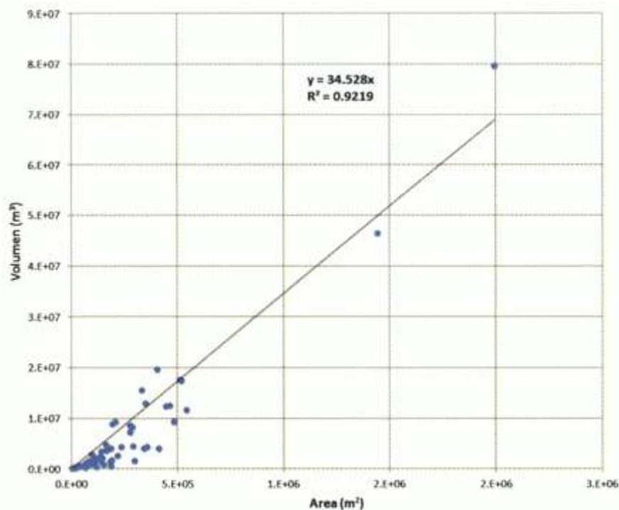
Figura 4: Relaciones superficie/volúmenes de los lagos en la cuenca del Santa y del Tablachaca (batimetría de 67 lagos en las cuencas del río Santa-fuente UGRH/ANA)
