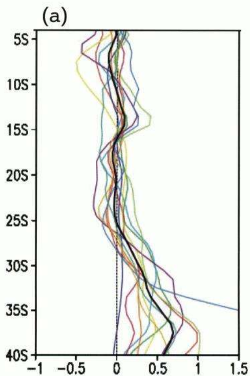
FIGURA A: PROYECCIONES DEL VIENTO COSTERO EN INVIERNO A LO LARGO DE LA COSTA DEL SISTEMA DE LA CORRIENTE DE HUMBOLDT SEGÚN LOS MODELOS GLOBALES DE CLIMA PARA EL ESCENARIO CLIMÁTICO EXTREMO CUADRUPPLICANDO LA CONCENTRACIÓN DE CO 2 EN LA ATMÓSFERA. LAS LÍNEAS DE COLOR INDICAN LOS DIFERENTES MODELOS CLIMÁTICOS Y LA LÍNEA NEGRA EL PROMEDIO DE LOS MODELOS. LA LÍNEA NARANJA INDICA EL MODELO IPSL-CM4 QUE FUE UTILIZADO EN LOS TRABAJOS DE REGIONALIZACIÓN [15].
