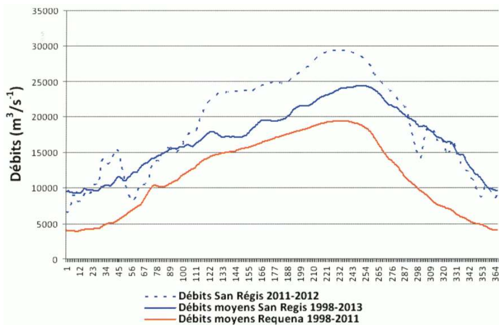
Figura 5: Ciclos hidrológicos promedios del Río Marañón en San Régis y del Ucayali en Requena y ciclo del Río Marañón en 2011-2012. Los caudales del Río Ucayali en 2011-2012, cerca de la normal, no son representados. Fuente de datos: HYBAM, adaptado de Espinoza et al. 2013
