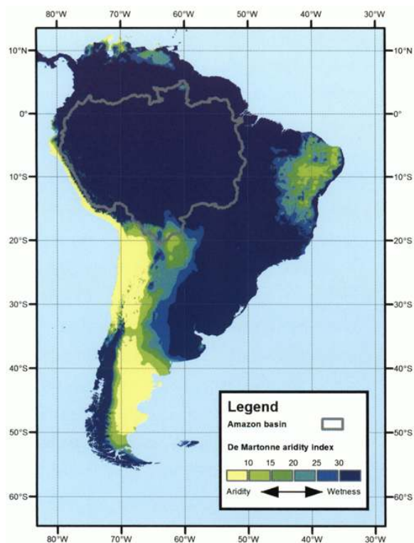
FIGURA 3B: PROYECCIÓN DE LOS VALORES DEL ÍNDICE DE ARIDEZ DE DE MARTONNE (DM) PARA EL AÑO 2080 SEGÚN EL ESCENARIO A2 Y EN BASE A LOS DATOS CLIMÁTICOS FUTUROS PROCEDENTES DE 19 MODELOS DE CIRCULACIÓN GENERAL (MCG). UN VALOR DM DE 10 SE CONSIDERA COMO EL LÍMITE SUPERIOR PARA CATEGORIZAR CLIMAS ÁRIDOS Y UN VALOR DE MÁS DE 30 POR LO GENERAL CARACTERIZA A LOS PAISAJES FORESTALES. DE ACUERDO CON ESTA PROYECCIÓN, LA CUENCA AMAZÓNICA DEBERÍA SER RELATIVAMENTE PRESERVADA DE LA ARIDEZ A LA EXCEPCIÓN DE SU PARTE MÁS MERIDIONAL.
