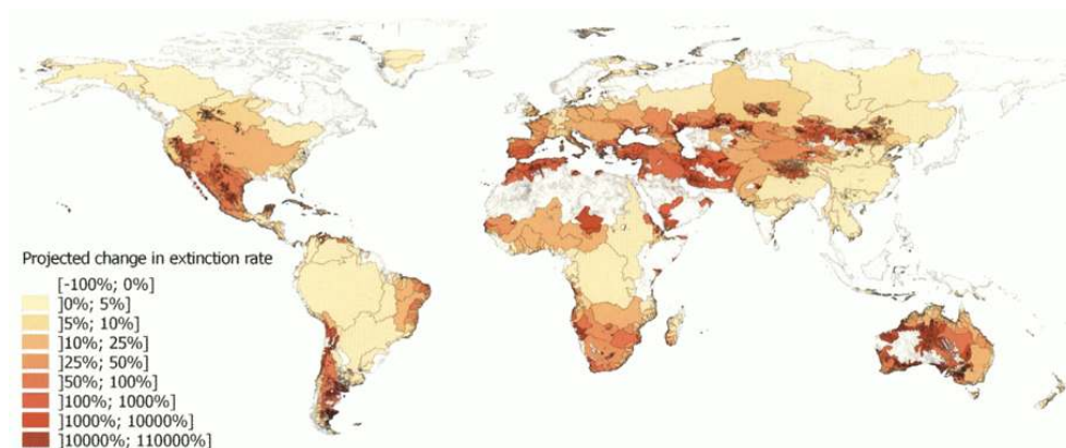
FIGURA 3A: PATRONES GLOBALES DE INCREMENTO O DISMINUCIÓN PROPORCIONALES DE LAS TASAS DE EXTINCIÓN ENTRE LAS CONDICIONES CLIMÁTICAS FUTURAS Y ACTUALES. LOS VALORES NEGATIVOS DEL CAMBIO PROYECTADO EN LA TASA DE EXTINCIÓN REPRESENTAN CUENCAS DONDE LAS TASAS DE EXTINCIÓN PUEDEN DISMINUIR, MIENTRAS QUE LOS VALORES POSITIVOS REPRESENTAN CUENCAS DONDE LAS TASAS DE EXTINCIÓN PUEDEN AUMENTAR. [6]
