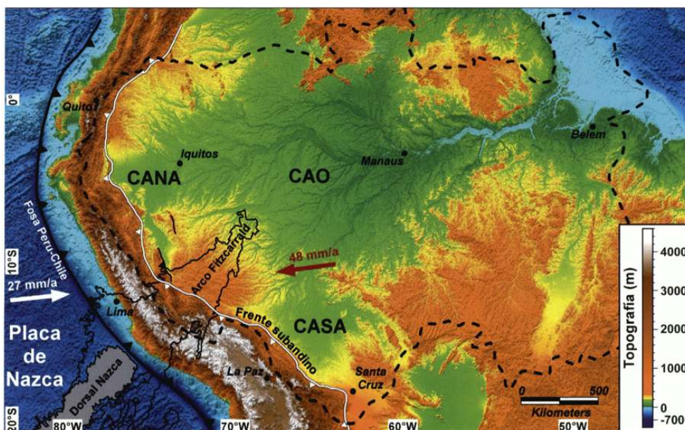
Figura 1: Modelo numérico de campo Tierra-Mar de los Andes y de la cuenca amazónica; CANA: Cuenca de Ante-país Nor Amazónica; CASA: Cuenca de Ante-país Sur Amazónica; CAO: Cuenca Amazónica Oriental (modificado según [15,27]).
