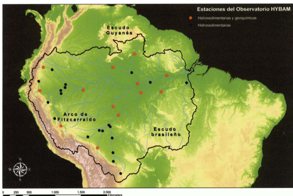
FIGURA 1: RED HIDROLÓGICA DEL OBSERVATORIO HYBAM EN LA CUENCA AMAZÓNICA: DESDE LOS PIEDEMONTES ANDINOS HASTA EL OCEANO ATLÁNTICO.
