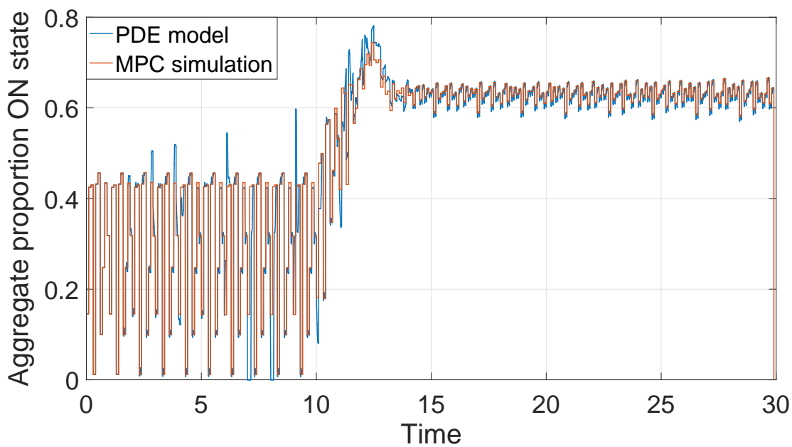
Figure 5.9 Comparaison de puissance consommée au cours du temps pour le modèle PDE et MPC, cas avec délai maximal de 2,5 unités de temps.
