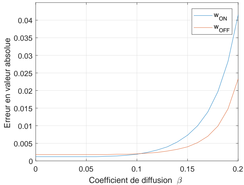
Figure 5.16 Erreur moyenne entre le modèle PDE et MPC en fonction du coefficient de diffusion pour une population homogène.
