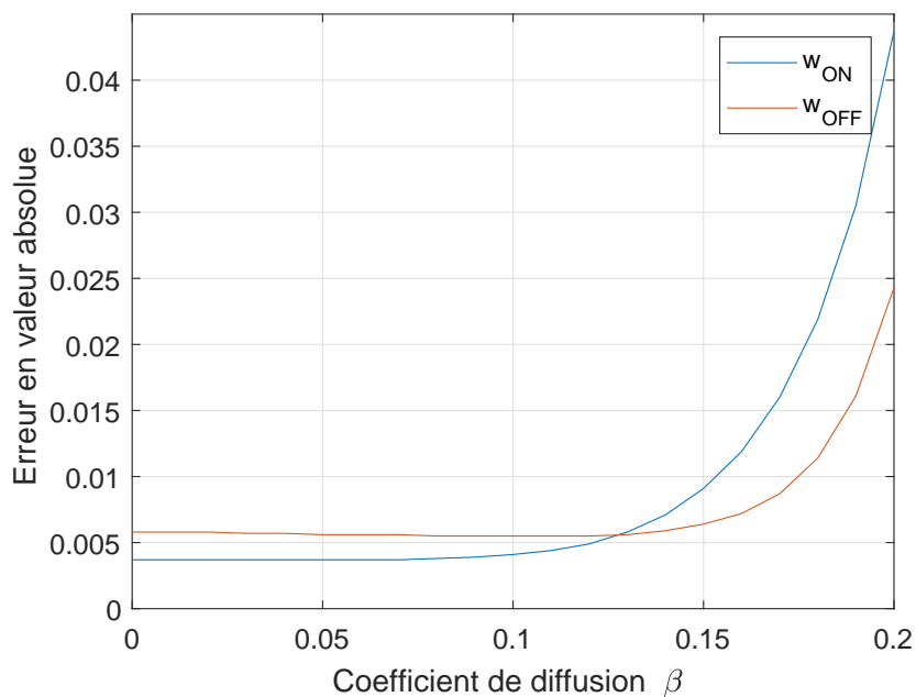
Figure 5.24 Erreur moyenne entre le modèle PDE et MPC en fonction du coefficient de diffusion pour une population hétérogène avec pénalisation aléatoire de l'effort de commande.
