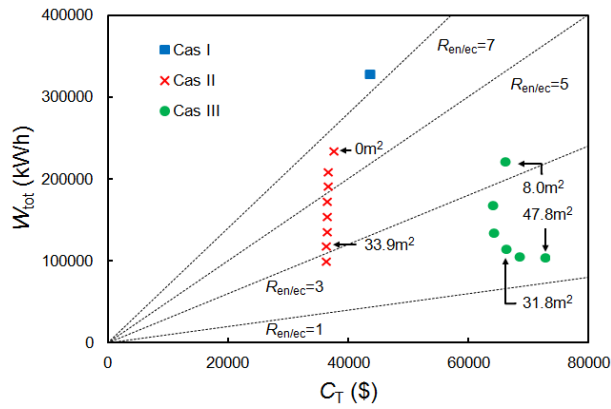
Figure 6.12 : W_{tot} vs C_T pour les cas d'études I à IV.
