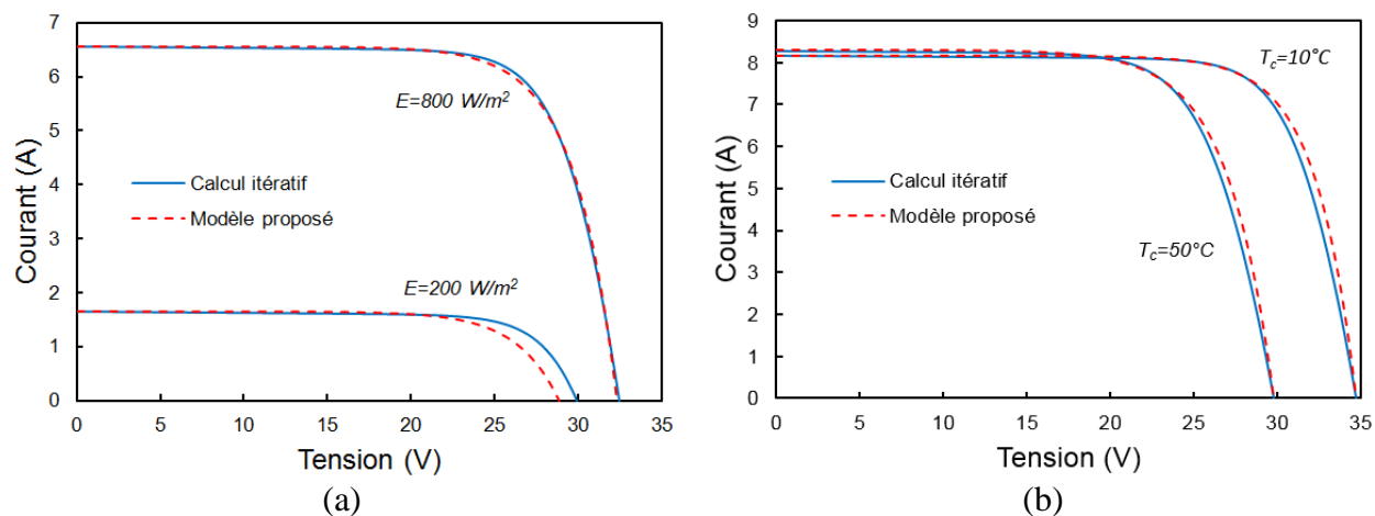
Figure 2.1 : Courbe caractéristique I-V pour le module KC200GT
