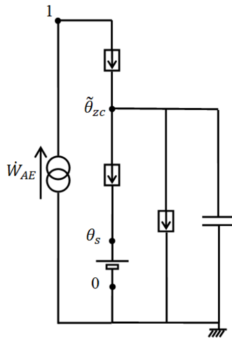
Figure 5.5 : Analogie exergétique-électrique du bâtiment avec appoint électrique.
