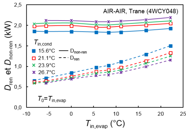
Figure 3.25 : Variations de la destruction d'exergie liée aux courants renouvelable et non renouvelable en fonction de T_{in,evap} à T_{in,cond} donnée pour la pompe à chaleur air-air de Trane® 10 4WCY4048 en mode chauffage et T_0 variable.
