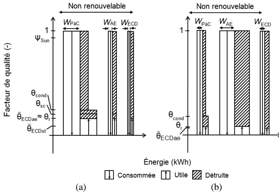
Figure 6.19 : Zoom sur les diagrammes exergetiques annuels des courants non renouvelables de : (a) la PaC solaire avec stockage de glace (T1GW025, S_{col}=31.8 \text{ m}^2 , V_{st,g}=25 \text{ m}^3 ) et (b) la PaC air-air avec panneaux PV (4WCY030, S_{PV}=33.9 \text{ m}^2 ).
