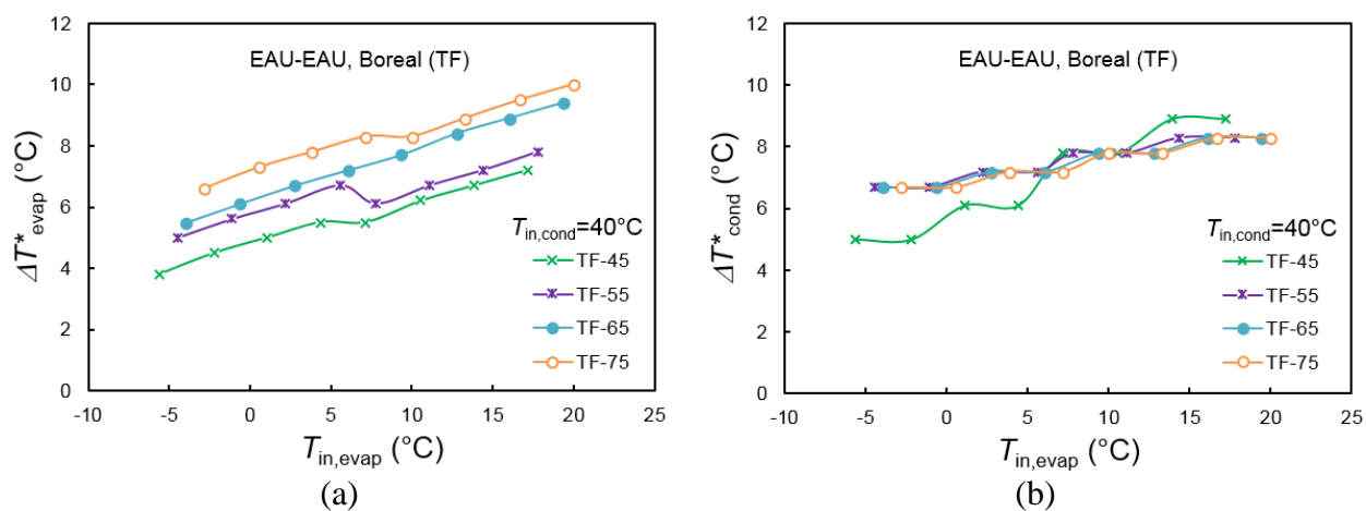
Figure A-9 : Variations de (a) \Delta T^*_{evap} et (b) \Delta T^*_{cond} en fonction de T_{in,evap} à T_{in,cond} = 40^\circ\text{C} pour la série TF eau-eau de Boreal® (TF-45,-55,-65,-75) en mode chauffage.
