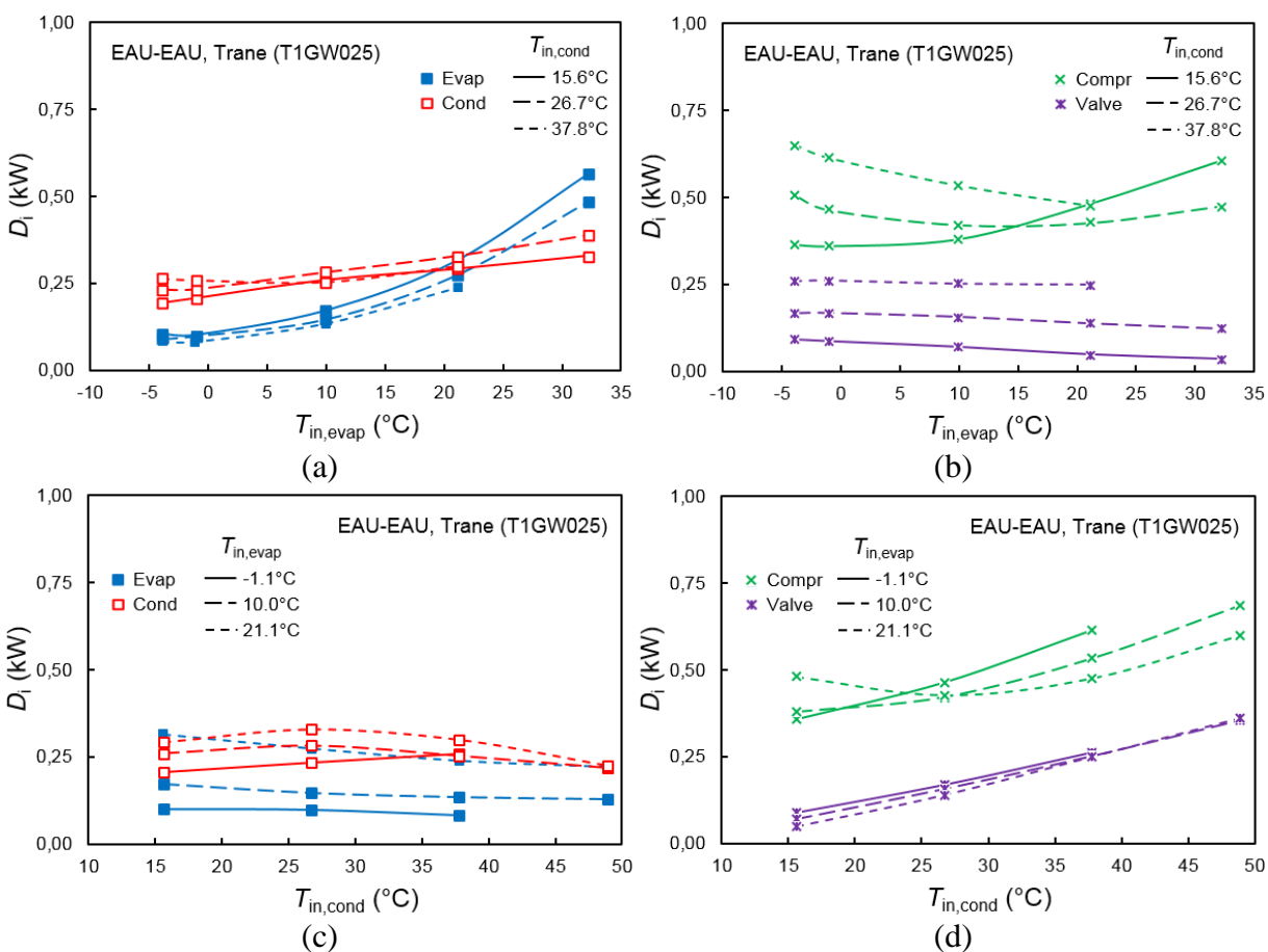
Figure A-26 : Variations de la destruction d'exergie dans les composants en fonction de T_{in,evap} à T_{in,cond} donnée et en fonction de T_{in,cond} à T_{in,evap} donnée pour la pompe à chaleur eau-eau de Trane® T1GW025 en mode chauffage.
