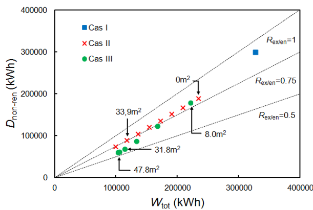
Figure 6.14 : D_{non-ren} vs W_{tot} pour les cas d'études I à IV.
