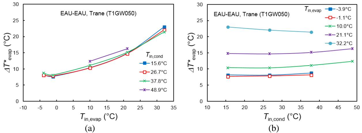
Figure 3.11 : Variations de \Delta T^*_{evap} en fonction de (a) T_{in, evap} à T_{in, cond} donnée et (b) T_{in, cond} à T_{in, evap} donnée pour la pompe à chaleur eau-eau de Trane® 10 T1GW050 en mode chauffage.
