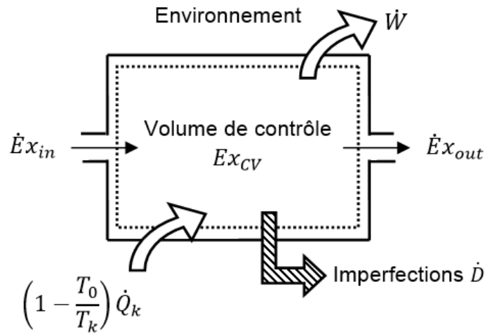
Figure 1.10 : Schéma du bilan d'exergie d'un volume de contrôle.
