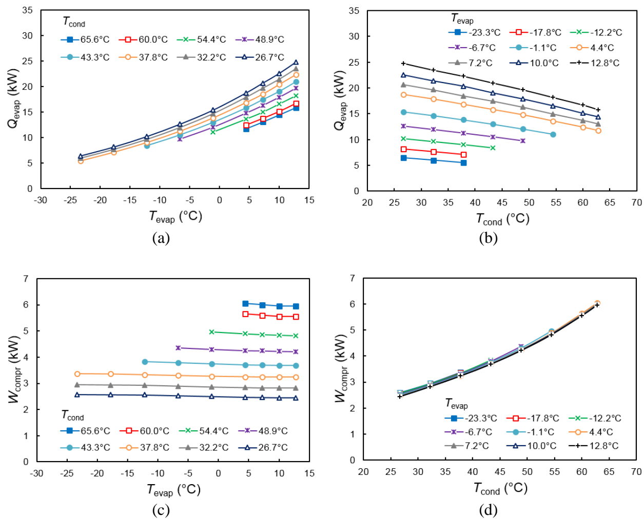
Figure 1.21 : Performances du compresseur Copeland™11 ZP51K5E-PFV.
