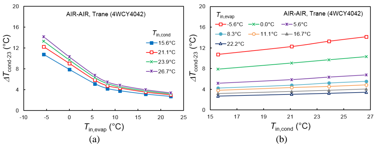
Figure A-33 : Variations de \Delta T_{cond-23} en fonction de (a) T_{in,evap} à T_{in,cond} donnée et (b) T_{in,cond} à T_{in,evap} donnée pour la pompe à chaleur air-air de Trane® 4WCY4042 en mode chauffage.
