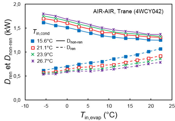
Figure A-39 : Variations de la destruction d'exergie liée aux courants renouvelable et non renouvelable en fonction de T_{in, evap} à T_{in, cond} donnée pour la pompe à chaleur air-air de Trane® 4WCY4042 en mode chauffage.
