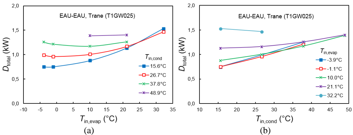
Figure A-24 : Variations de la destruction d'exergie totale en fonction de (a) T_{in, evap} à T_{in, cond} donnée et (b) T_{in, cond} à T_{in, evap} donnée pour la pompe à chaleur eau-eau de Trane® T1GW025 en mode chauffage.
