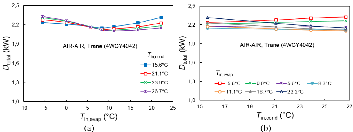
Figure A-35 : Variations de la destruction d'exergie dans les composants en fonction de T_{in,evap} à T_{in,cond} donnée pour la pompe à chaleur air-air de Trane® 4WCY4042 en mode chauffage.
