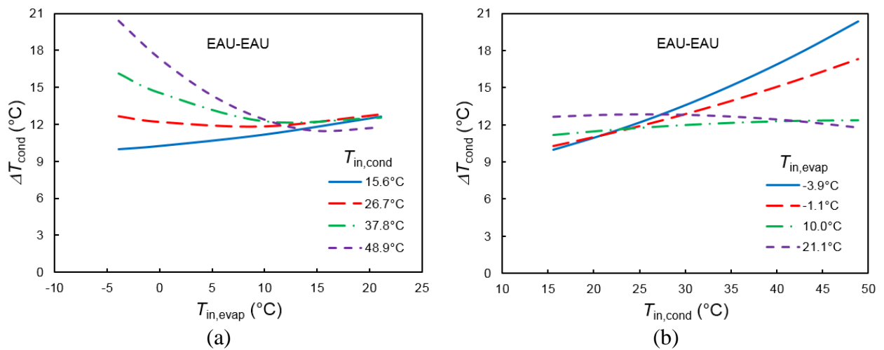
Figure 4.4 : Variations de \Delta T_{cond} en fonction de (a) T_{in,evap} et (b) T_{in,cond} avec l'approximation pour les pompes à chaleur eau-eau.
