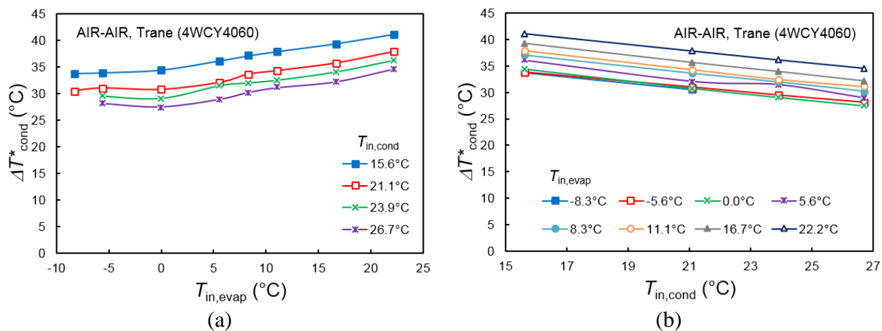
Figure A-32 : Variations de \Delta T^*_{cond} en fonction de (a) T_{in, evap} à T_{in, cond} donnée et (b) T_{in, cond} à T_{in, evap} donnée pour la pompe à chaleur air-air de Trane® 4WCY4060 en mode chauffage.
