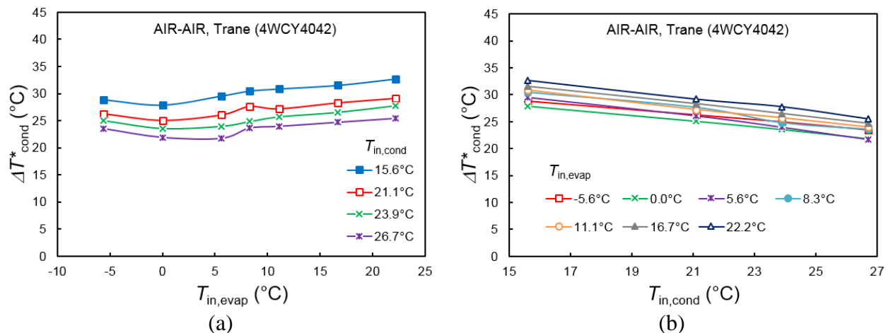
Figure A-31 : Variations de \Delta T^*_{cond} en fonction de (a) T_{in, evap} à T_{in, cond} donnée et (b) T_{in, cond} à T_{in, evap} donnée pour la pompe à chaleur air-air de Trane® 4WCY4042 en mode chauffage.
