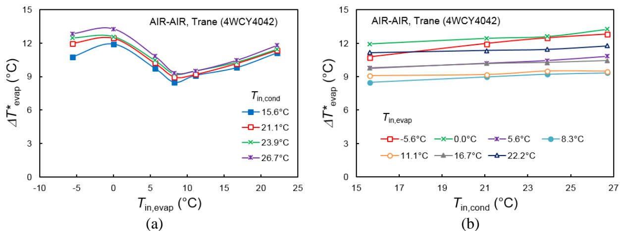
Figure A-29 : Variations de \Delta T^*_{evap} en fonction de (a) T_{in, evap} à T_{in, cond} donnée et (b) T_{in, cond} à T_{in, evap} donnée pour la pompe à chaleur air-air de Trane® 4WCY4042 en mode chauffage.
