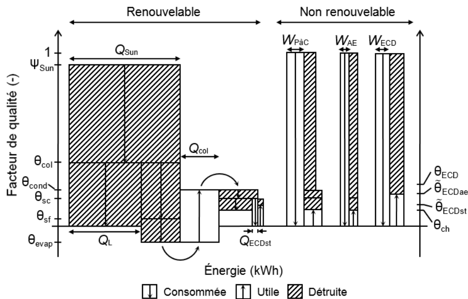
Figure 5.22 : Diagramme exergetique de la pompe à chaleur solaire avec stockage de glace.
