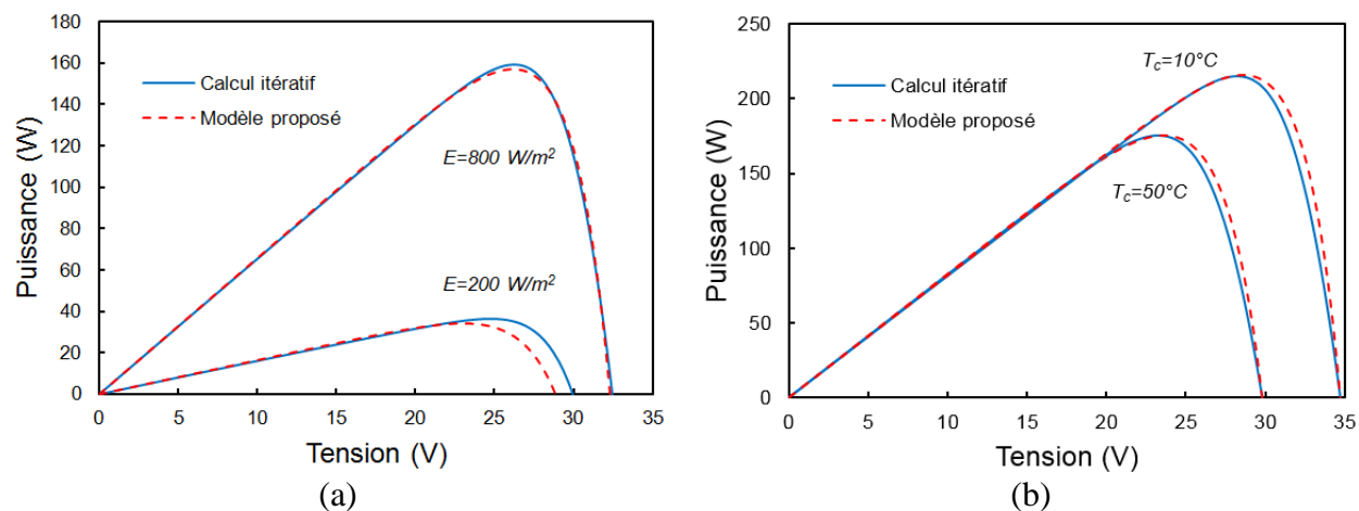
Figure 2.2 : Courbe de puissance P-V pour le module KC200GT
