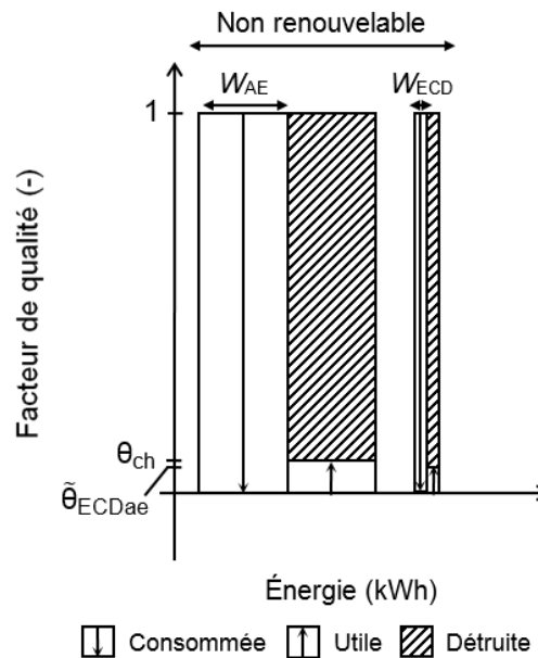
Figure 5.25 : Diagramme exergetique annuel du cas de référence (tout électrique).
