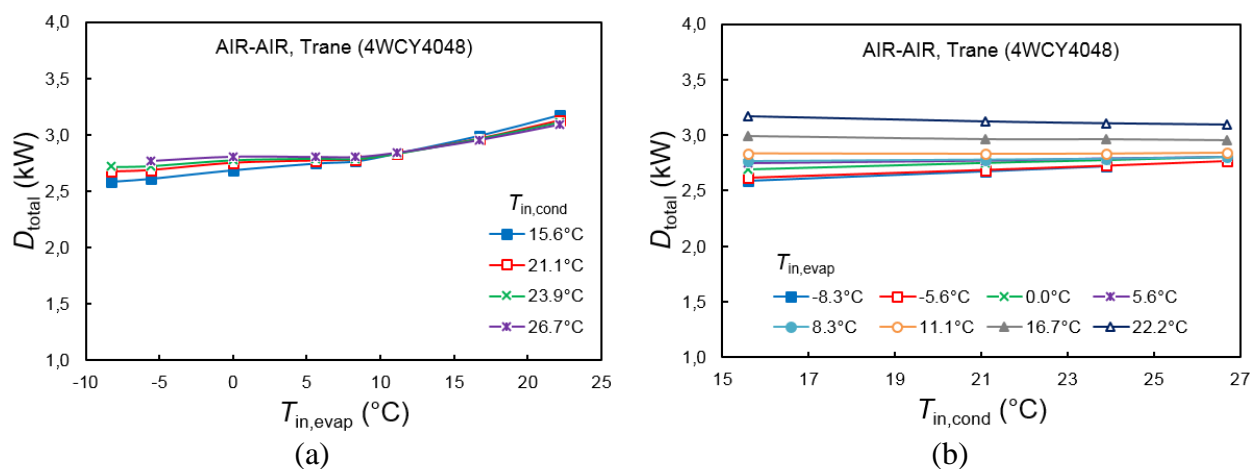
Figure 3.22 : Variations de la destruction d'exergie totale en fonction de (a) T_{in, evap} à T_{in, cond} donnée et (b) T_{in, cond} à T_{in, evap} donnée pour la pompe à chaleur air-air de Trane® 10 4WCY4048 en mode chauffage.
