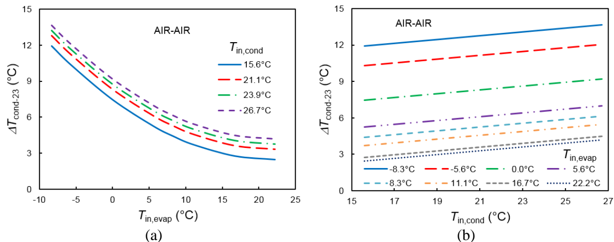
Figure 4.7 : Variations de \Delta T_{\text{cond-23}} en fonction de (a) T_{\text{in,evap}} et (b) T_{\text{in,cond}} avec l'approximation pour les pompes à chaleur air-air.
