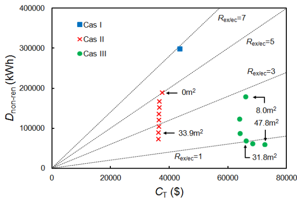
Figure 6.13 : D_{non-ren} vs C_T pour les cas d'études I à IV.
