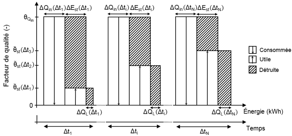
Figure 5.17 : Diagramme exergetique d'un systeme de stockage.
