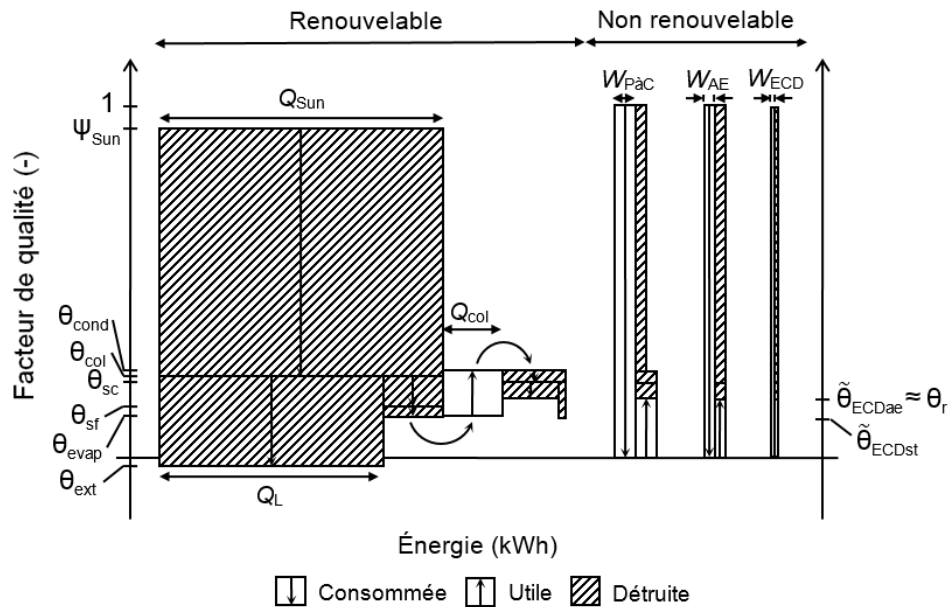
Figure 5.24 : Diagramme exergetique annuel de la pompe à chaleur solaire avec stockage de glace pour la pompe à chaleur T1GW050, S_{col}=31.8 \text{ m}^2 et V_{st,g}=25 \text{ m}^3 .
