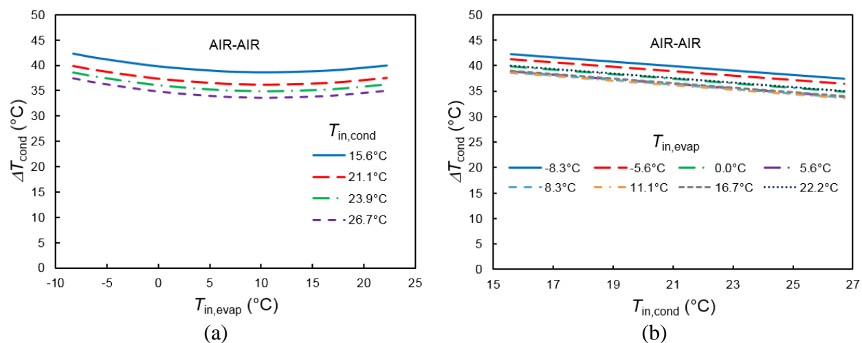
Figure 4.8 : Variations de \Delta T_{\text{cond}} en fonction de (a) T_{\text{in,evap}} et (b) T_{\text{in,cond}} avec l'approximation pour les pompes à chaleur air-air.
