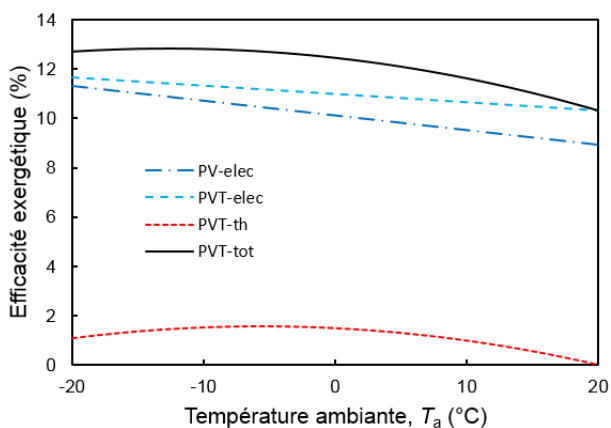
Figure 3.5 : Efficacité exergetique des systèmes PV et PV/T en fonction de la température ambiante pour E=500 \text{ W/m}^2 et T_{in}=18^\circ\text{C} .
