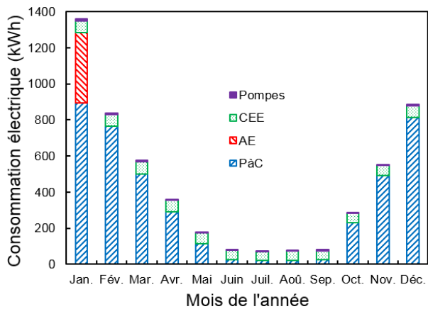
Figure A-57 : Consommation électrique des différents composants (pompe à chaleur, appoint électrique du réservoir, chauffe-eau électrique, pompes) pour la période de chauffage avec les modèles proposés et la pompe à chaleur T1GW050 et aucun temps de fonctionnement minimal.
