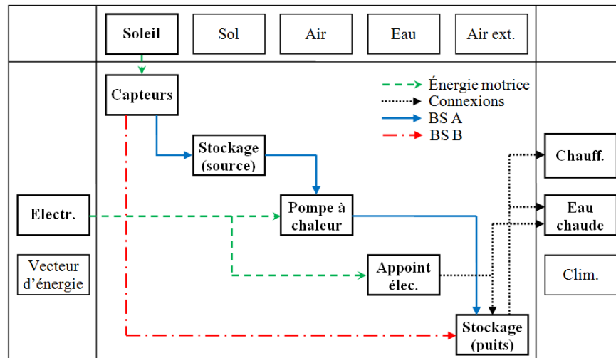
Figure 5.1 : Schéma de Frank et al. [170] appliqué à la pompe à chaleur solaire avec stockage de glace.
