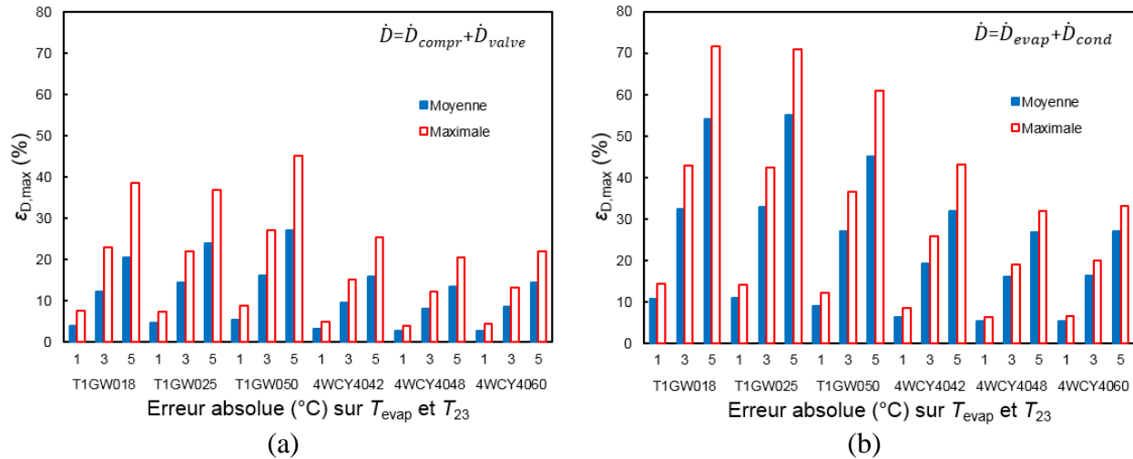
Figure 3.10 : Sensibilité de la destruction exergetique vis-à-vis des températures pour (a) le compresseur et la valve et (b) l'évaporateur et le condenseur.
