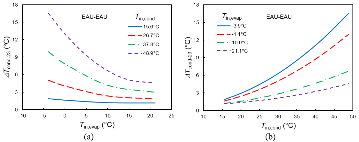
Figure 4.3 : Variations de \Delta T_{cond-23} en fonction de (a) T_{in,evap} et (b) T_{in,cond} avec l'approximation pour les pompes à chaleur eau-eau.
