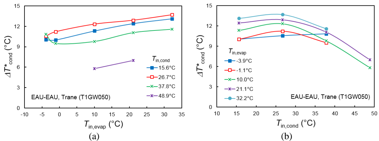
Figure 3.12 : Variations de \Delta T^*_{cond} en fonction de (a) T_{in, evap} à T_{in, cond} donnée et (b) T_{in, cond} à T_{in, evap} donnée pour la pompe à chaleur eau-eau de Trane® 10 T1GW050 en mode chauffage.
