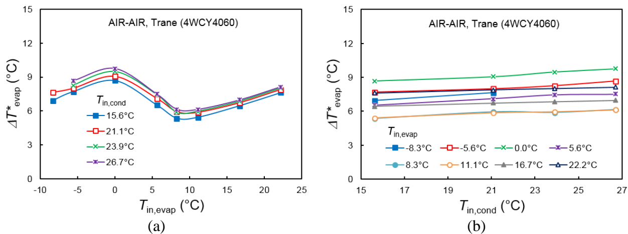
Figure A-30 : Variations de \Delta T^*_{evap} en fonction de (a) T_{in, evap} à T_{in, cond} donnée et (b) T_{in, cond} à T_{in, evap} donnée pour la pompe à chaleur air-air de Trane® 4WCY4060 en mode chauffage.
