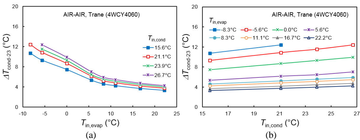
Figure A-34 : Variations de \Delta T_{cond-23} en fonction de (a) T_{in,evap} à T_{in,cond} donnée et (b) T_{in,cond} à T_{in,evap} donnée pour la pompe à chaleur air-air de Trane® 4WCY4060 en mode chauffage.
