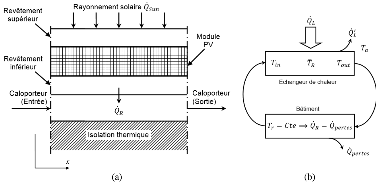
Figure 3.2 : (a) Schéma simplifié du système PV/T et (b) diagramme des flux de chaleur de l'unité de récupération de chaleur.
