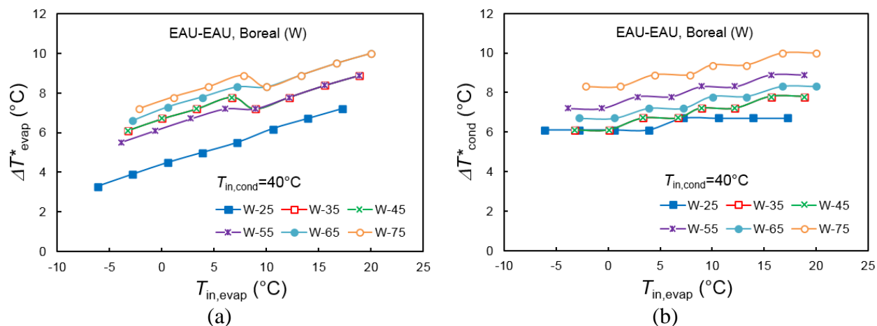
Figure A-8 : Variations de (a) \Delta T^*_{evap} et (b) \Delta T^*_{cond} en fonction de T_{in,evap} à T_{in,cond} = 40^\circ\text{C} pour la série W eau-eau de Boreal® (W-25,-35,-45,-55,-65,-75) en mode chauffage.
