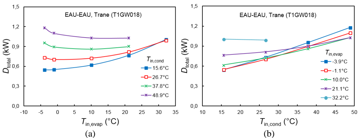
Figure A-23 : Variations de la destruction d'exergie totale en fonction de (a) T_{in, evap} à T_{in, cond} donnée et (b) T_{in, cond} à T_{in, evap} donnée pour la pompe à chaleur eau-eau de Trane® T1GW018 en mode chauffage.
