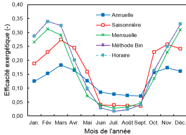
Figure 5.11 : Efficacité exergetique mensuelle de la pompe à chaleur solaire avec stockage de glace pour plusieurs températures de références avec T_{1GW050} , S_{col}=31.8 \text{ m}^2 et V_{st,g}=25 \text{ m}^3 .
