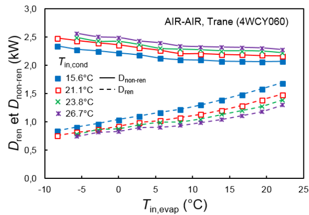
Figure A-40 : Variations de la destruction d'exergie liée aux courants renouvelable et non renouvelable en fonction de T_{in, evap} à T_{in, cond} donnée pour la pompe à chaleur air-air de Trane® 4WCY4060 en mode chauffage.
