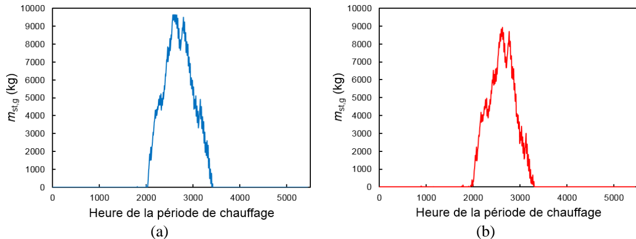
Figure 4.22 : Comparaison de l'évolution de la masse de glace pour la période de chauffage obtenue (a) avec les modèles proposés et (b) par Tamasauskas et al. [51].
