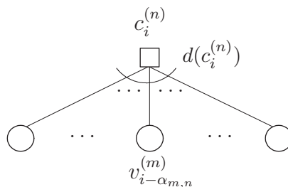
FIGURE 3.9 Sous-graphe induit par les variables apparaissant dans la n -ième équations de contraintes à l'instant i .
