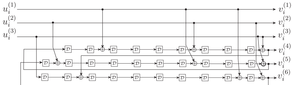
FIGURE 2.6 Exemple d'un codeur convolutionnel récursif composé de 3 registres en parallèle et d'un taux de codage 3/6.
