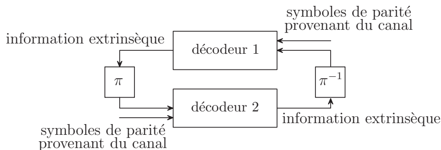
FIGURE 2.3 Exemple schématique d'un décodeur pour les codes Turbo.
