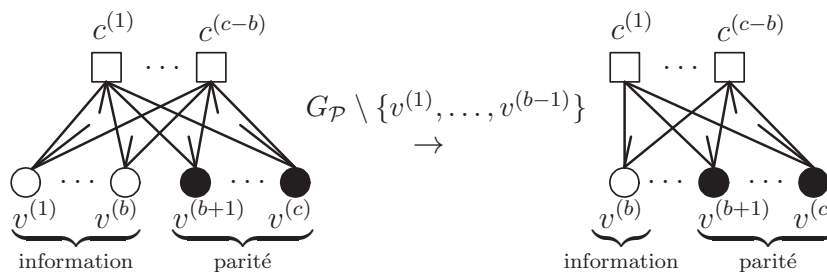
FIGURE 6.2 À gauche, le protographe général G_{\mathcal{P}} d'un ensemble de codes RCDO. À droite, le protographe imbriqué \tilde{G}_{\mathcal{P}(b-1)} qui correspond au sous-graphe induit G_{\mathcal{P}} \setminus \{v^{(1)}, \dots, v^{(b-1)}\} .
