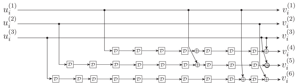
FIGURE 2.5 Exemple d'un codeur convolutionnel non récursif composé de 3 registres en parallèle et d'un taux de codage 3/6.
