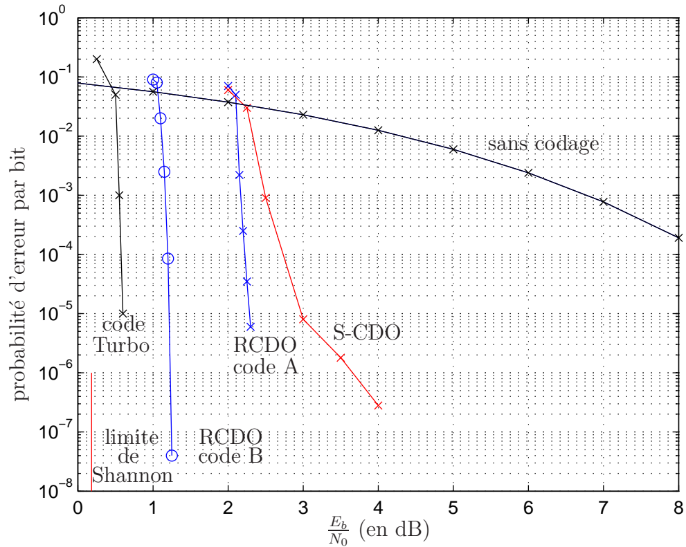
FIGURE 2.7 Comparaison des performances d'erreur entre différentes familles de codes convolutionnels de taux de codage 1/2.
