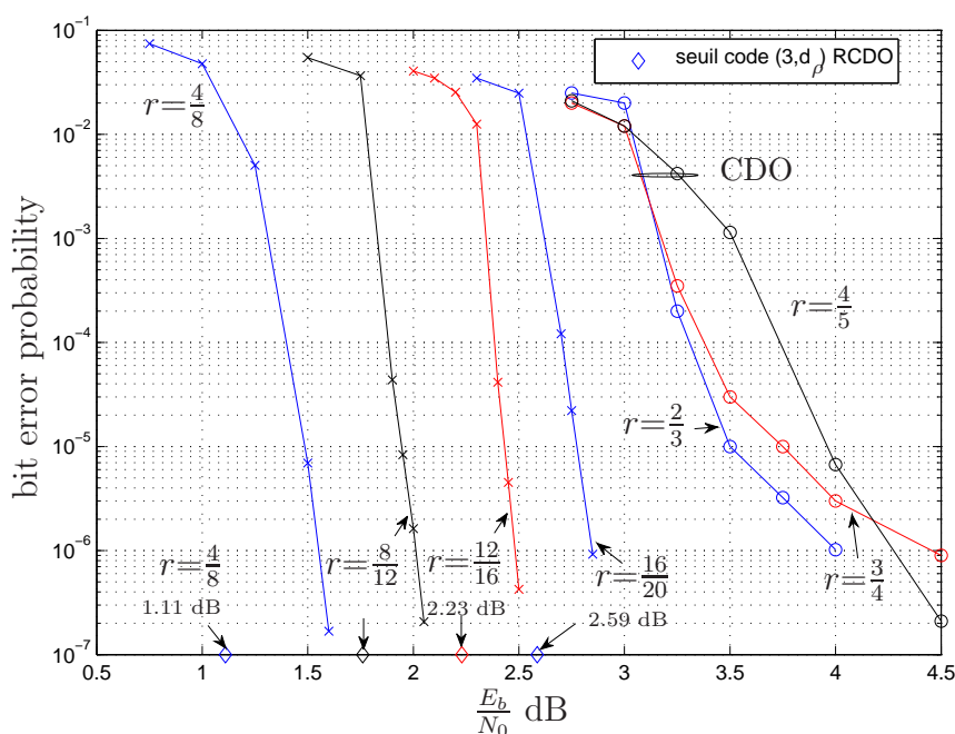
FIGURE 6.6 Performances d'erreur des codes imbriqués RCDO au code mère RCDO régulier (3, 15) qui permet d'atteindre les taux de codage 4/8, 8/12, 12/16 , et 16/20 à la suite de 25 itérations, m_s = 700 . Aussi reproduit, les performances d'un code multi taux de codage CDO avec m_s = 74451 .
