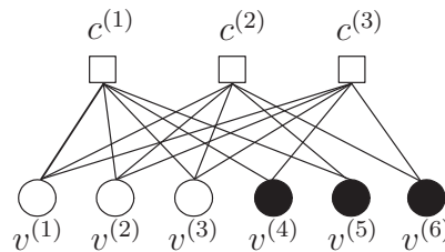
FIGURE 3.7 Protographe irrégulier représentant le code convolutionnel récurrent de taux de codage r = 3/6 de la Figure 3.6.
