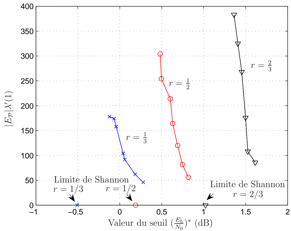
FIGURE 5.7 Nombre d'additions |E_{\mathcal{P}}|\lambda'(1) requises par itération en fonction du seuil associé aux paires de distributions (\lambda, \rho) des Tableaux 5.6, 5.7 et 5.8.
