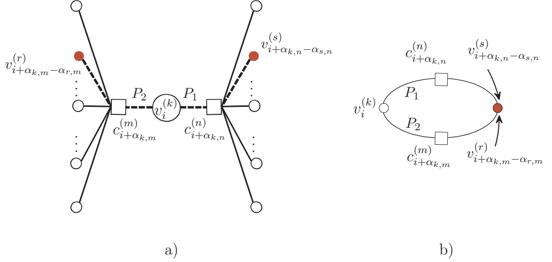
FIGURE A.1 a) Sous-graphe induit par les équations (A.1) et (A.2) dans le graphe de Tanner d'un code convolutionnel récursif simplement orthogonal. b) Cycle de longueur 4.
