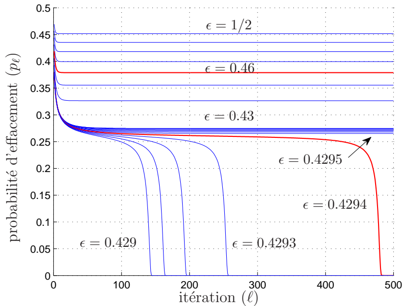
FIGURE 5.2 Évolution de la probabilité d’effacement p_\ell en fonction du nombre d’itérations \ell effectuées par le décodeur itératif.
