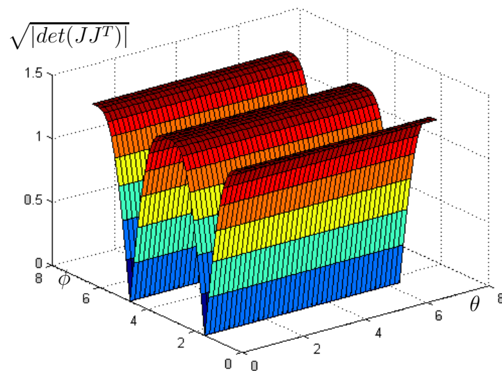
Figure I.2 Manipulabilité du manipulateur M'_1
