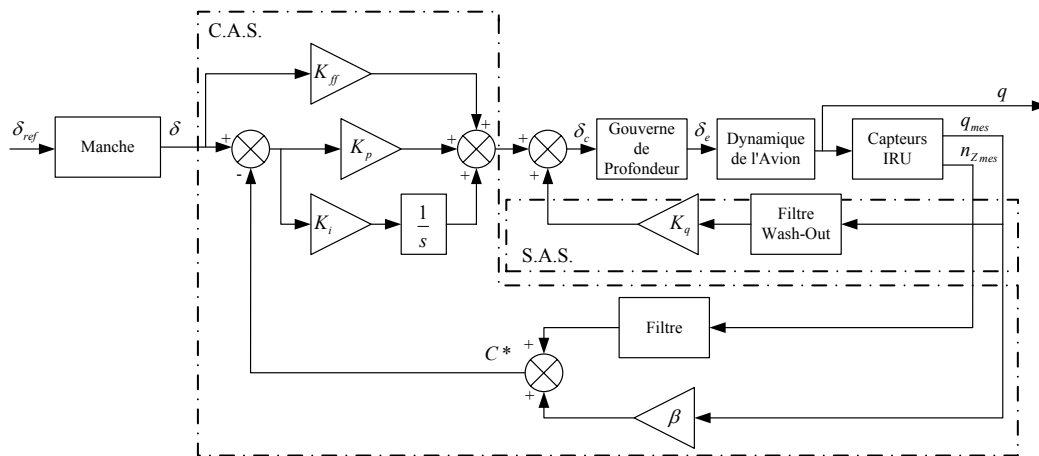
Figure 2.8 Contrôle C^*
