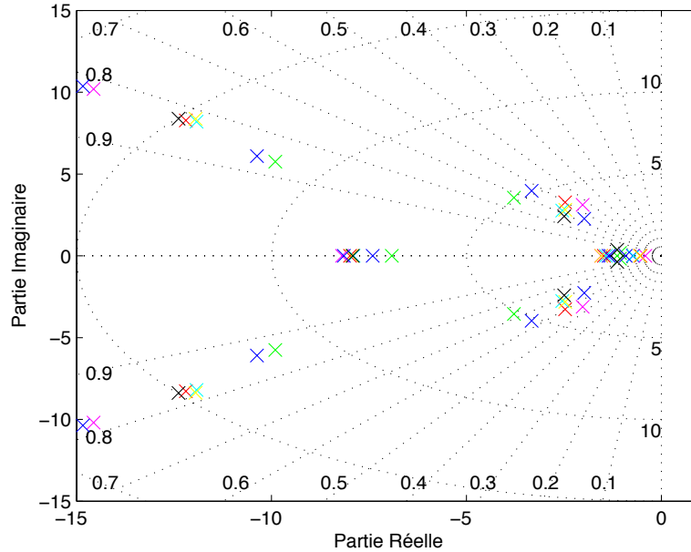
Figure 7.18 Pôles en boucle fermée pour les 8 configurations avec le correcteur réduit 3
