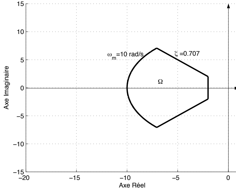
Figure 4.4 Domaine \Omega à garder
