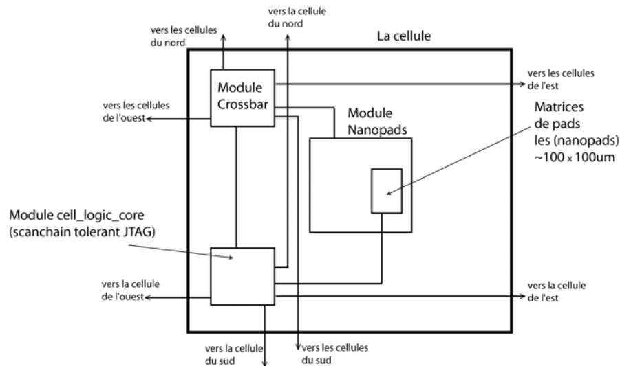
4-3 Architecture interne de la cellule.
