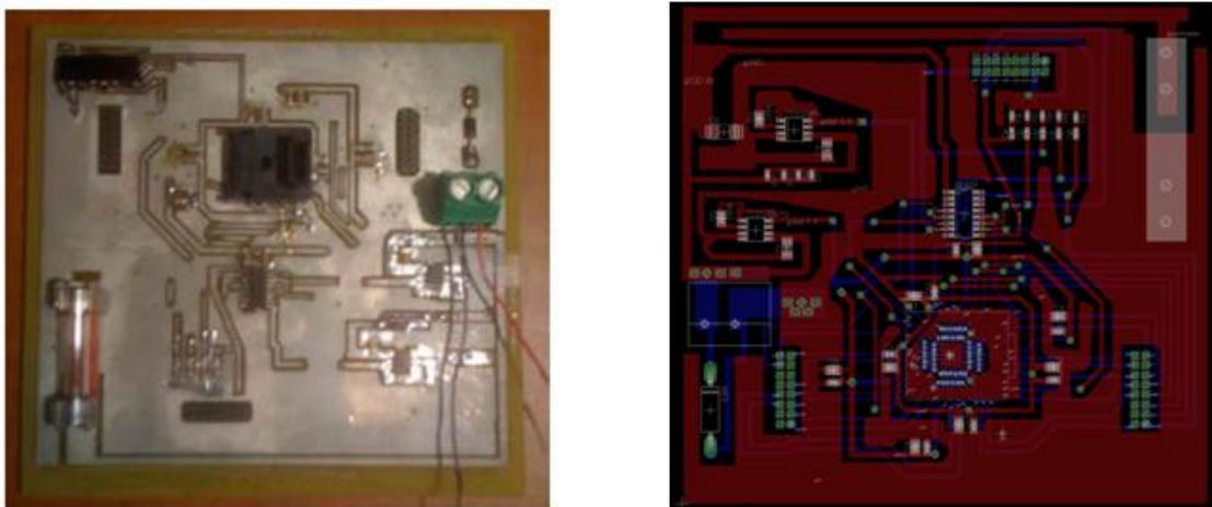
5-2 Vue XY du PCB fabriqué (gauche) et du dessin (droite)
