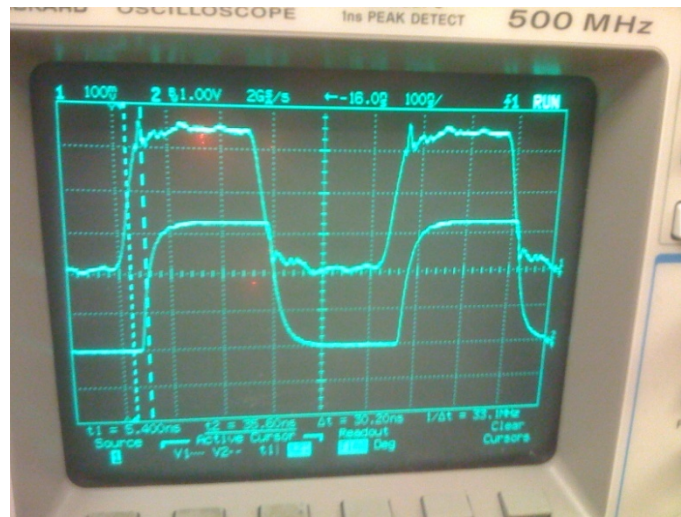
5-3 Propagation du signal dans le WaferNet du TestChip V1.0
