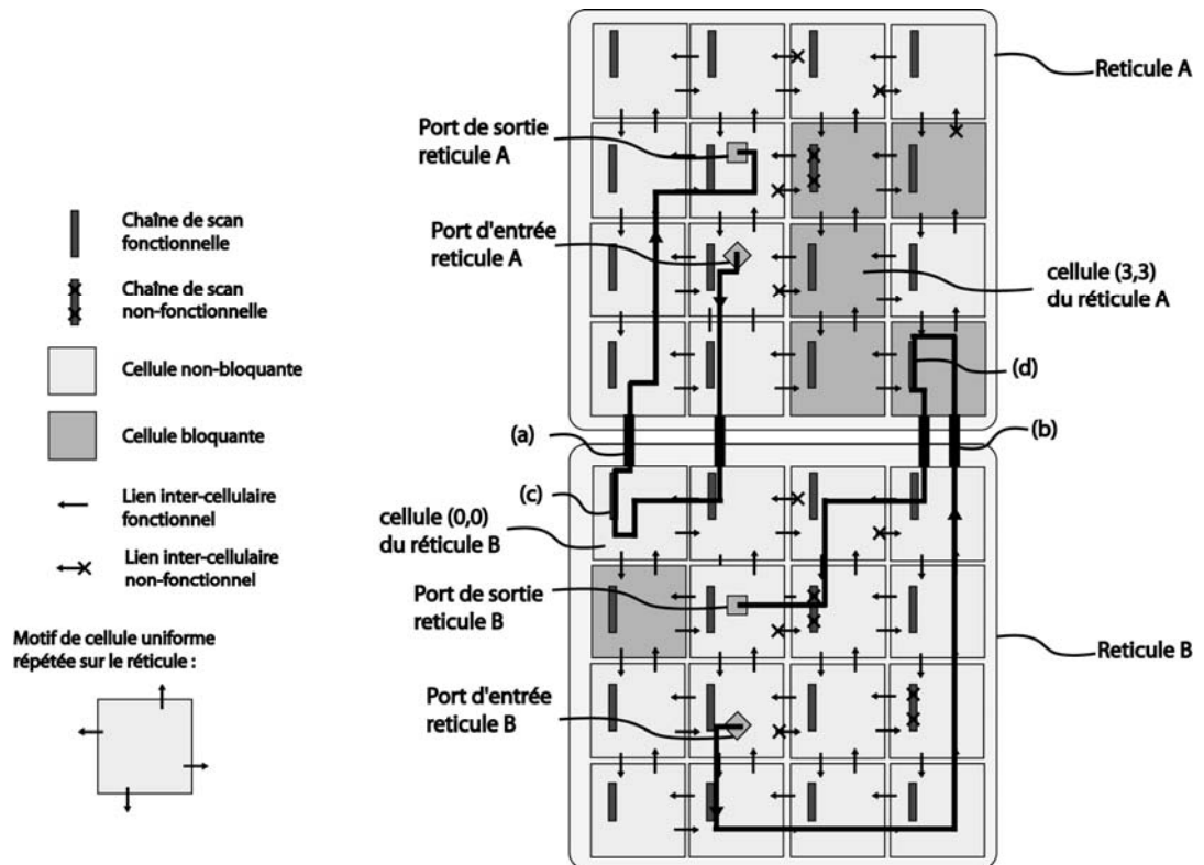
2-7 Exemple de communication sérielle entre deux réseaux voisins
