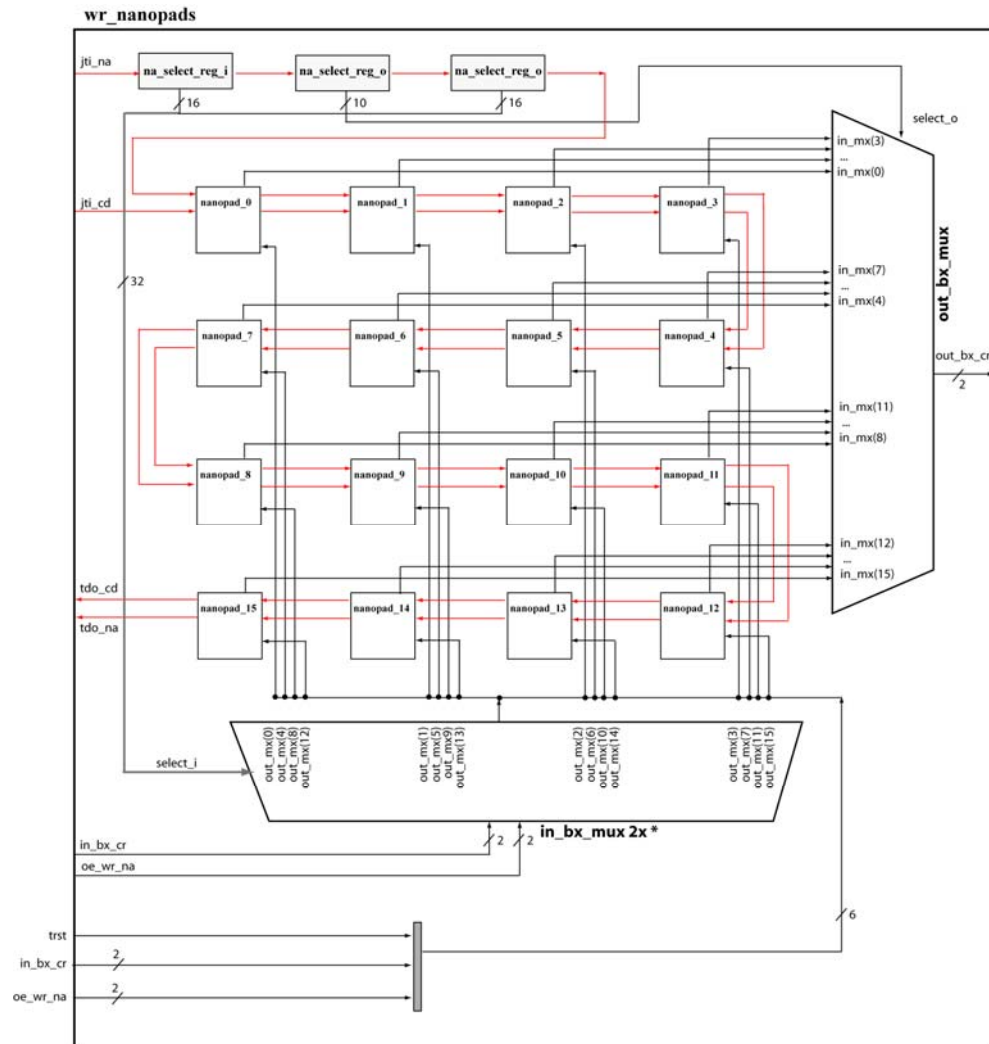
Figure D.2 Description structurale détaillée (VHDL) de l'entité wr_nanopads
