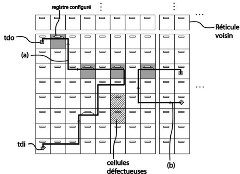
3-8 Les capacités de la chaîne reconfigurable pour le diagnostic.
