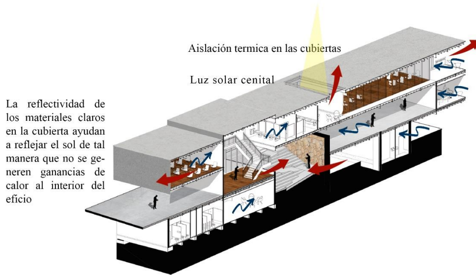
Ilustración 7 Corte detalle longitudinal Fuente: Elaboración propia, año 2018
