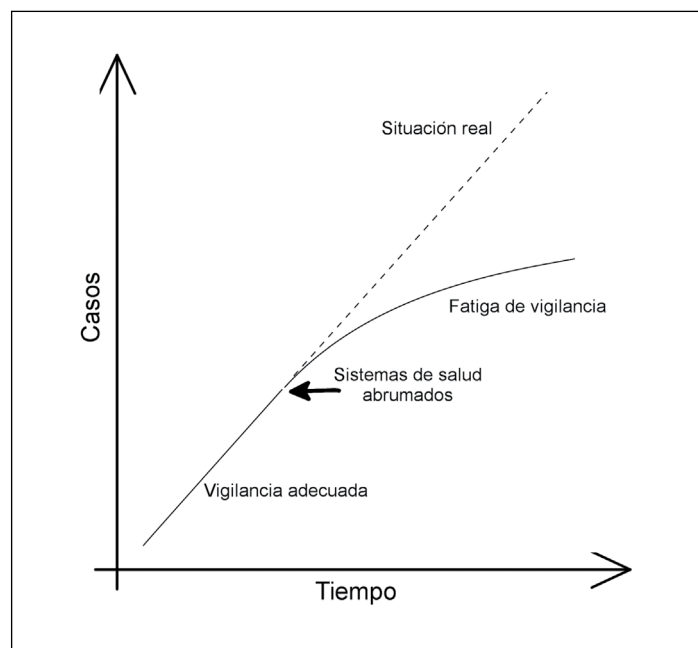
Figura 1. Ejemplo de fatiga de vigilancia. El número acumulado de casos reportados en la etapa inicial de una epidemia puede reflejar el número de casos correctamente (línea recta continua). A medida que el tiempo pasa, la eficacia de la notificación de casos disminuye debido, por ejemplo, a la escasez de personal o suministros de laboratorio y al elevado número de pacientes que abruma los sistemas de salud (flecha). Esto puede resultar en un número incompleto de casos reportados (línea de curva continua), que no refleja el número real de casos (línea discontinua).
