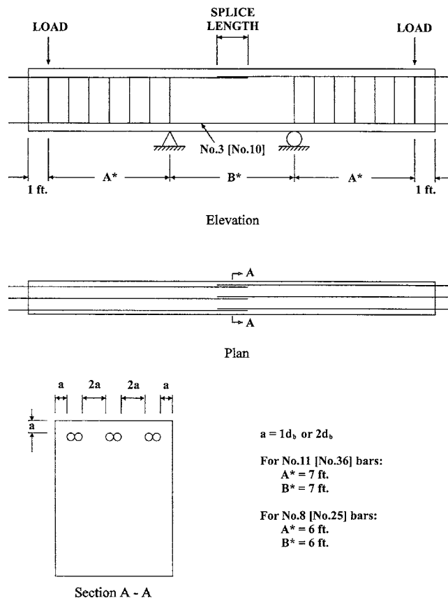
Fig. 1—Test specimen.
