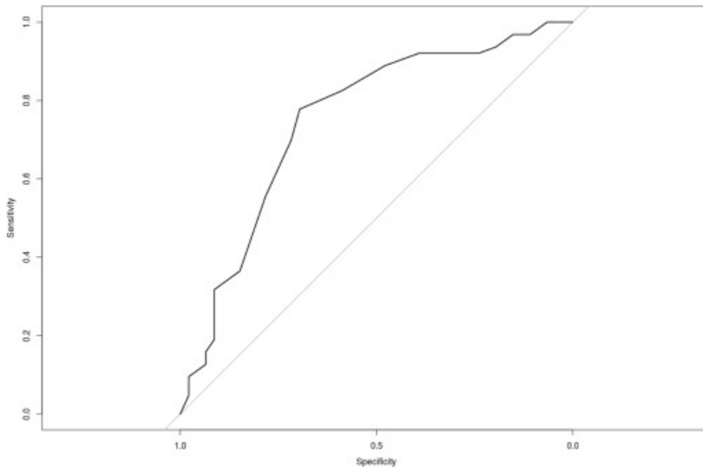
Fig. 1. ROC analysis.
