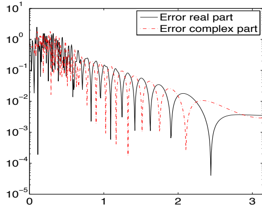
(d) Relative errors for k = 8
