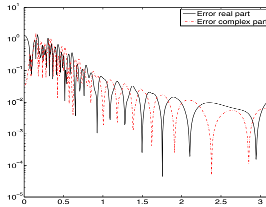
(d) Relative errors for k = 6
