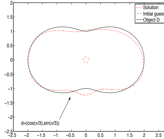
(d) Spline, k = 1 , d = (\sqrt{3}/2, 1/2) , N_r^2 = 12
