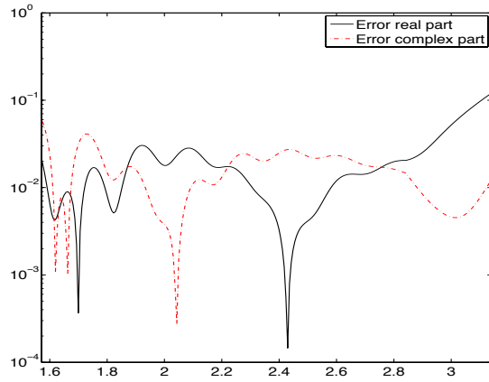
(d) Relative errors for k = 7
