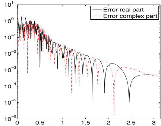
(d) Relative errors for k = 8
