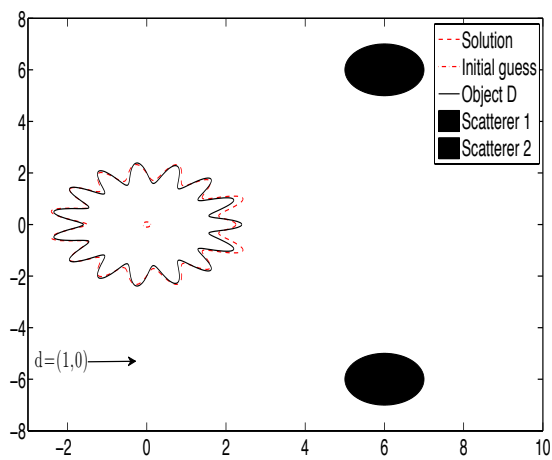
(d) k_j = 0.5j , N_r = 17 , N_{\text{inc}} = 12 , d = (1, 0)
