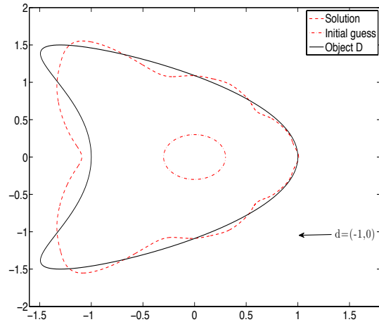
(e) Trigonometric, k = 1 , d = (-1, 0) , N_r^1 = 20
