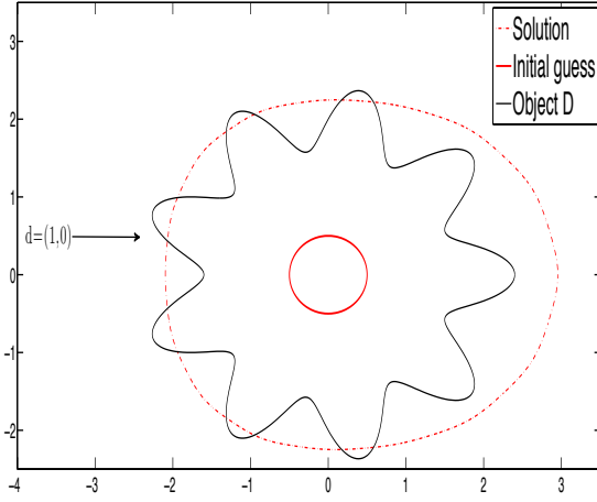
(d) k = 0.5 , N_r = 32 , d = (1, 0)
