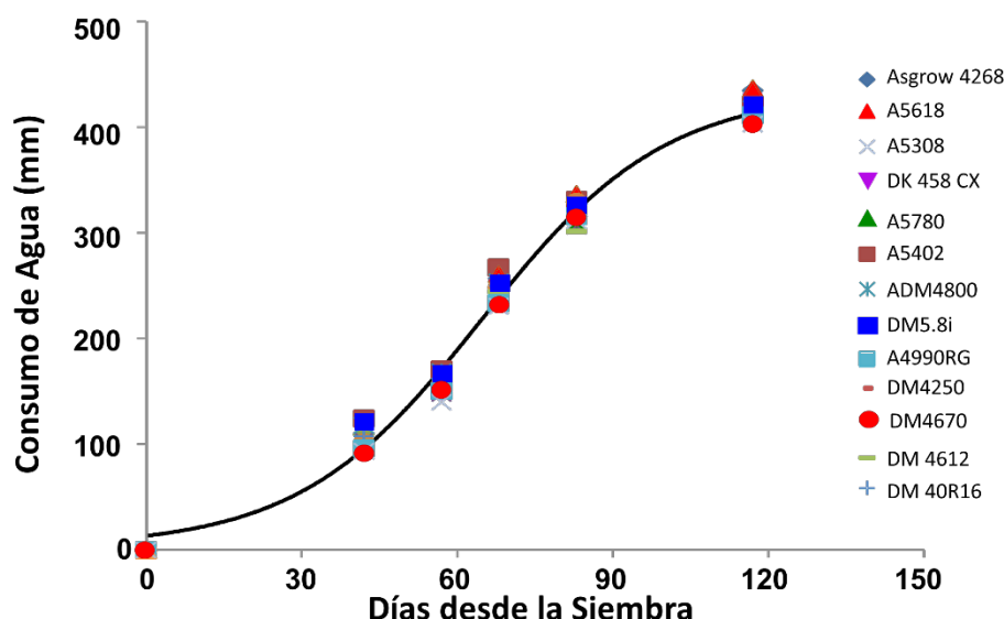
Figura 3. Evolución del consumo de agua ( ET_c : Evapotranspiración del cultivo) desde la siembra a R7, medido en 13 variedades de soja en Pergamino. La línea representa el modelo sigmoide ( ETC = a/(1-\exp(-b \times (X-c))) ) ajustado al conjunto de todas las variedades ( r^2 = 0,99 ; p < 0,001 ).
