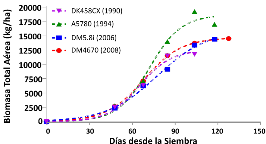
Figura 2. Evolución de la biomasa total aérea (BT) de cuatro variedades de soja. Los datos corresponden a las dos de menor (DK458CX-1990 y DM5.8i-2006) y mayor (A5780-1994 y DM4670-2008) rendimiento en grano a través de las localidades evaluadas (Tabla 1). Las líneas punteadas corresponden a los modelos sigmoideos ( BT = a/(1-\exp(-b \times (X-c))) ) ajustados ( r^2 \geq 0,983 ; p \leq 0,006 ).
