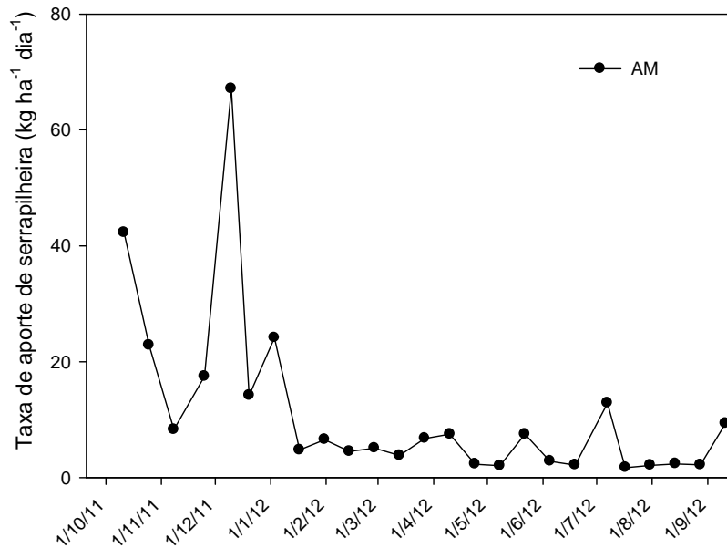
Fig. 4. Aporte de sarrapilheira em Cambissolo Háplico no período de um ano. Vila Nova do Sul, 2012. AM: Acácia.
