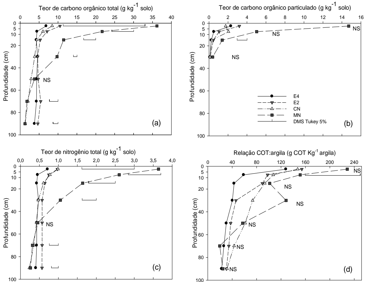
Fig. 5. Teor de COT (a), de COP (b) e de NT (c) e relação COT:argila (d) no solo em um Argissolo Vermelho-Amarelo nos diferentes usos do solo. Cacequi (2012). E4: eucalipto com 4 anos de cultivo; E2: eucalipto com 2 anos de cultivo; CN: campo nativo (área de referência); MN: mata nativa. As barras horizontais indicam a diferença mínima significativa pelo teste de Tukey ( P < 0,05 ) entre os tratamentos avaliados dentro da respectiva camada de solo. NS: diferença não significativa.
