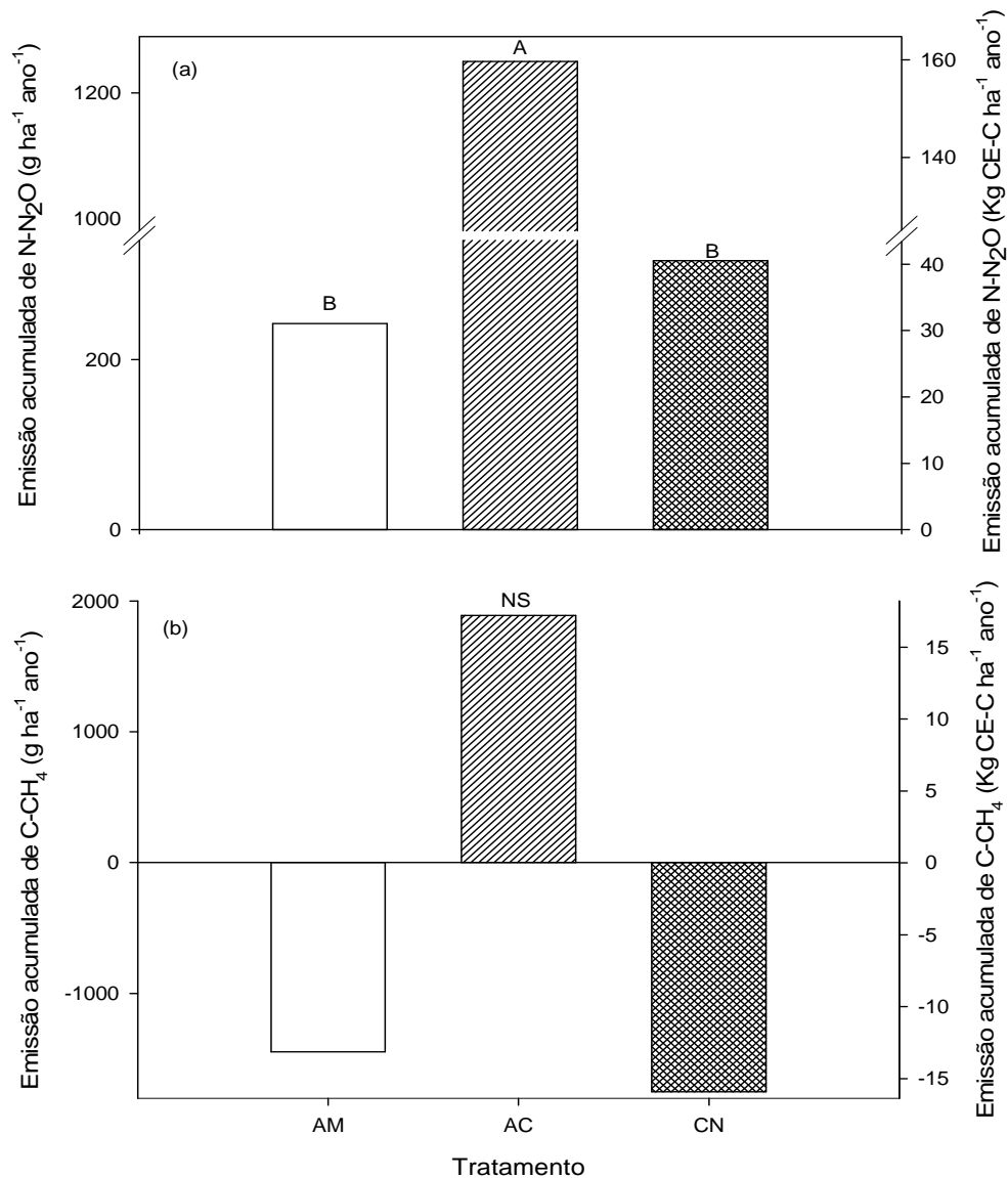
Fig. 5. Emissão acumulada de N-N 2 O (a) e C-CH 4 (b) em Cambissolo Háplico sob diferentes usos do solo no período de um ano. Vila Nova do Sul, 2012. AM: Acácia; AC: Acácia colhida; CN: campo nativo (área de referência); A, B: teste de Tukey ( P < 0,05 ); NS: diferença não significativa entre os tratamentos avaliados.
