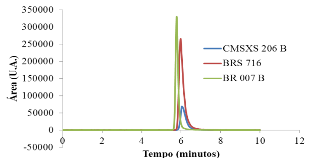
Figura 2: Cromatograma de sorgoleone dos genótipos testados.
