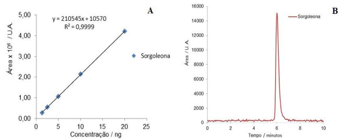
Figura 1: Curva de calibração (A) e cromatograma da sorgoleone na concentração de 1,3 ng (B).
