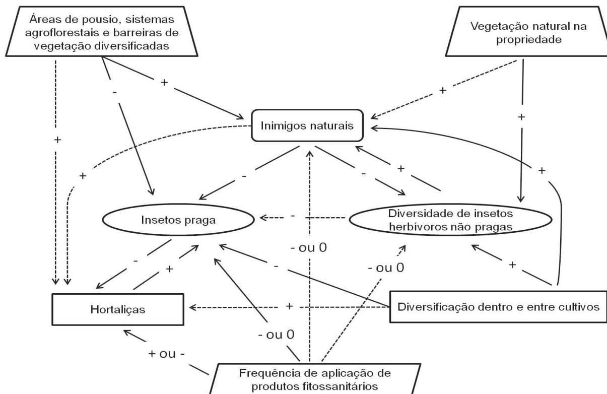
Figura 1 – Interações ecológicas entre práticas culturais, manejo da propriedade agrícola, insetos praga, insetos herbívoros não pragas e inimigos naturais em hortaliças orgânicas. As linhas sólidas indicam interações diretas e as linhas tracejadas interações indiretas de natureza positiva (+), negativa (-) ou neutras (0).
