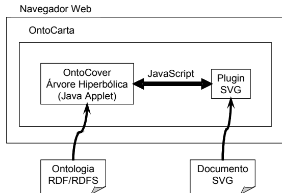
Figura 6 – Arquitetura Geral do OntoCarta
