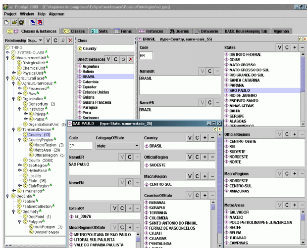
Figura 1- A ontologia agrícola no Protégé 2000
