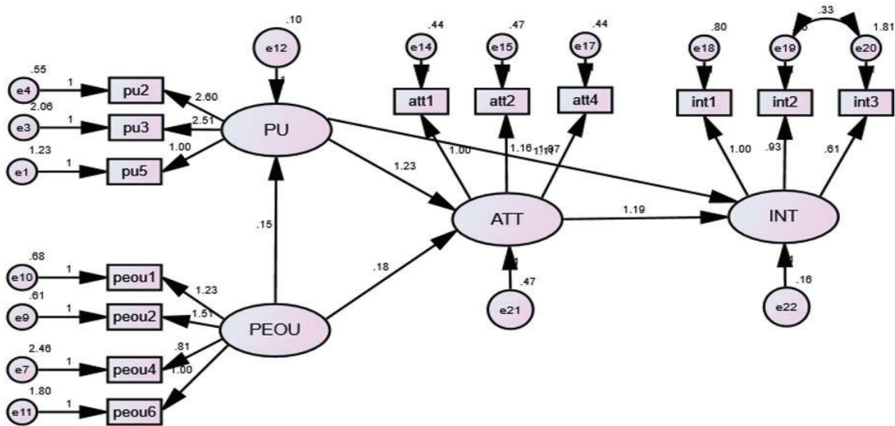
Figure 2. Path diagram Abbildung 2. Pfaddiagramm
