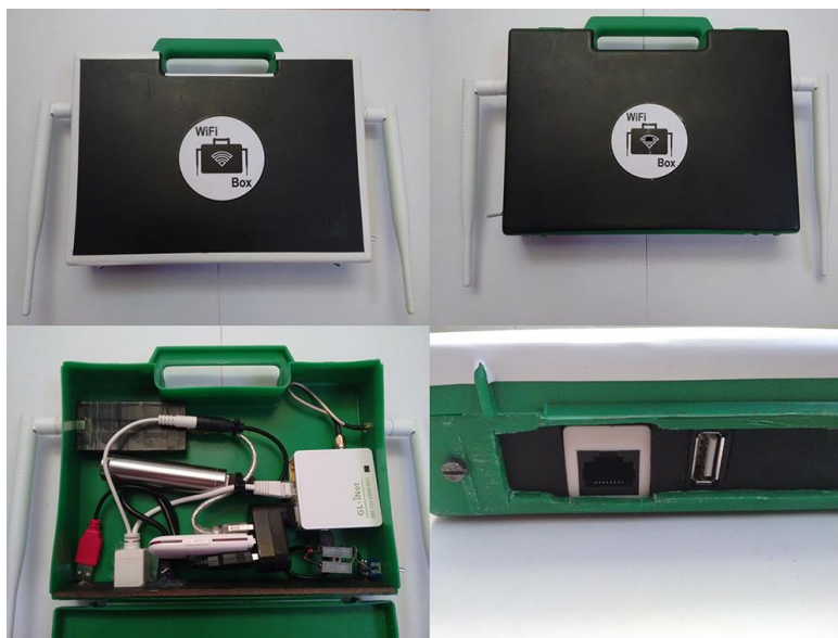
Slika 6. Uređaj WiFiBox.
