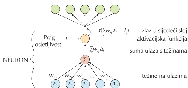
Slika 2 – Prikaz perceptrona
