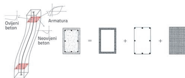
Slika 1. Tipični model vlakana AB elementa [17]
