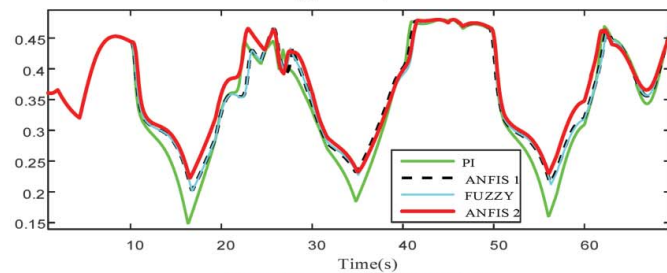
(d) Power conversion coefficients
