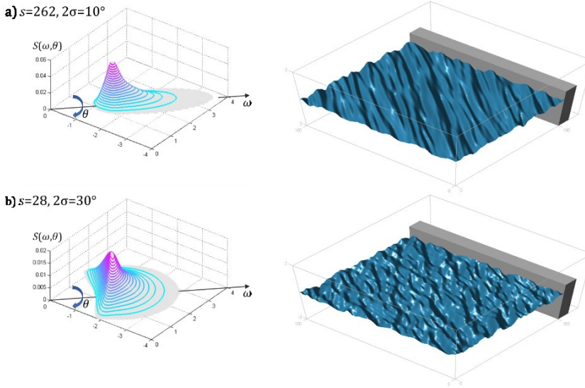
Slika 7. Dvodimenzijски спектар valova i sintetički generirana površina mora za H_s = 0,5 m i dva različita s faktora, koji odgovaraju rasponu kutova \pm 10^\circ i \pm 30^\circ oko glavnog smjera napredovanja \theta_0=45^\circ
