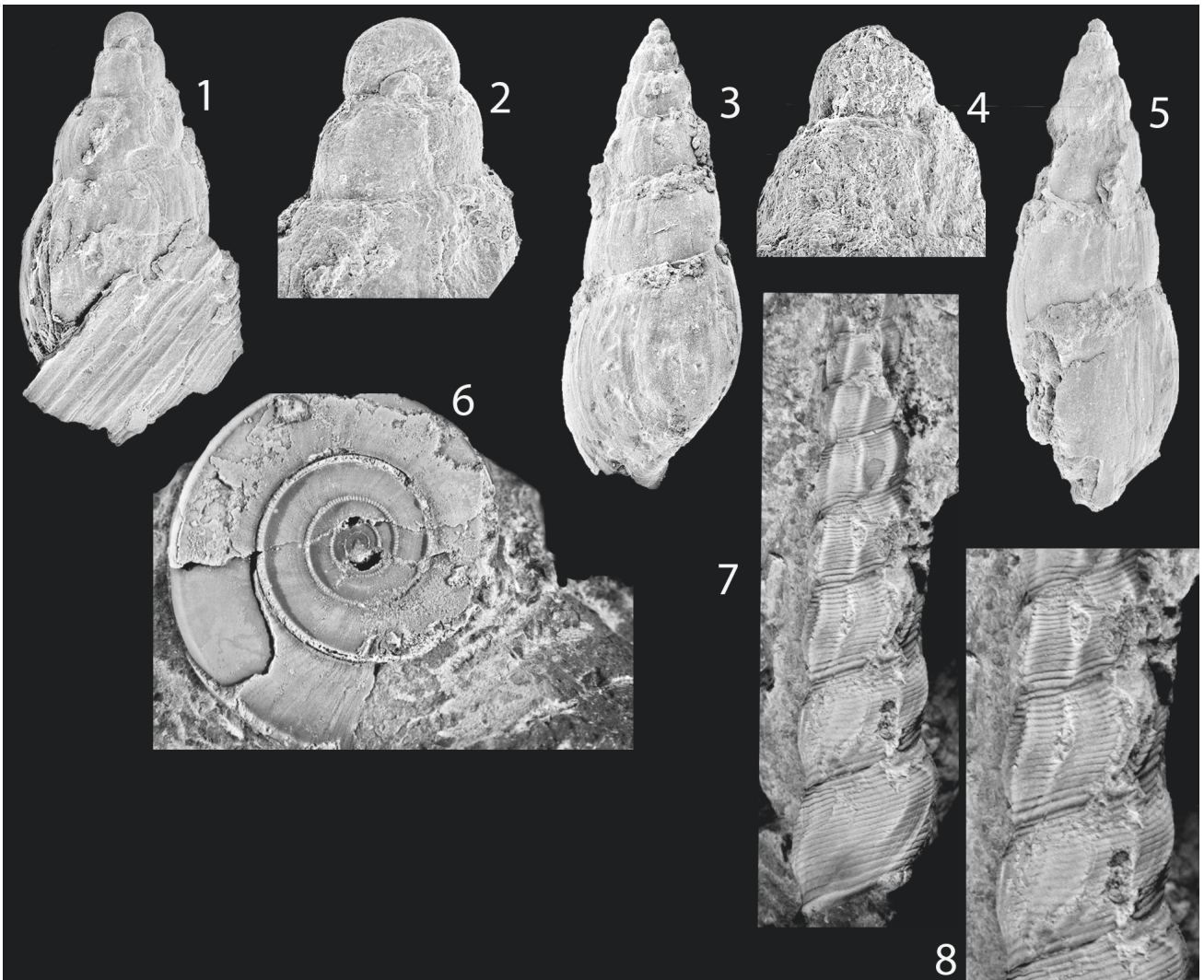
Tafel 8: (1, 2) Cossmannina kalchreuthensis (Gründel & Nützel, 1998), Dörlbach (JME – 2015/60), 1: Gehäuse in Seitenansicht, Breite 1,3 mm, 2: Gehäusespitze in Seitenansicht, Durchmesser des Protoconchs 0,34 mm. (3–5) Cossmannina? franconica (Kuhn, 1935, Dörlbach (JME – 2015/61), 3, 5: Gehäuse in zwei Seitenansichten, Höhe 7,1 mm, 4: Gehäusespitze in Seitenansicht, Durchmesser des Protoconchs 0,27 mm. (6) Discohelix calculiformis schlosseri Kuhn, 1936, Bauaushub Stauf (SMNS 67900), Gehäuse in Seitenansicht, Breite 23 mm (Kopie von Gründel 2011: Taf. 1, Fig. 1), (7, 8) Pseudokatosira? sp. 1 , Bauaushub Stauf (SMNS 67801), 7: Gehäuse in Seitenansicht, Höhe 19,5 mm, 8: Detail der Seitenansicht, Höhe 10 mm (Kopie von Gründel 2011: Taf. 1, Fig. 5, 6).
