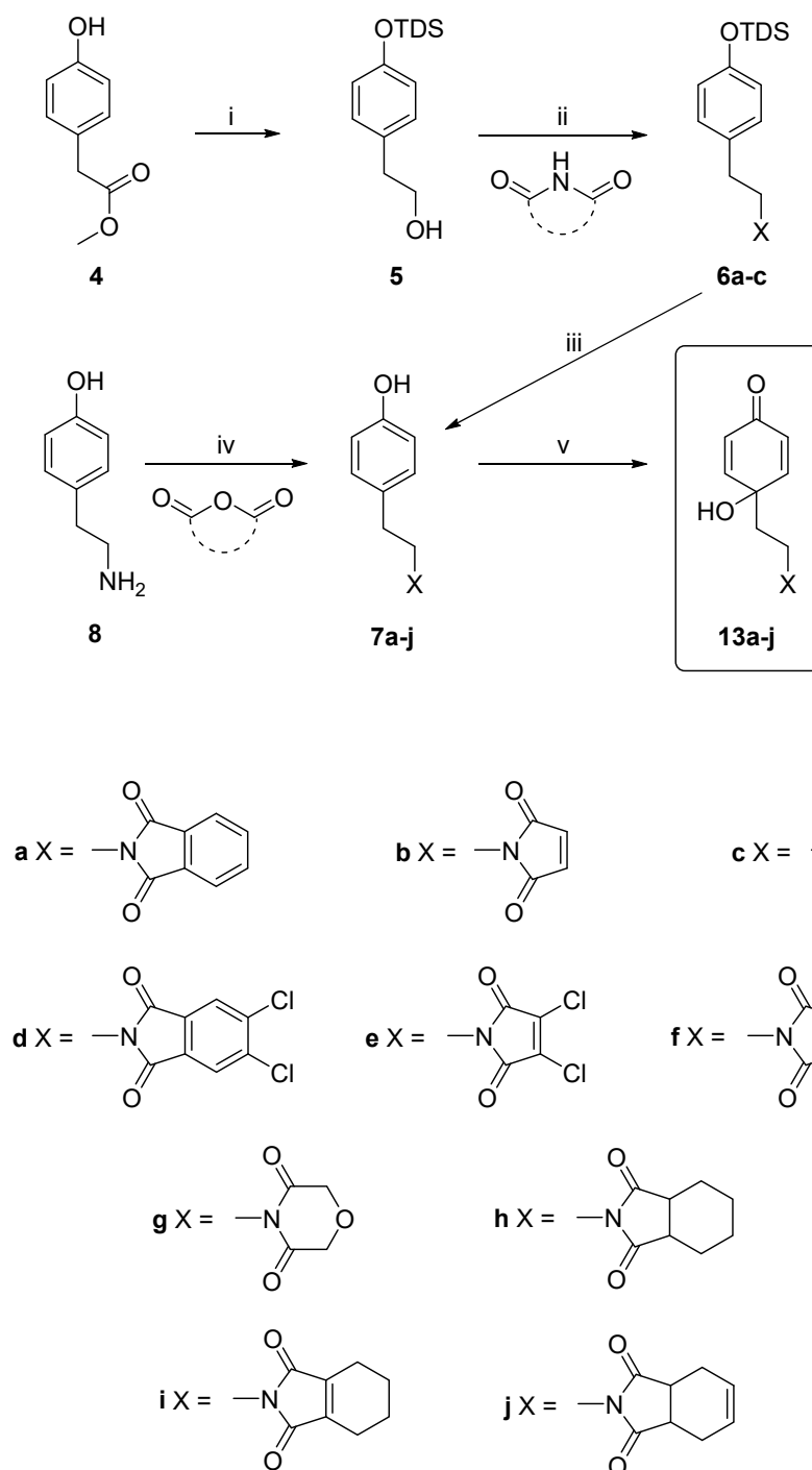
Scheme 1. Reagents and conditions: method A: (i) 1. TDSCl, DBU, RT, 1.5 h; 2. \text{LiAlH}_4 , THF, 0 °C, 2 h (98%); (ii) imide, \text{PPh}_3 , DIAD, THF, 0 °C→RT, 2.5–24 h ( 6a : 90%, 6b : 70%, 6c : 77%); (iii) TBAF, \text{CH}_2\text{Cl}_2 , RT, 1 h ( 7a : 80%, 7b : 85%, 7c : 82%); (iv) anhydride, AcOH, 120 °C, 1.5 h (method B: 7a : 73%, 7b : 55%, 7c : 58%, 7d : 89%, 7e : 90%, 7f : 0%, 7g : 0%, 7h : 86%, 7i : 92%, 7j : 79%) or PEG 400, 140 °C, 4 h (method C: 7a : 23%, 7b : 51%, 7c : 98%, 7d : 67%, 7e : 67%, 7f : 86%, 7g : 71%, 7h : 79%, 7i : 98%, 7j : 98%); (v) \text{PhI}(\text{OAc})_2 , \text{CH}_3\text{CN}/\text{H}_2\text{O} (12:5), 0 °C, 7 min ( 13a : 67%, 13b : 17%, 13c : 55%, 13d : 40%, 13e : 64%, 13f : 19%, 13g : 18%, 13h : 79%, 13i : 88%, 13j : 49%).
