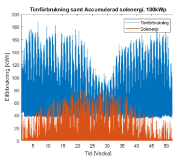
Figur 7: Timfördelning, 100kWp
