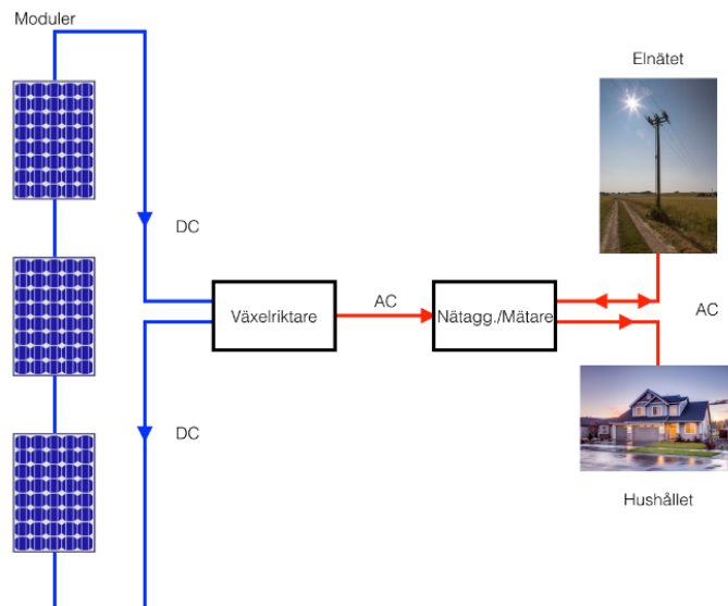
Figur 2. Schematisk bild över en nätansluten solcellsanläggning.
