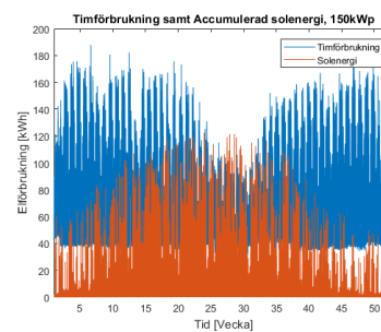
Figur 8: Timfördelning 150kWp
