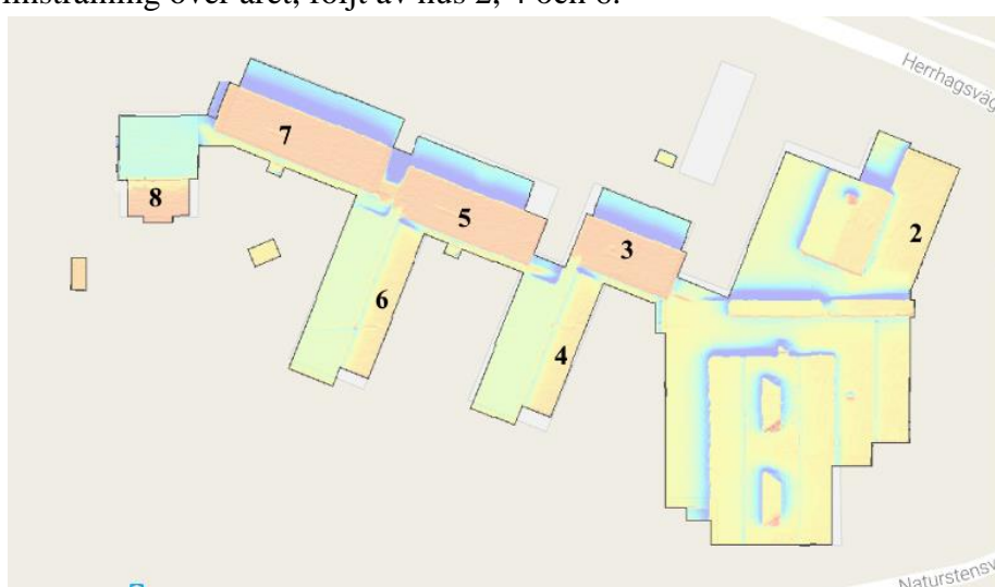
Figur 5: Karta över instrålad effekt på samtliga tak på SBKC där röd färg indikerar högst solinstrålning (Uppsala Kommun 2015).
