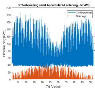
Figur 6: Timfördelning, 50kWp
