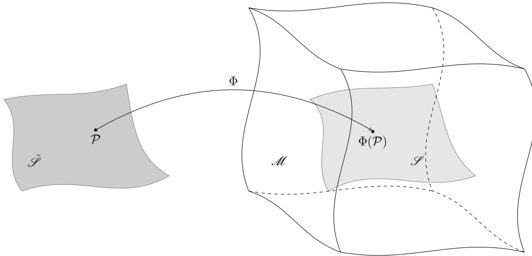
Figura 2.2.1: Rappresentazione dell'immersione \Phi di una varietà 3-dimensionale \tilde{\mathcal{S}} in una varietà 4-dimensionale \mathcal{M} che definisce l'ipersuperficie \mathcal{S} .
