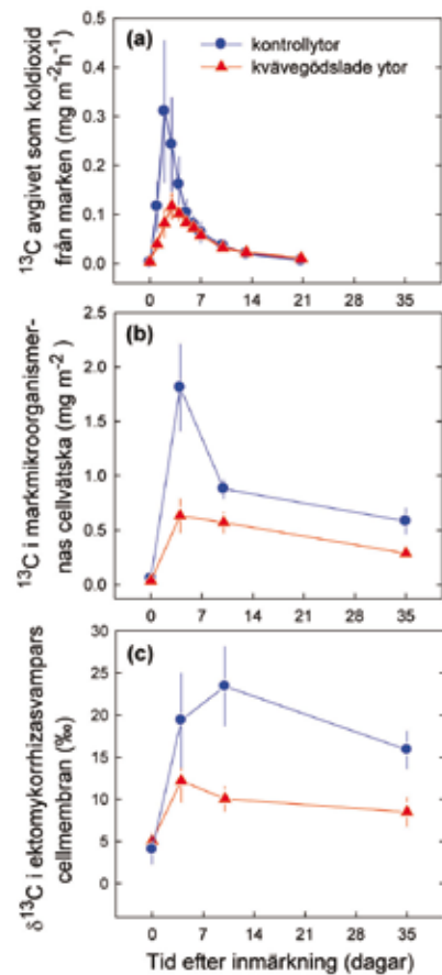
FIGUR 3. Allokeringen av kol ( ^{13}C ) från trädens kronor till organismer i marken på ogödslade kontrolltytor (blått) och på kvävegödslade tytor (rött) över tiden. Inmärkningsen med ^{13}C (se Figur 2) avslutades vid dag 0. Figur 3a visar hur märkt kol respireras och avgår från marken, 3b visar hur abundansen av märkt kol i markmikroorganismernas cellvätska ändras, och 3c visar abundansen av märkt kol i en fettsyra ( \delta^{13}C beskriver avvikelser i kvoten ^{13}C/^{12}C relativt Vienna Pee Dee Belemnite-standard uttryckt i promille (Högberg, M.N. et al. 2010)) som är typisk för ektomykorrhizasvamparnas cellmembran.
