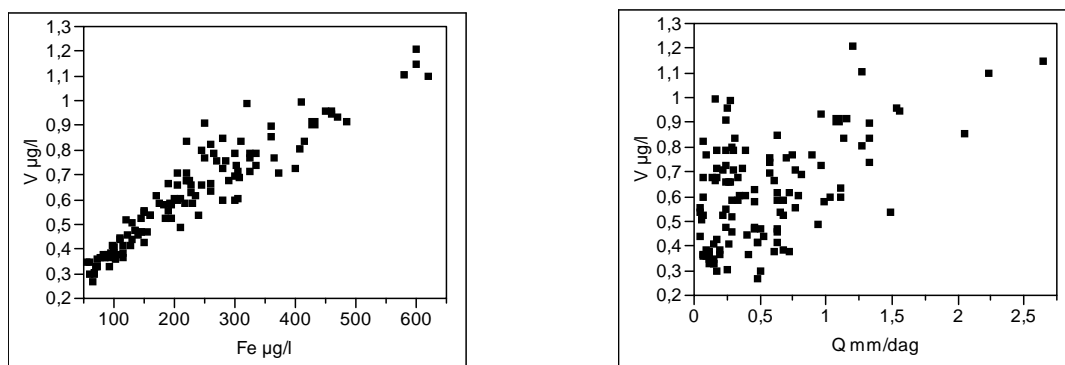
Figur 100. Samband mellan V och Fe ( r^2=0,87 , p<0,0001 ) respektive flödet ( r^2=0,42 , p<0,0001 ) i Nyköpingsån under perioden 1998-2007 ( N=117 ).
