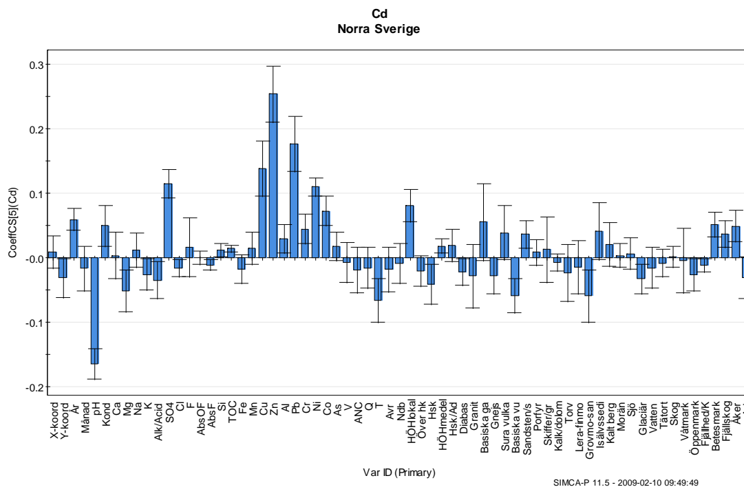
Figur 41. Korrelationskoefficienter mellan Cd och övriga variabler (centrerade och normaliserade), norra Sverige, 39 vattendrag. Modellen har 5 signifikanta komponenter ( R2X = 0,507 ; R2Y = 0,637 ; Q2(\text{cum}) = 0,626 ).
