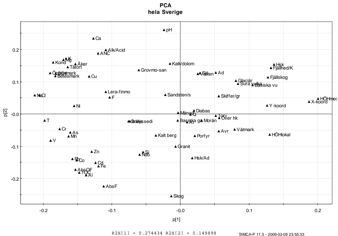
Figur 26. PCA, Loading plot för hela datamaterialet, omfattande data från 80 vattendrag. Modellen har 9 signifikanta komponenter, ( R2X = 0,726 ; Q2(cum) = 0,549 )
