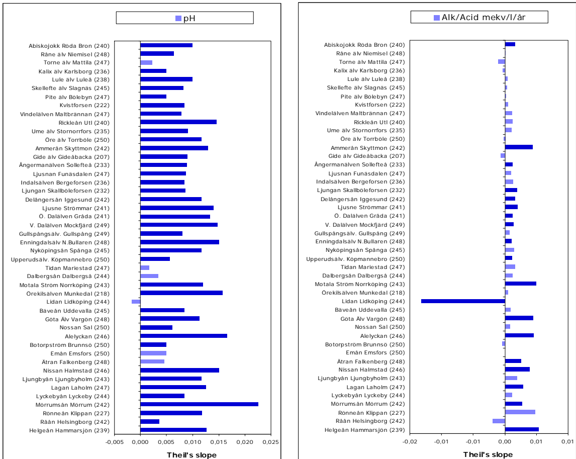
Figur 1. Trender i pH och alkalinitet i 46 vattendrag under perioden 1987-2007. Trenderna är beräknade med Theil's slope där statistiskt signifikanta trender ( p < 0,05 , Seasonal Kendall) visas med mörkblå staplar, medan icke statistiskt signifikanta trender visas med
