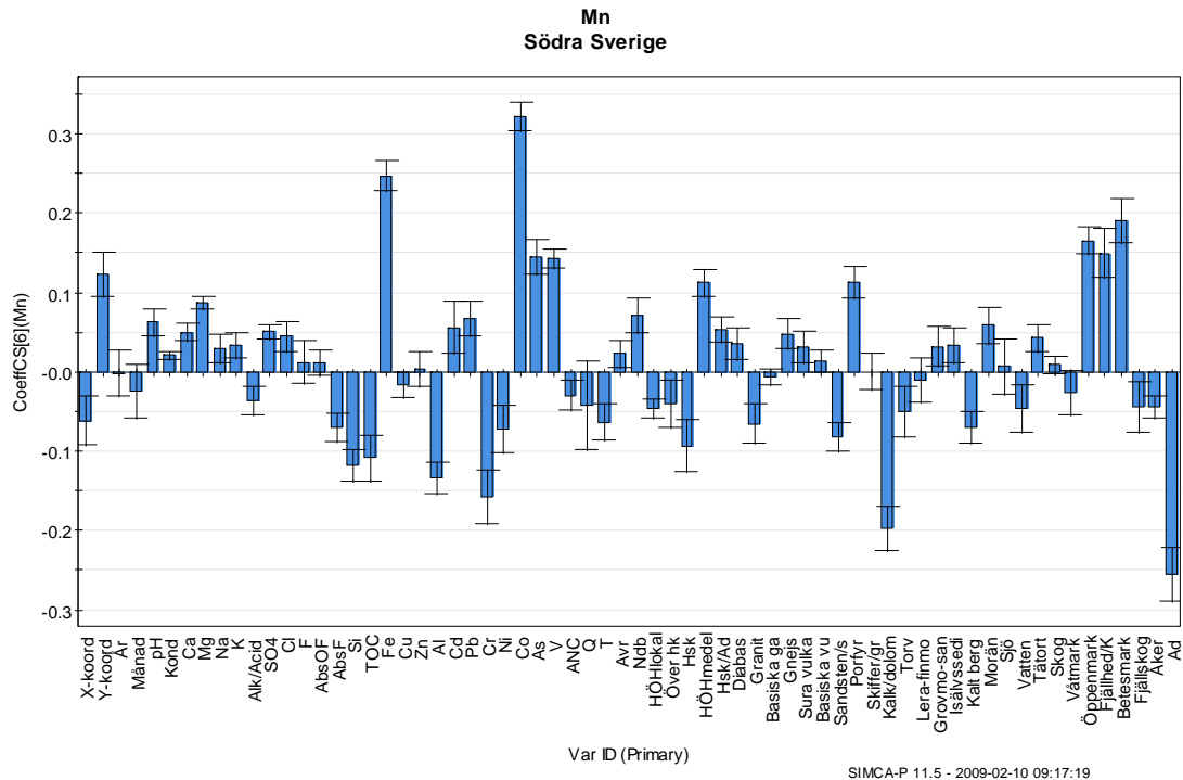
Figur 32. Korrelationskoefficienter mellan Mn och övriga variabler (centrerade och normaliserade), södra Sverige, 41 vattendrag. Modellen har 6 signifikanta komponenter ( R2X = 0,596 ; R2Y = 0,787 ; Q2(cum) = 0,784 ).
