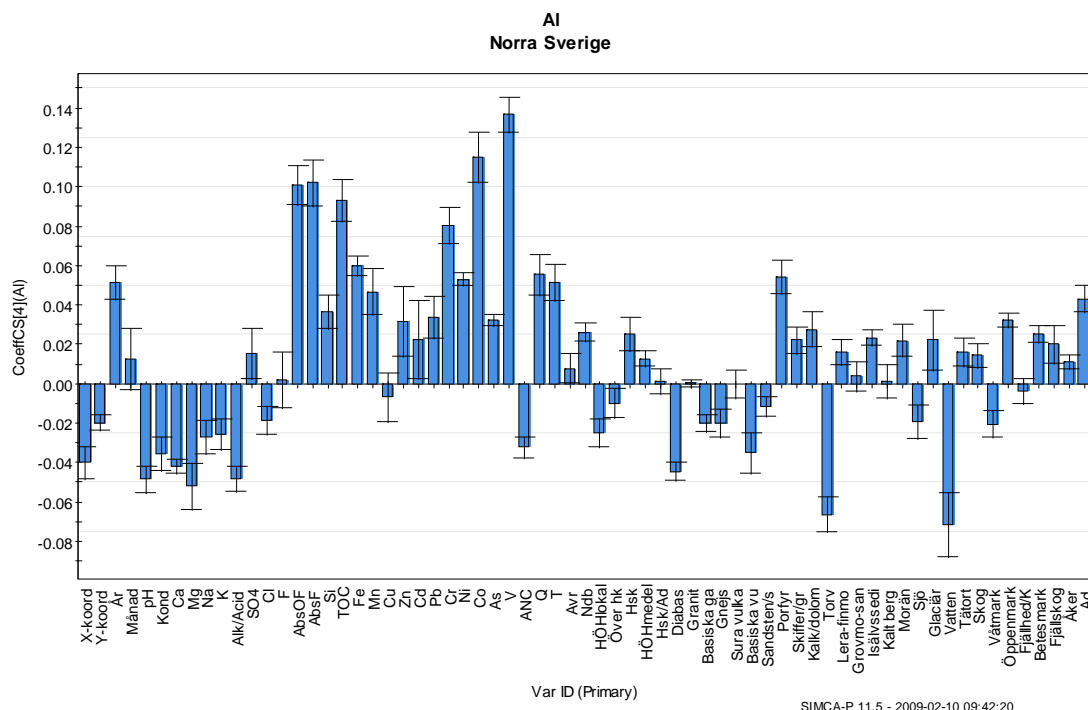
Figur 33. Korrelationskoefficienter mellan Al och övriga variabler (centrerade och normaliserade), norra Sverige, 39 vattendrag. Modellen har 4 signifikanta komponenter ( R2X = 0,464 ; R2Y = 0,905 ; Q2(cum) = 0,904 ).
