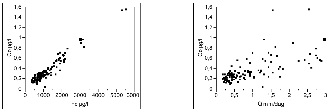
Figur 92. Samband mellan Co-koncentration och Fe ( r^2 = 0,93 , p<0,001 ) respektive flödet ( r^2=0,45 , p<0,001 ) i Tidan under perioden 1998-2007 (N=117).
