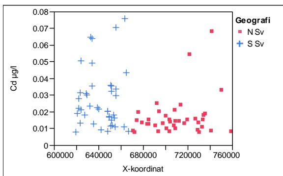
Figur 76. Koncentration av Cd i vattendrag i förhållande till vattendragens geografiska läge i norra respektive södra Sverige (medelvärden, N=79).
