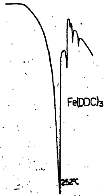
DTA (B)
