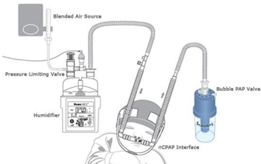
Figura 7: Partes de la CPAP Burbuja
