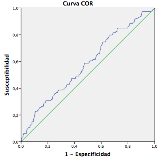
Figura 1.2: PCR
