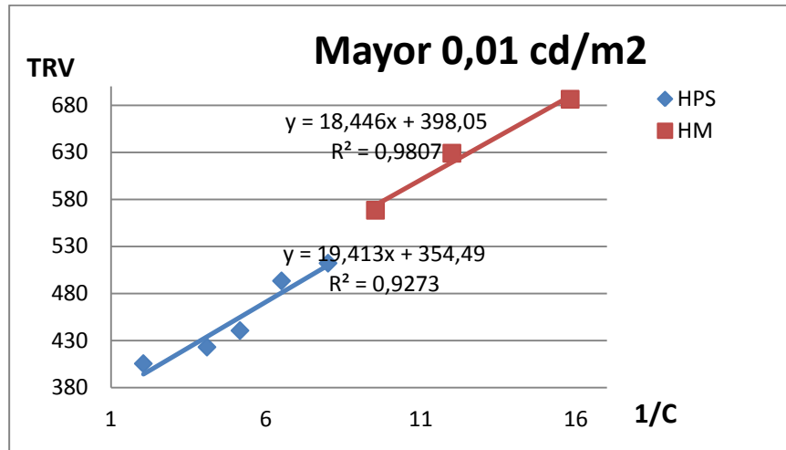
Figura 7. Tiempos de reacción para un sujeto de edad avanzada con una luminancia de 0.01 cd/m 2 .
