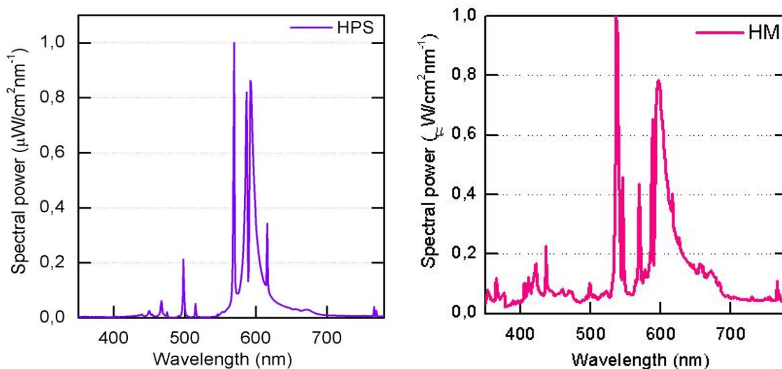
Figura 3. Espectros de las lámparas HPS y HM.
