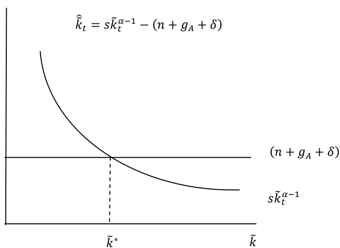
Figura 2.2: DINÁMICA DE TRANSICIÓN EN EL MODELO DE SOLOW
