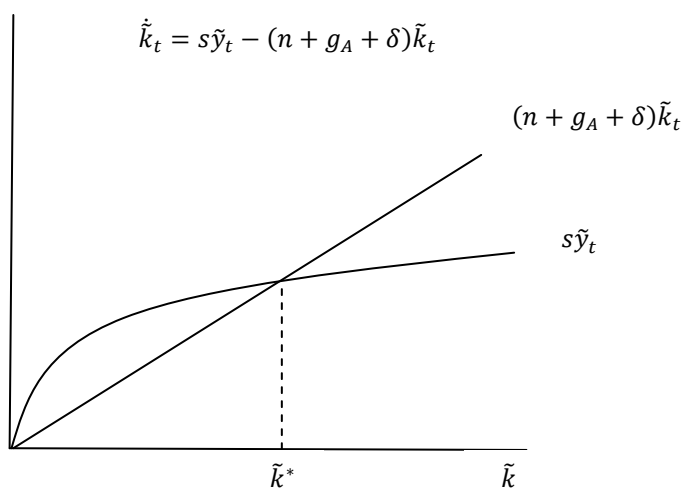
Figura 2.1: DIAGRAMA DE SOLOW CON PROGRESO TÉCNICO
