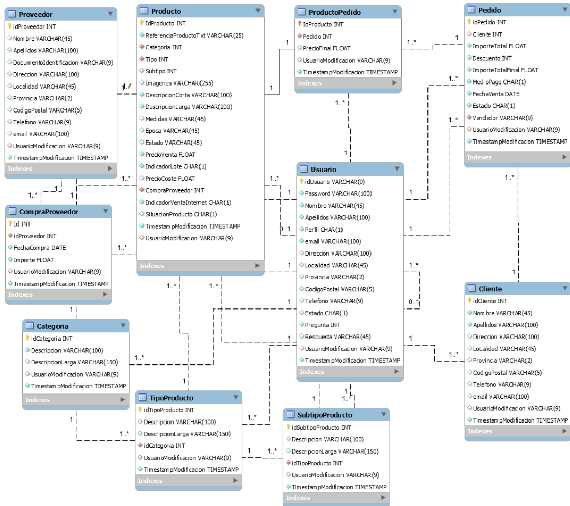
Imagen 10.2 - 3. Diagrama modelo relacional (completo).
