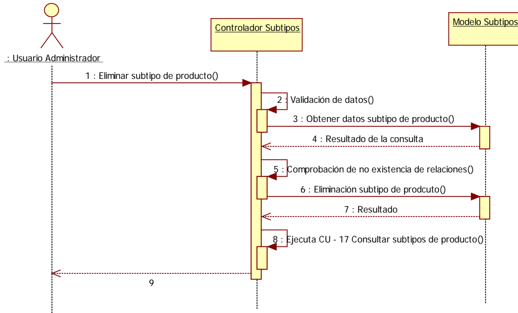
Imagen 9.5 - 25. Diagrama de secuencia CU – 21 Eliminar subtipo de producto.
