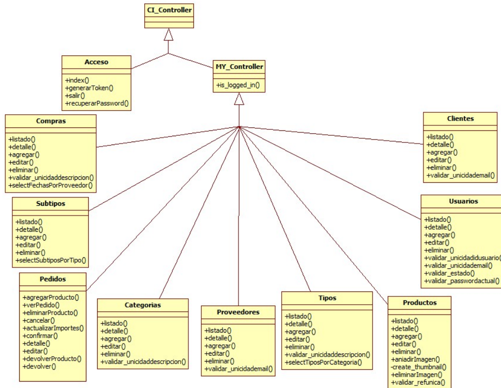
Imagen 10.1 - 1 Diagrama de clases de los controladores.
