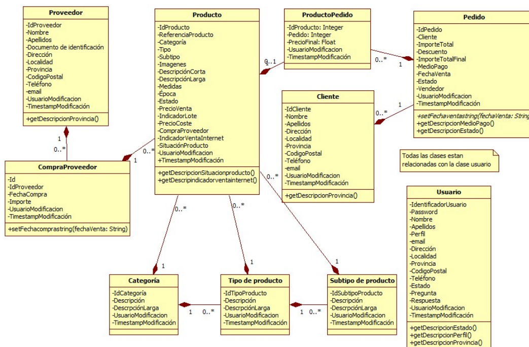
Imagen 10.1 - 3. Diagrama de clases de entidades.
