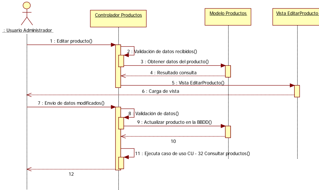
Imagen 9.5 - 41. Diagrama de secuencia CU - 34 Modificar producto.
