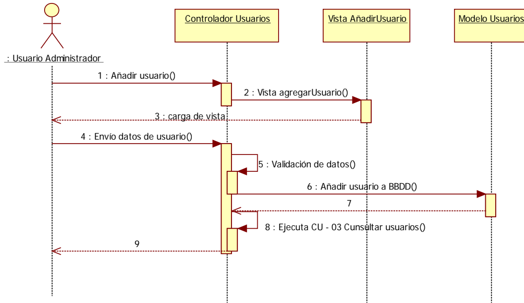
Imagen 9.5 - 3. Diagrama de secuencia CU - 02 Añadir usuario.
