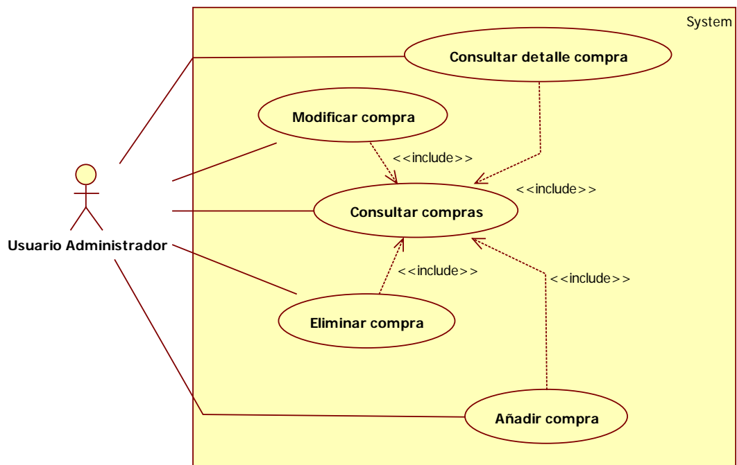
Imagen 9.5 - 32. Diagrama de casos de uso Compras a proveedores
