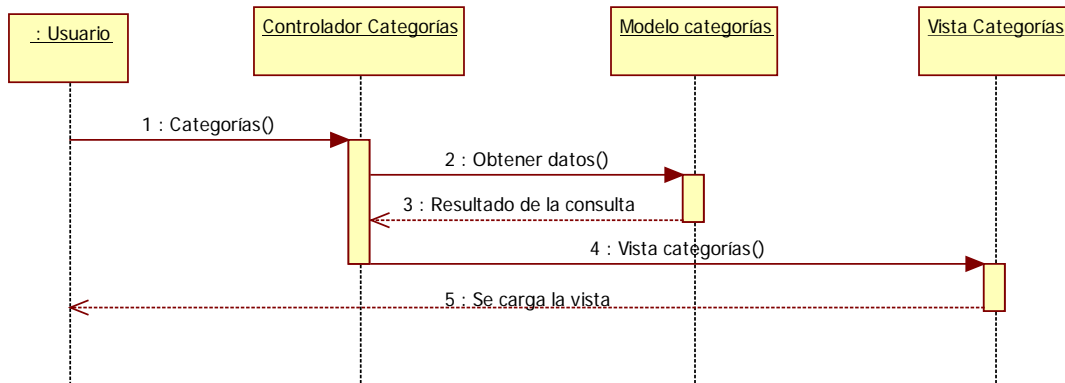
Imagen 9.5 - 10. Diagrama de secuencia CU - 07 Consultar categorías
