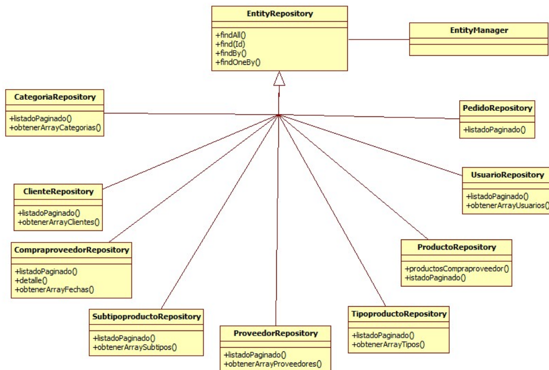
Imagen 10.1 - 2. Diagrama de clase de repositorios.
