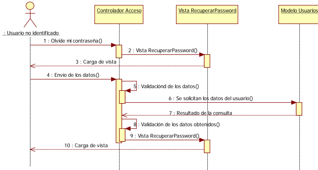
Imagen 9.5 - 8. Diagrama de secuencia CU – 52 Recuperar contraseña.
