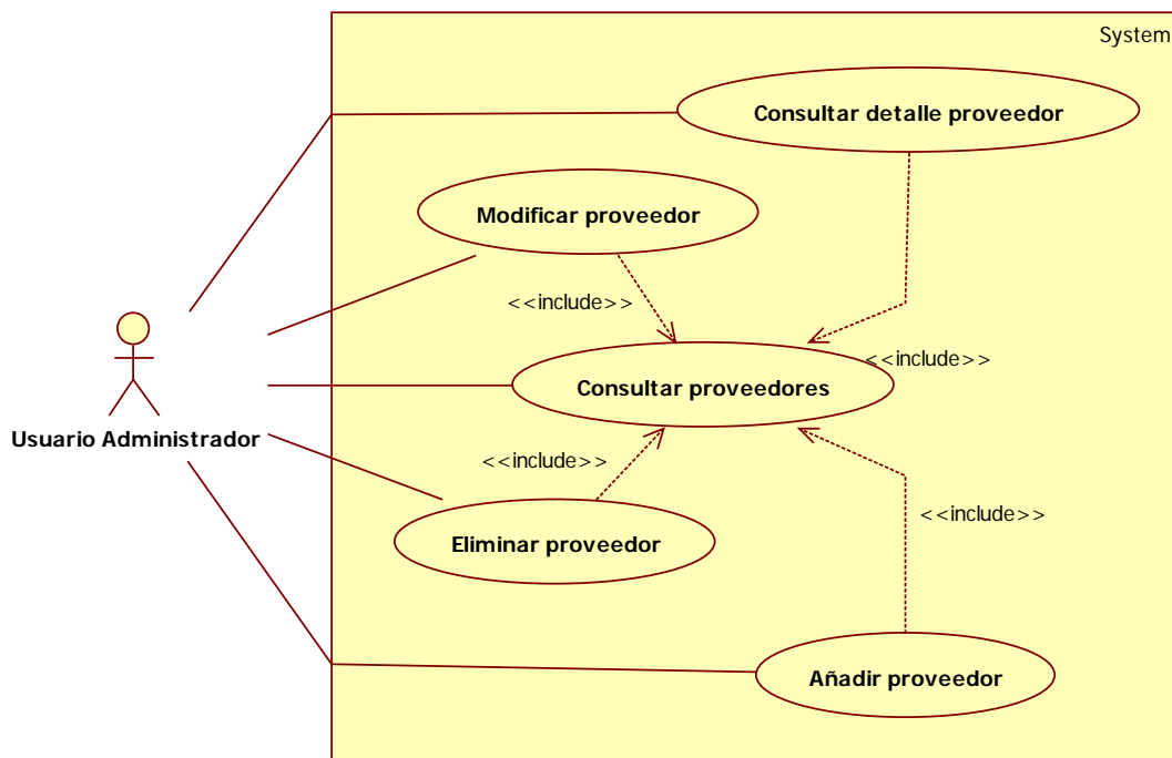
Imagen 9.5 - 26. Diagrama de casos de uso para proveedores.
