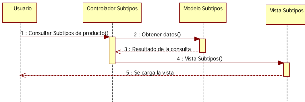
Imagen 9.5 - 21. Diagrama de secuencia CU - 17 Consultar subtipos de producto.
