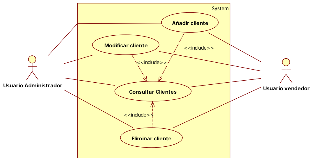
Imagen 9.5 - 56. Diagrama de casos de uso subsistema clientes.
