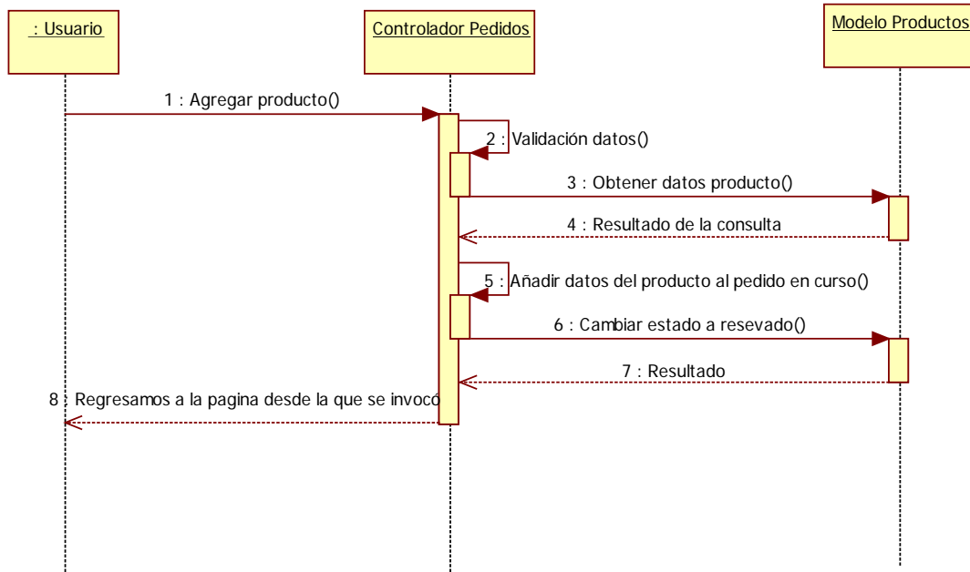
Imagen 9.5 - 45. Diagrama de secuencia CU - 37 Agregar producto a pedido.
