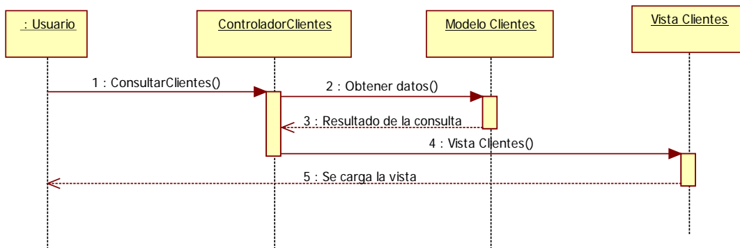
Imagen 9.5 - 57. Diagrama de secuencia CU - 47 Consultar clientes.
