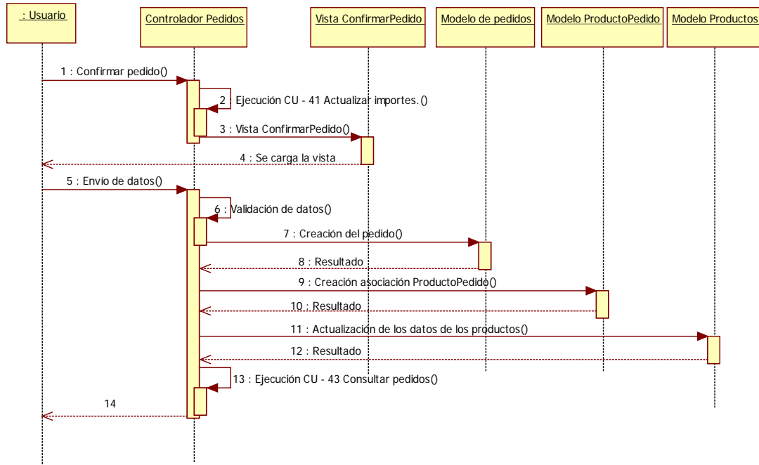
Imagen 9.5 - 50. Diagrama de secuencia CU - 42 Confirmar pedido.
