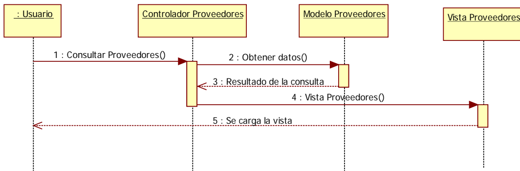
Imagen 9.5 - 27. Diagrama de secuencia CU – 22 Consultar proveedores.
