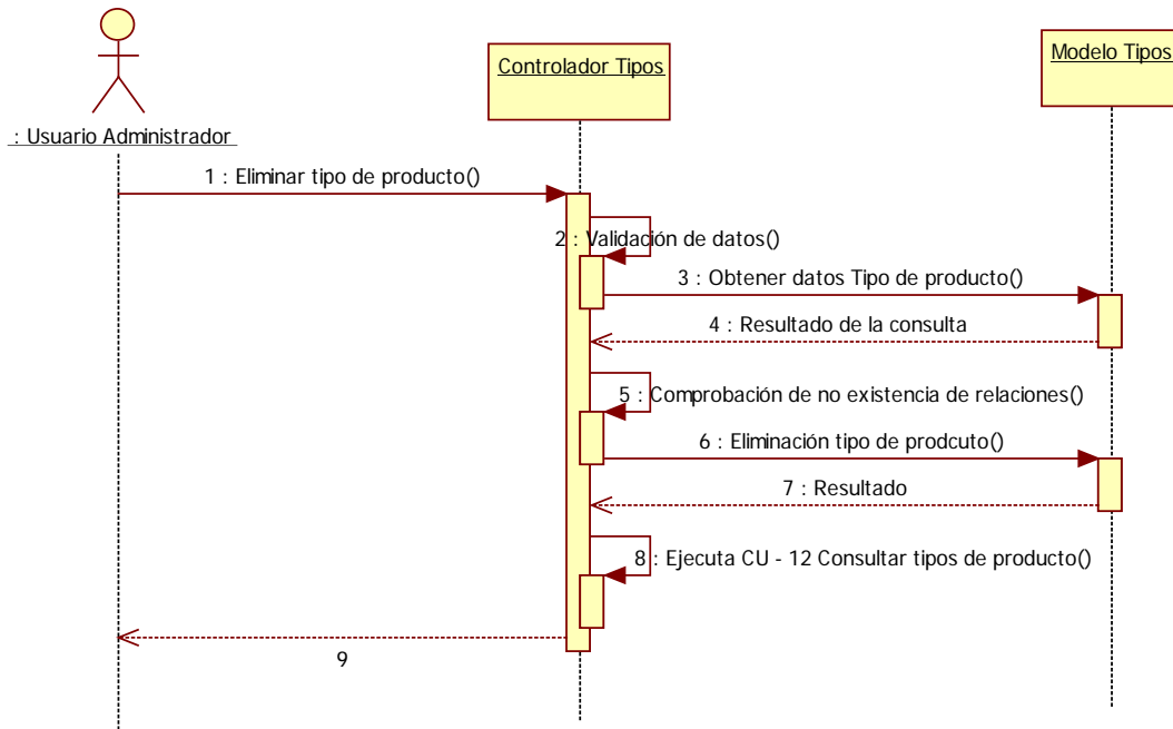
Imagen 9.5 - 19. Diagrama de secuencia CU - 16 Eliminar producto.
