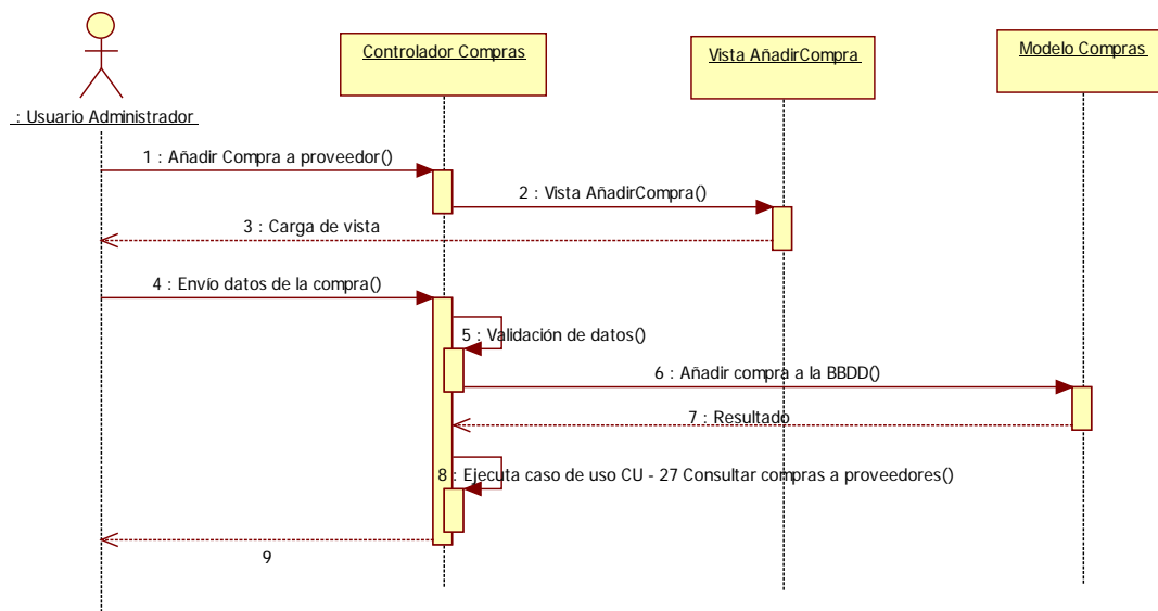
Imagen 9.5 - 34. Diagrama de secuencia CU - 28 Añadir compra a proveedor.
