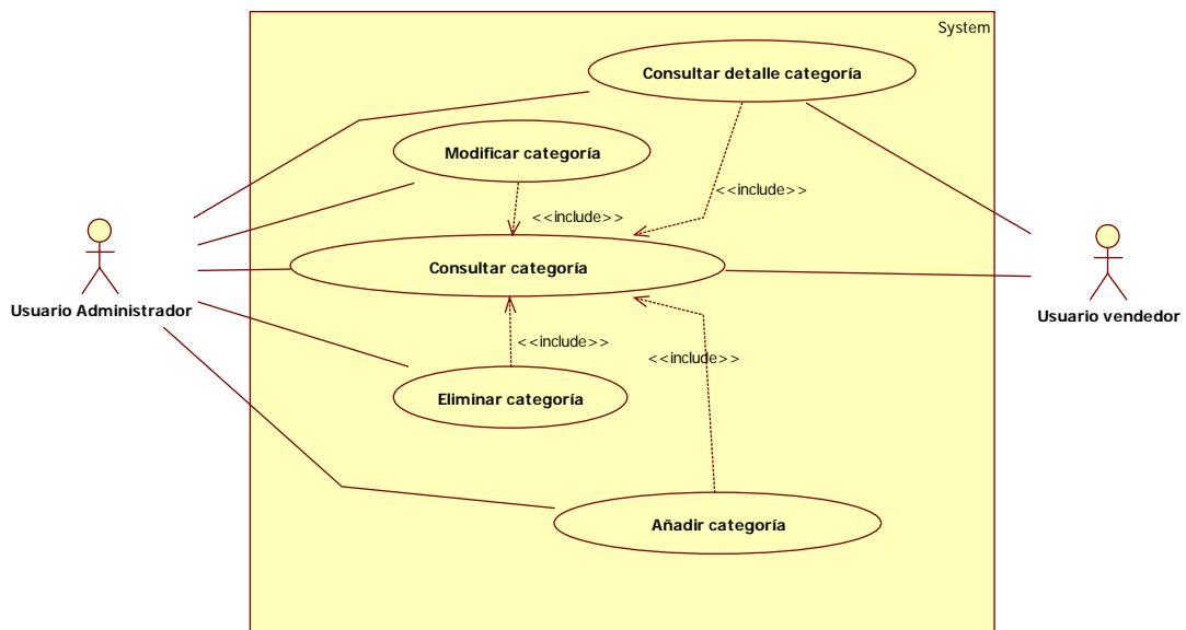
Imagen 9.5 - 9. Diagrama de casos de uso subsistema Categorías
