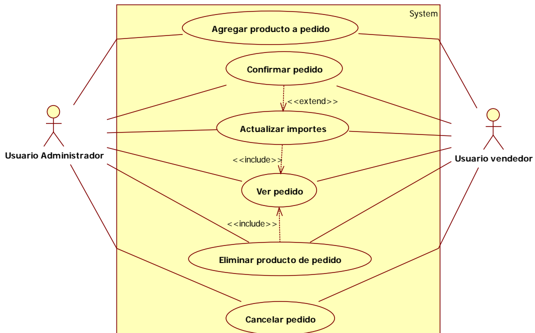
Imagen 9.5 - 44. Diagrama de casos de uso para el pedido en curso.
