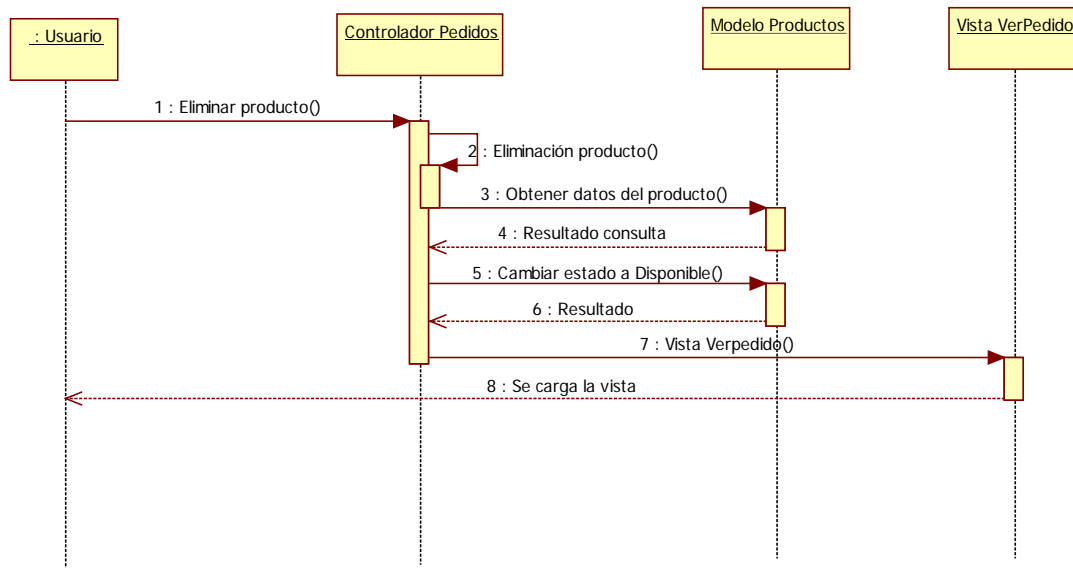
Imagen 9.5 - 47. Diagrama de secuencia CU - 39 Eliminar producto de pedido
