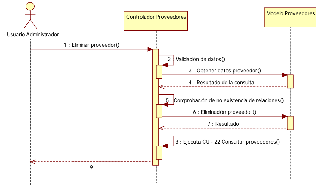
Imagen 9.5 - 31. Diagrama de secuencia CU - 26 Eliminar proveedor.
