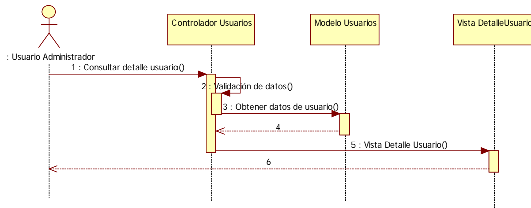
Imagen 9.5 - 6. Diagrama de secuencia CU - 05 Consultar detalle usuario
