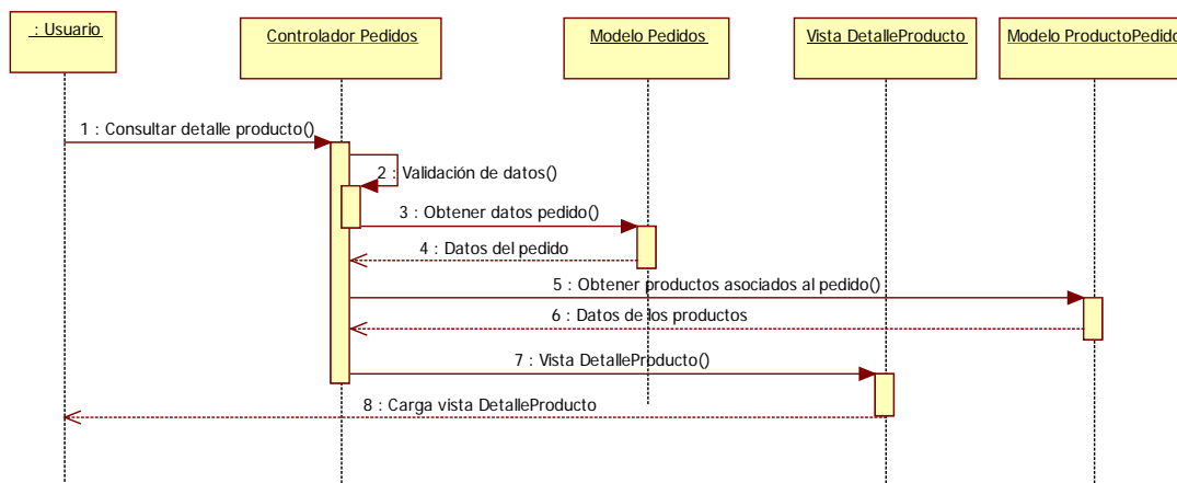
Imagen 9.5 - 54. Diagrama de secuencia CU - 45 Consultar Detalle pedido.
