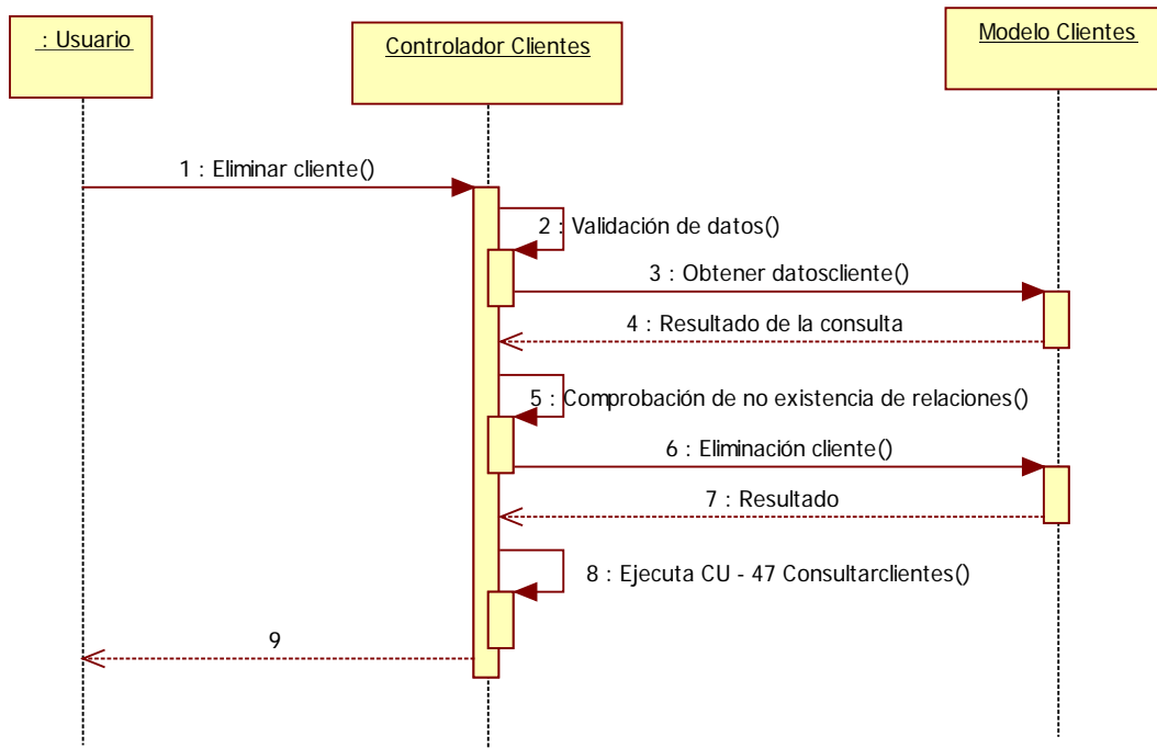
Imagen 9.5 - 61. Diagrama de secuencia CU – 51 Eliminar cliente.
