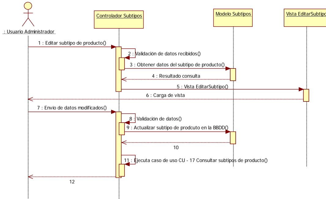
Imagen 9.5 - 23. Diagrama de secuencia CU - 19 Modificar subtipo de producto.
