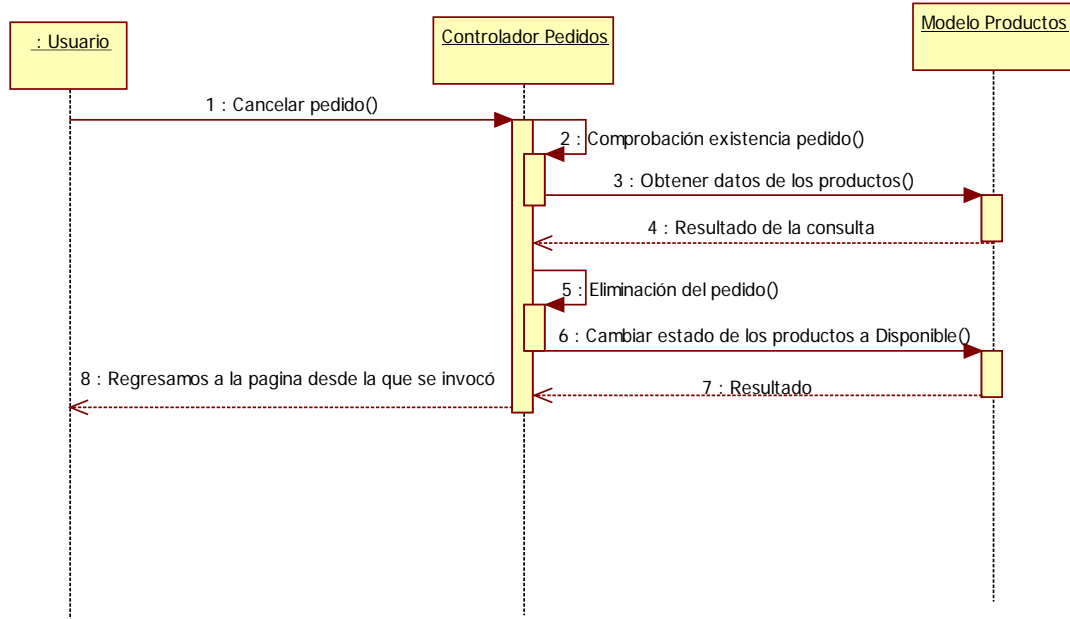
Imagen 9.5 - 48. Diagrama de secuencia CU - 40 Cancelar pedido
