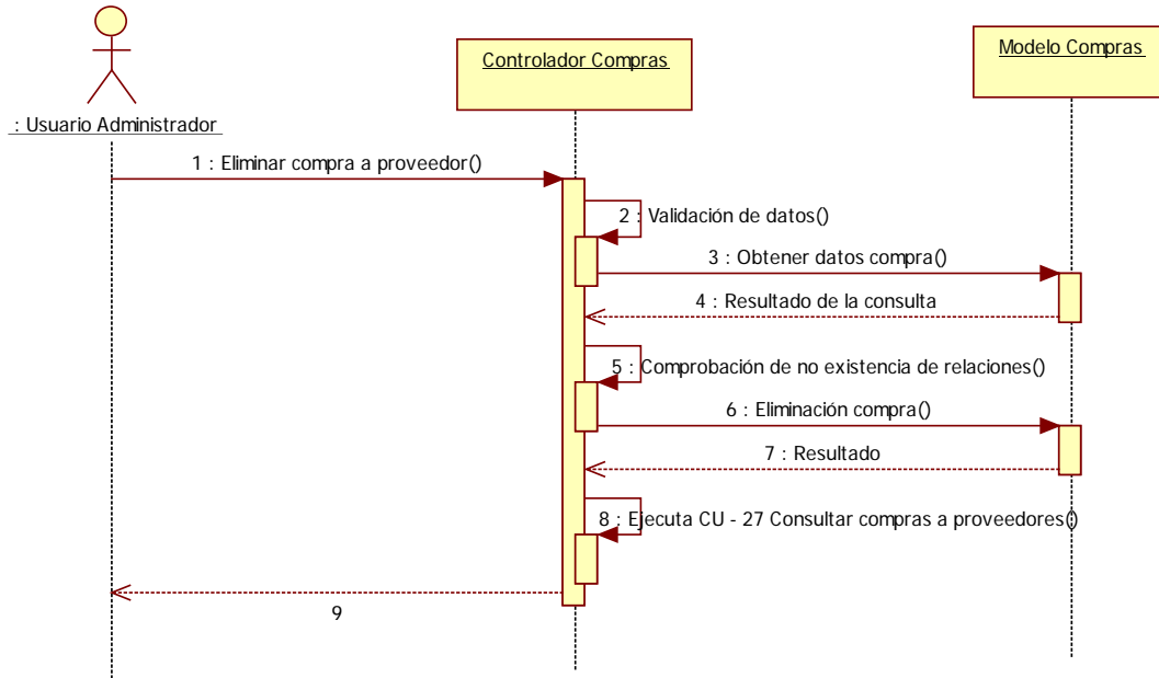
Imagen 9.5 - 37. Diagrama de secuencia CU – 31 Eliminar compra a proveedor.
