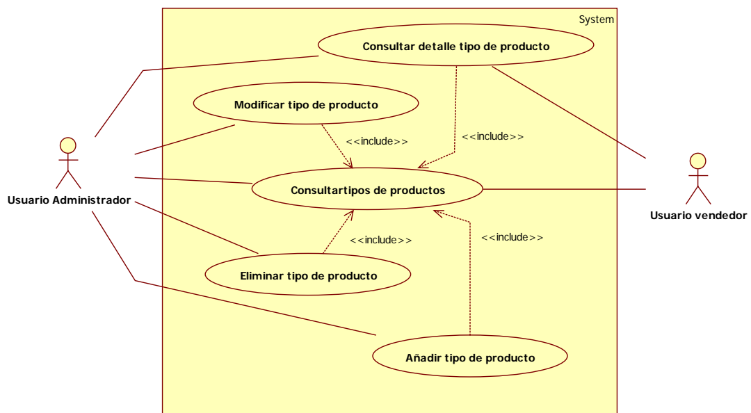
Imagen 9.5 - 1. Diagrama de casos de uso del subsistema Tipos de producto.
