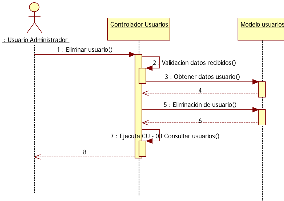
Imagen 9.5 - 7. Diagrama de secuencia CU - 06 Eliminar usuario
