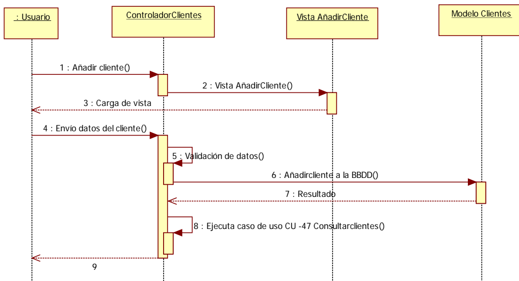
Imagen 9.5 - 58. Diagrama de secuencia CU - 48 Añadir cliente.
