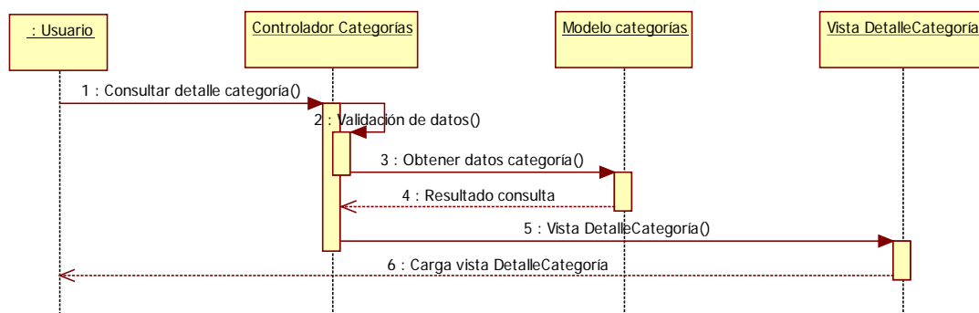
Imagen 9.5 - 13. Diagrama de secuencia CU - 10 Consultar detalle categoría
