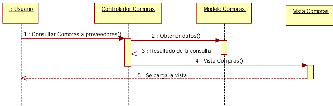
Imagen 9.5 - 33. Diagrama de secuencia CU - 27 Consultar compras a proveedores.
