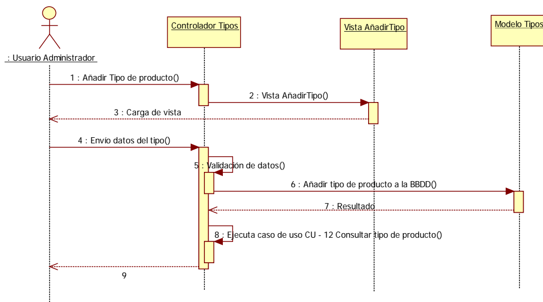
Imagen 9.5 - 16. Diagrama de secuencia CU - 13 Añadir tipo de producto.
