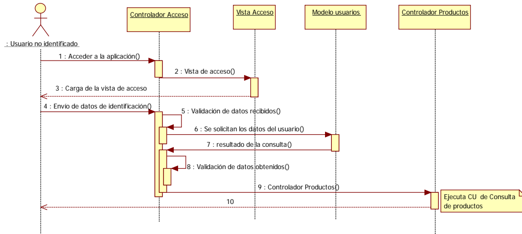
Imagen 9.5 - 2. Diagrama de secuencia CU – 01 Validar usuario.
