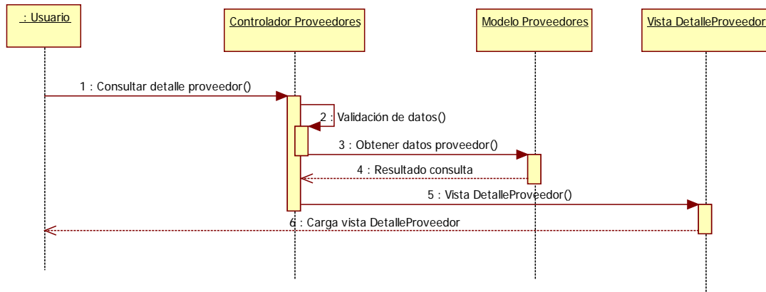
Imagen 9.5 - 30. Diagrama de secuencia CU - 25 Consultar detalle proveedor
