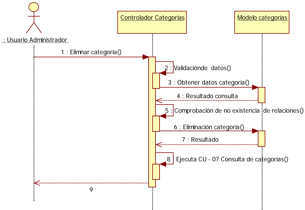
Imagen 9.5 - 14. Diagrama de secuencia CU - 11 Eliminar categoría
