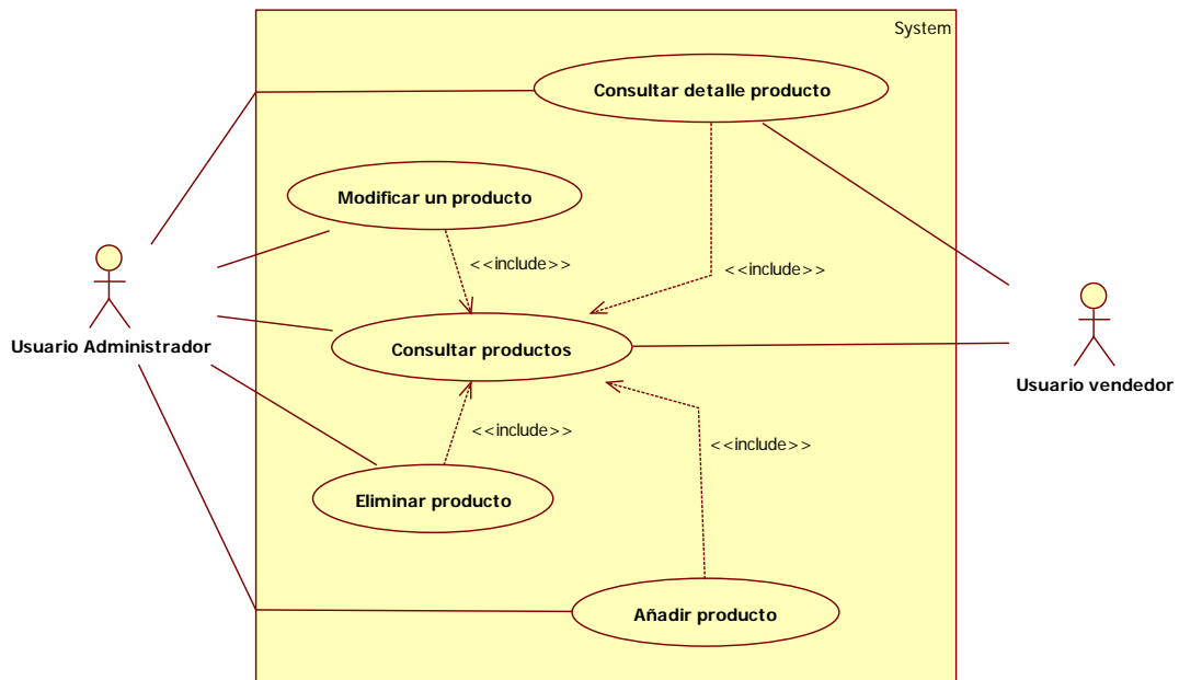
Imagen 9.5 - 38. Diagrama de casos de uso subsistema Productos.
