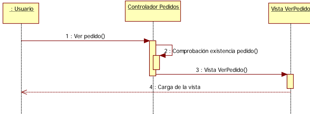
Imagen 9.5 - 46. Diagrama de secuencia CU – 38 Ver pedido.
