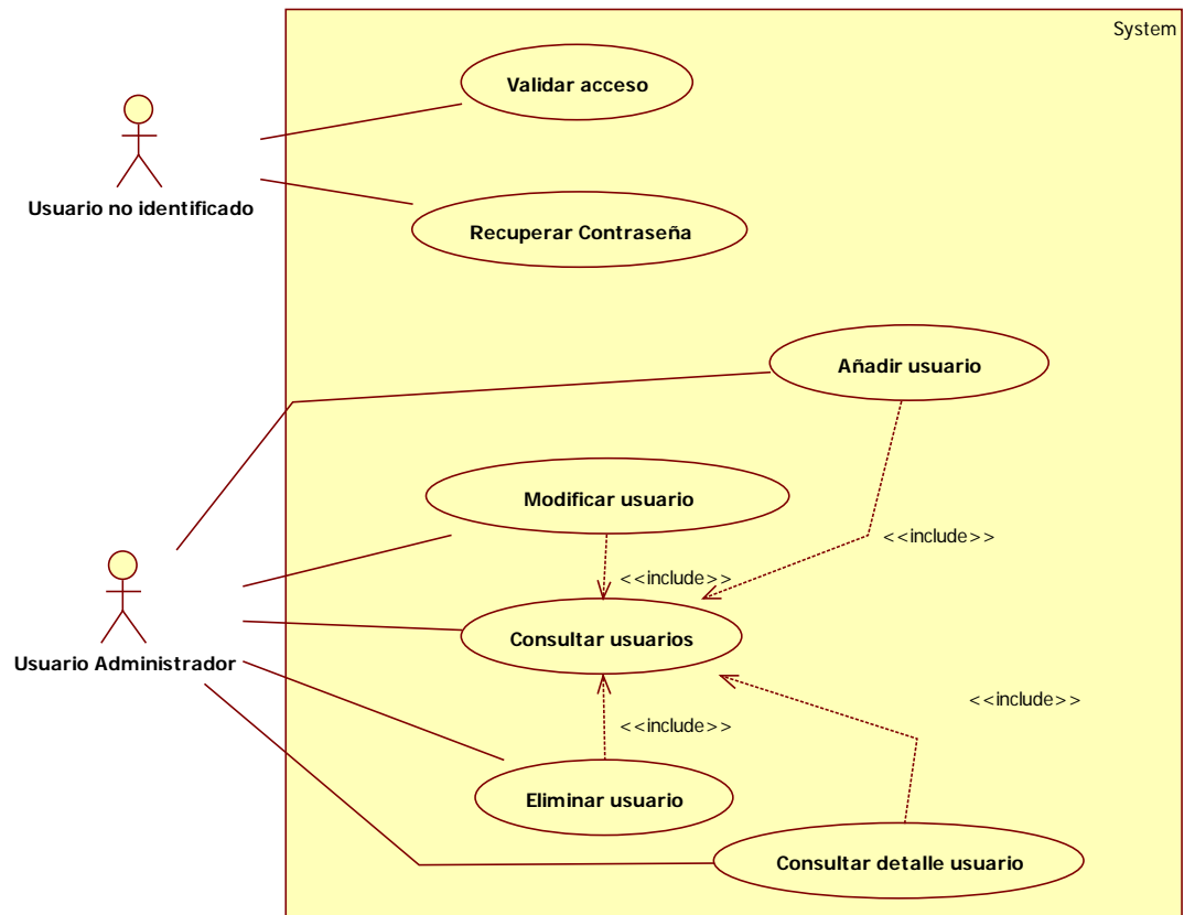
Imagen 9.5 - 1. Diagrama de casos de uso subsistema usuarios.
