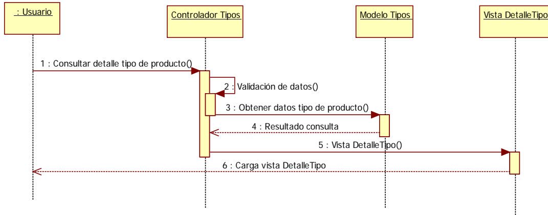
Imagen 9.5 - 18. Diagrama de secuencia CU - 15 Consultar detalle tipo de producto.
