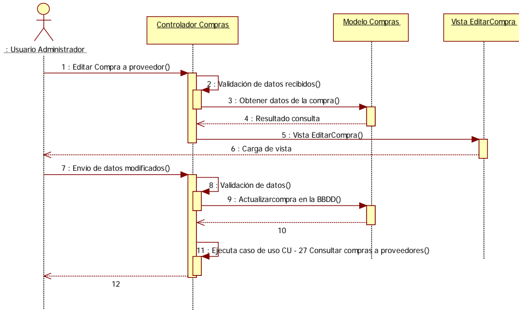
Imagen 9.5 - 35. Diagrama de secuencia CU - 29 Modificar compra a proveedor
