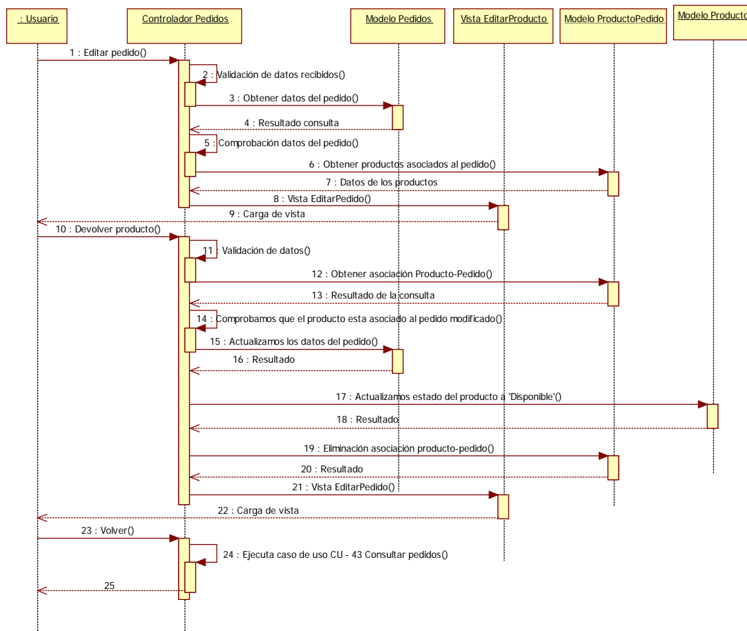
Imagen 9.5 - 53. Diagrama de secuencia CU - 44 Modificar pedido.
