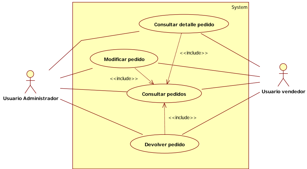
Imagen 9.5 - 51. Diagrama de casos de uso para pedidos confirmados.
