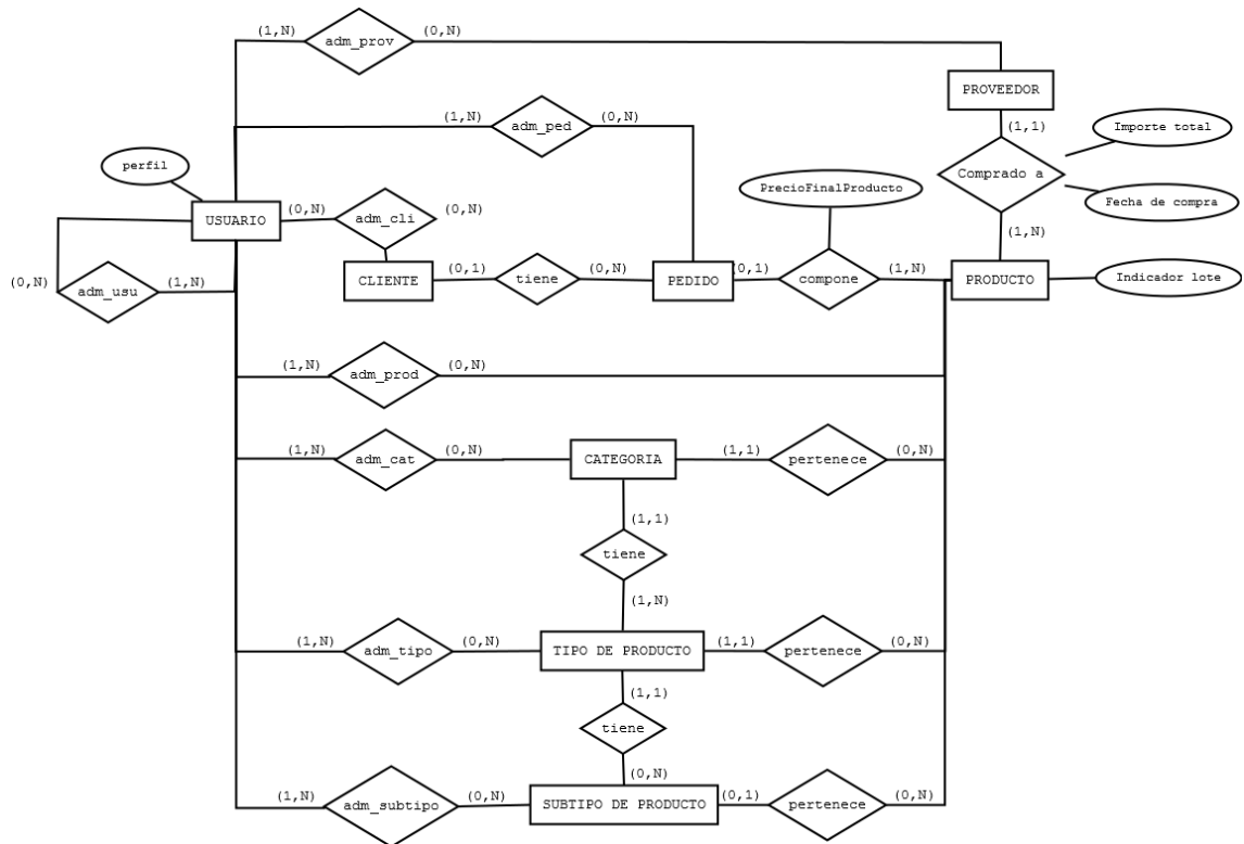
Imagen 10.2 - 1. Diagrama entidad-relación.
