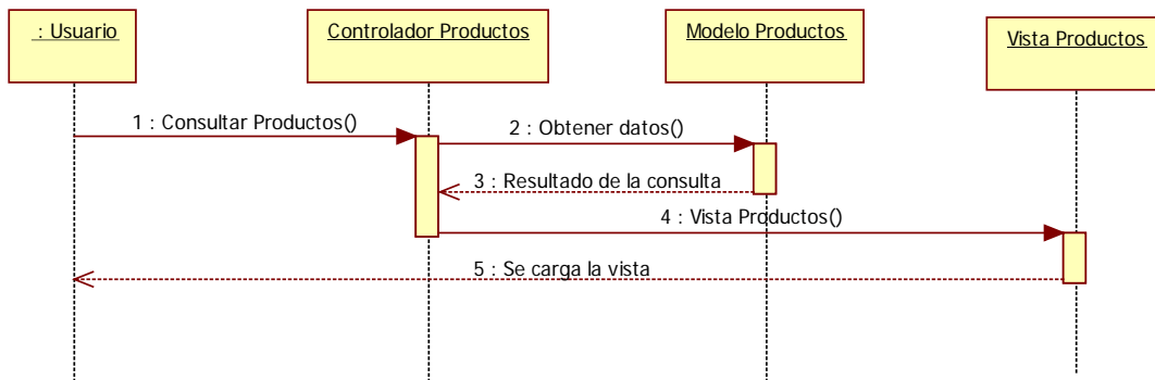
Imagen 9.5 - 39. Diagrama de secuencia CU - 32 Consultar productos.
