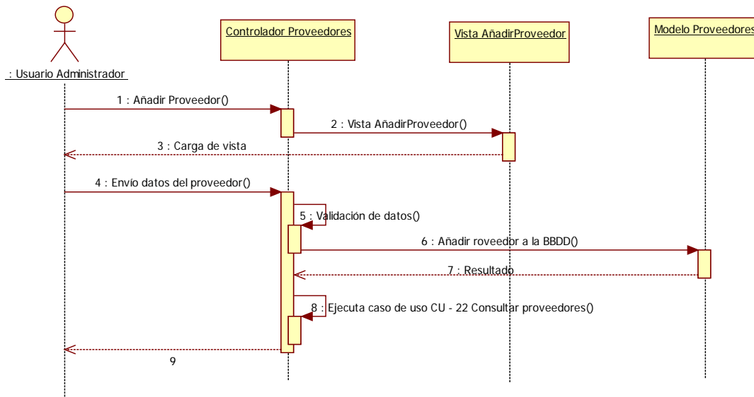
Imagen 9.5 - 28. Diagrama de secuencia CU - 23 Añadir proveedor.
