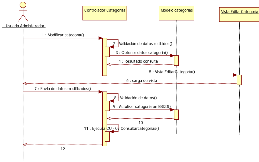
Imagen 9.5 - 12. Diagrama de secuencia CU - 09 Modificar categoría.
