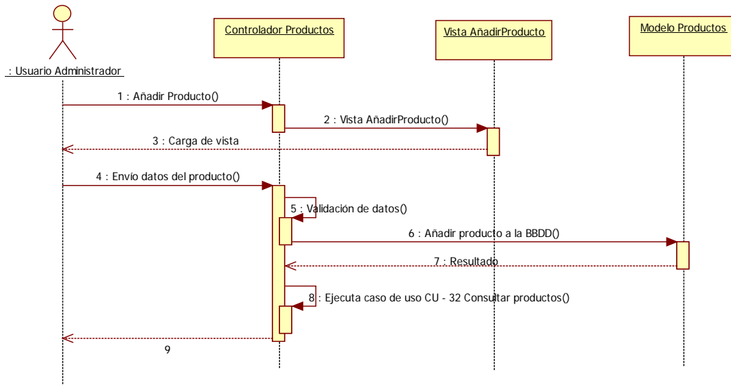
Imagen 9.5 - 40. Diagrama de secuencia CU - 33 Añadir producto.
