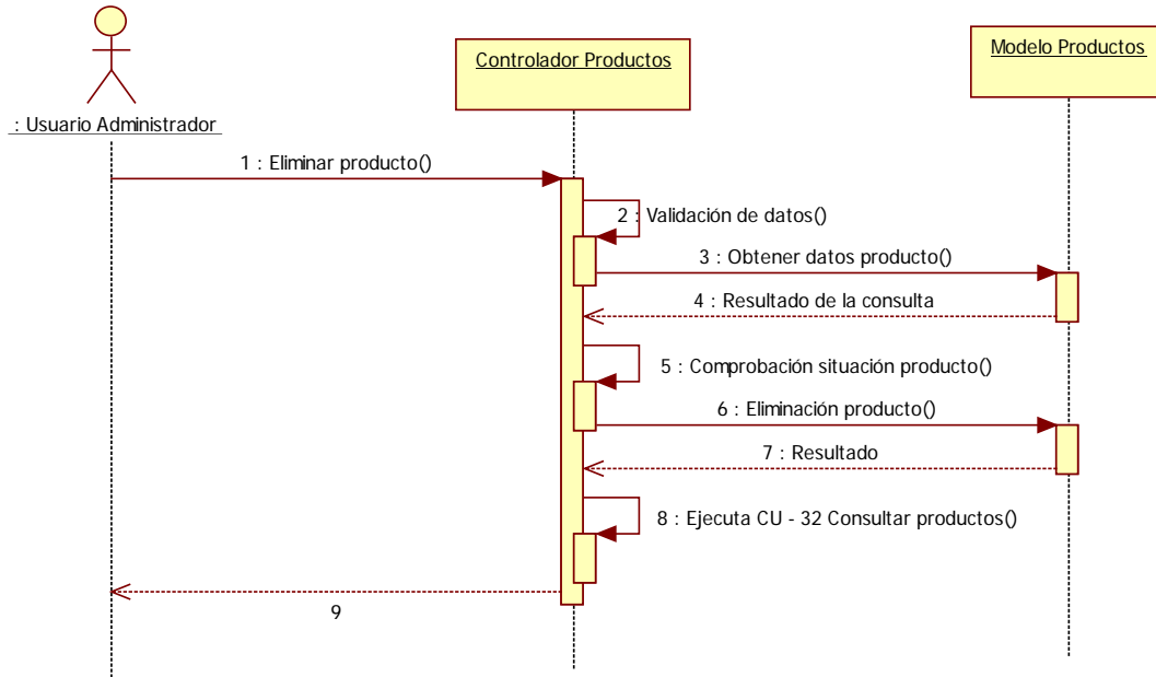
Imagen 9.5 - 43. Diagrama de secuencia CU - 36 Eliminar producto.
