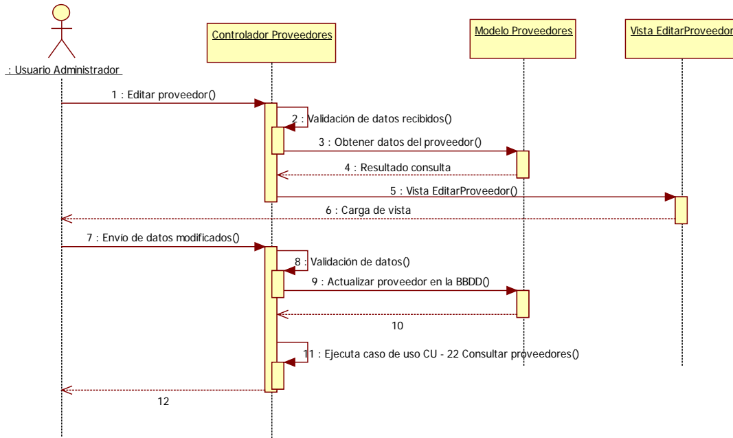
Imagen 9.5 - 29. Diagrama de secuencia CU - 24 Modificar proveedor.
