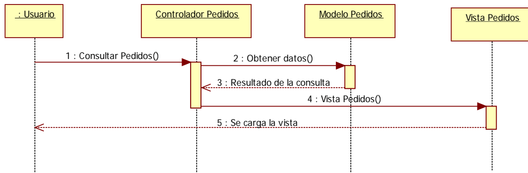
Imagen 9.5 - 52. Diagrama de secuencia CU - 43 Consultar pedidos.
