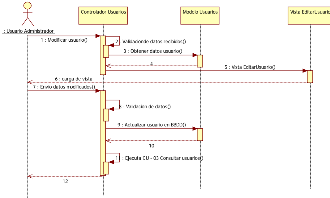
Imagen 9.5 - 5. Diagrama de secuencia CU - 04 Modificar usuario.
