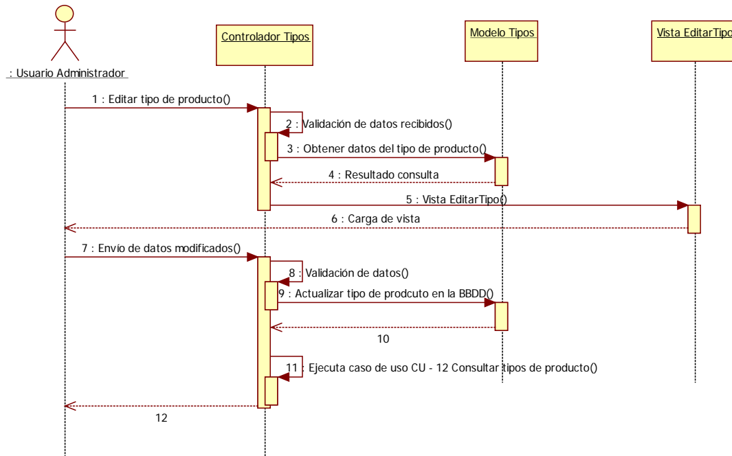
Imagen 9.5 - 17. Diagrama de secuencia CU- 14 Modificar tipo de producto.
