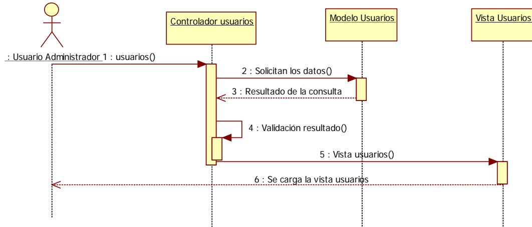
Imagen 9.5 - 4. Diagrama de secuencia CU - 03 Consultar usuarios.
