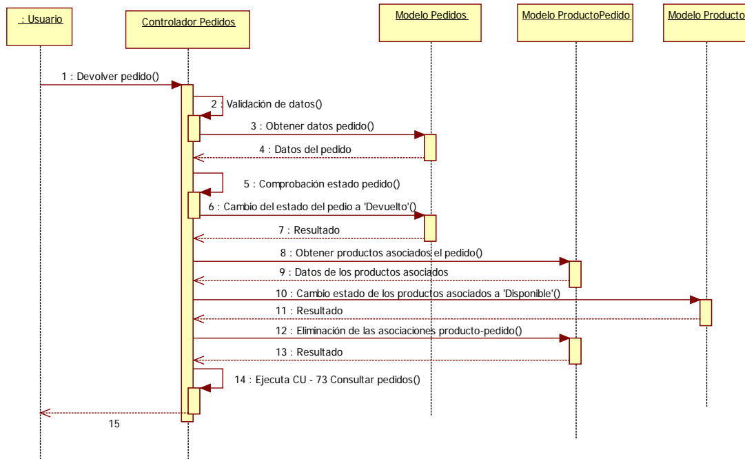
Imagen 9.5 - 55. Diagrama de secuencia CU - 46 Devolver pedido.
