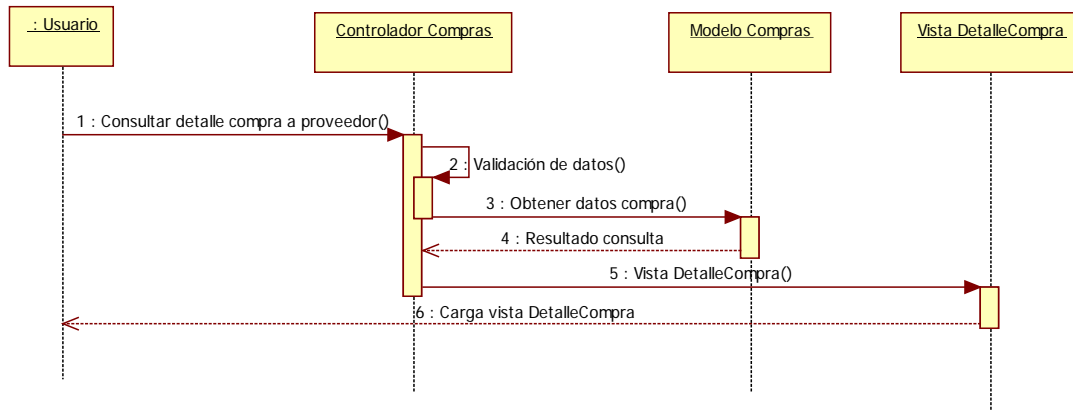
Imagen 9.5 - 36. Diagrama de secuencia CU - 30 Consultar detalle compra a proveedor.
