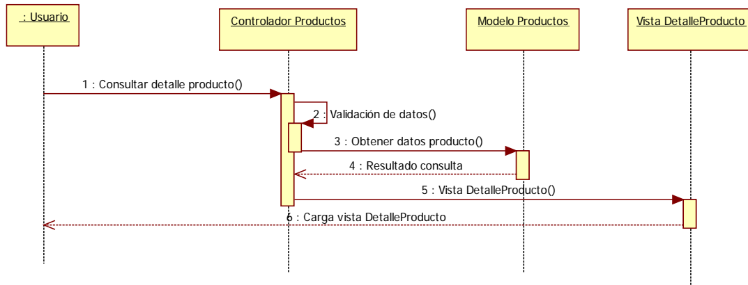
Imagen 9.5 - 42. Diagrama de secuencia CU - 35 Consultar detalle producto.
