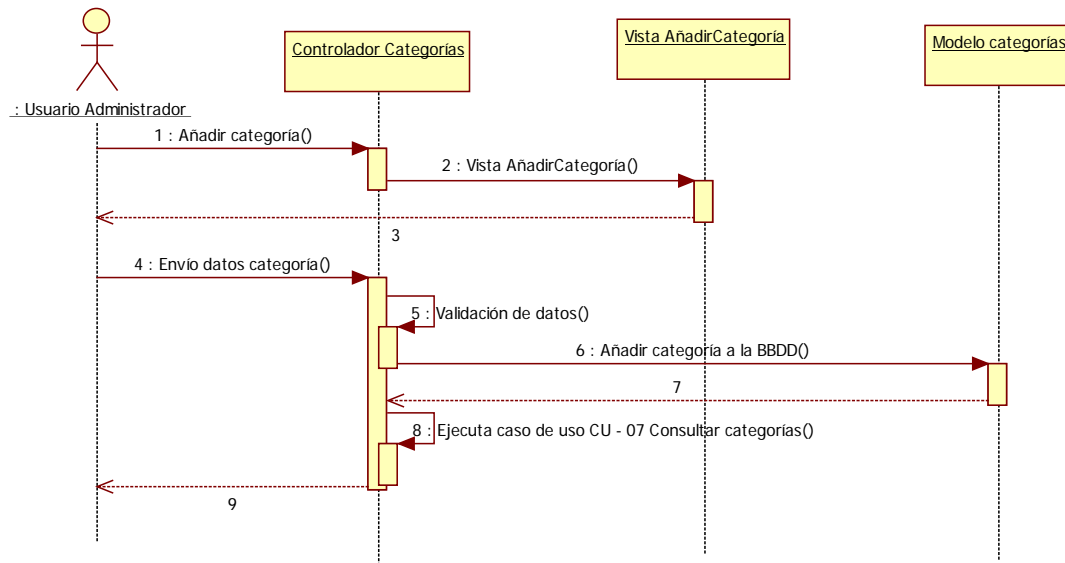
Imagen 9.5 - 11. Diagrama de secuencia CU - 08 Añadir categoría.
