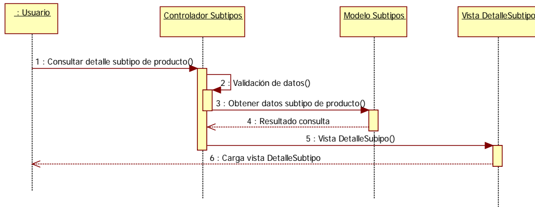
Imagen 9.5 - 24. Diagrama de secuencia CU - 20 Consultar detalle subtipo de producto.
