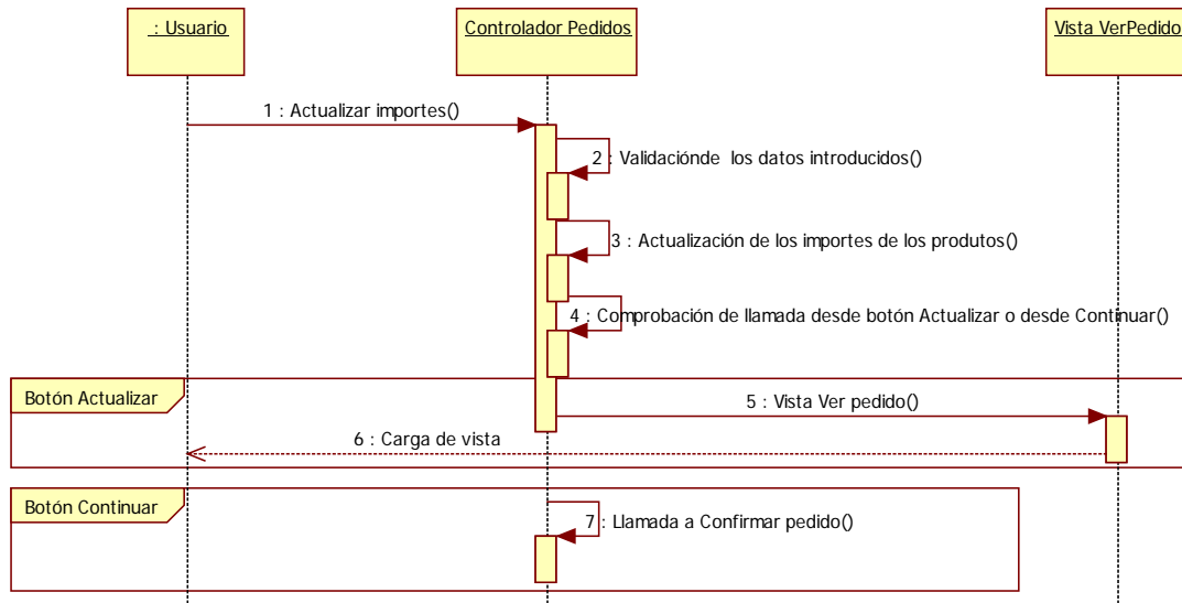
Imagen 9.5 - 49. Diagrama de secuencia CU - 41 Actualizar importes.
