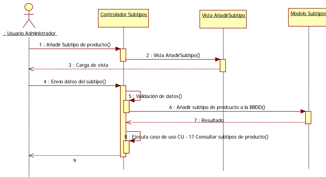
Imagen 9.5 - 22. Diagrama de secuencia CU - 18 Añadir subtipo de producto.
