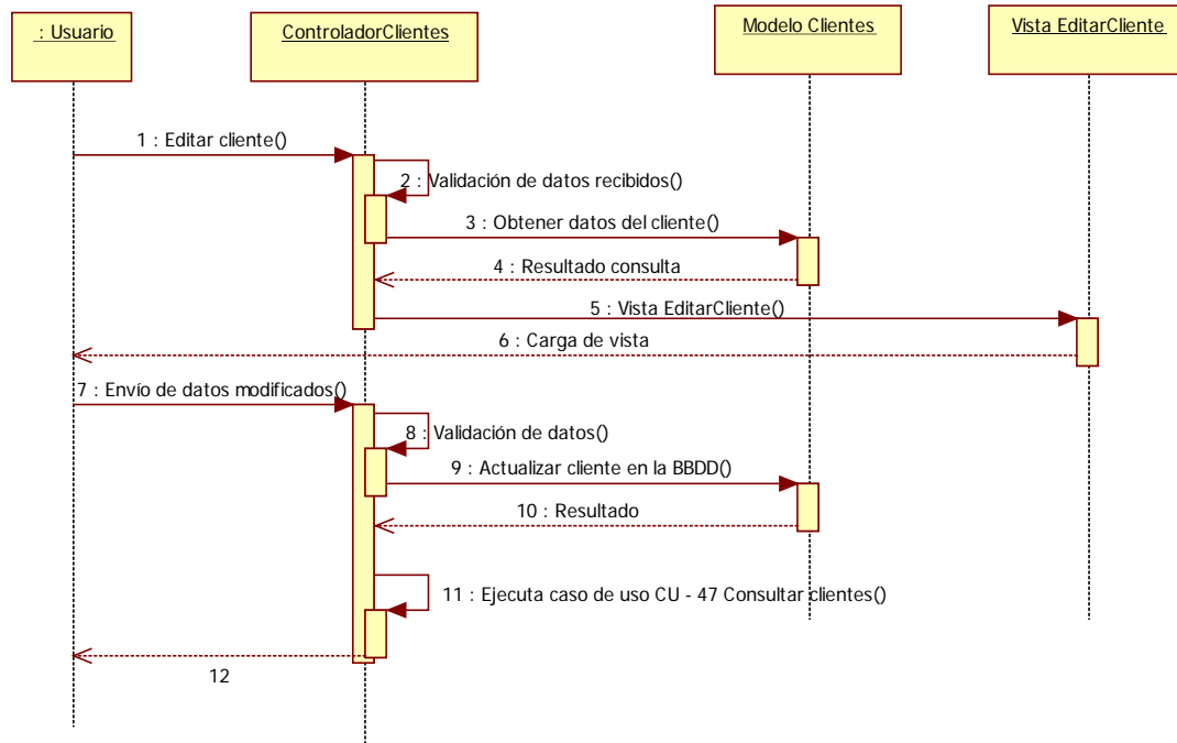
Imagen 9.5 - 59. Diagrama de secuencia CU - 49 Modificar cliente.
