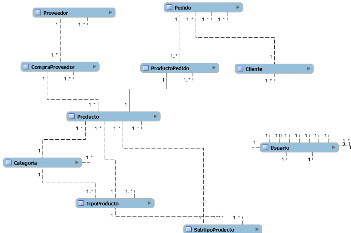
Imagen 10.2 - 2. Diagrama modelo relacional (solo relaciones)
