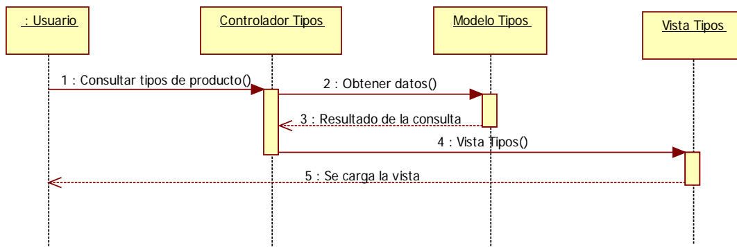
Imagen 9.5 - 15. Diagrama de secuencia CU - 12 Consultar tipos de producto
