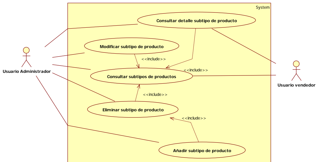
Imagen 9.5 - 20. Diagrama de casos de uso del subsistema Subtipos de producto
