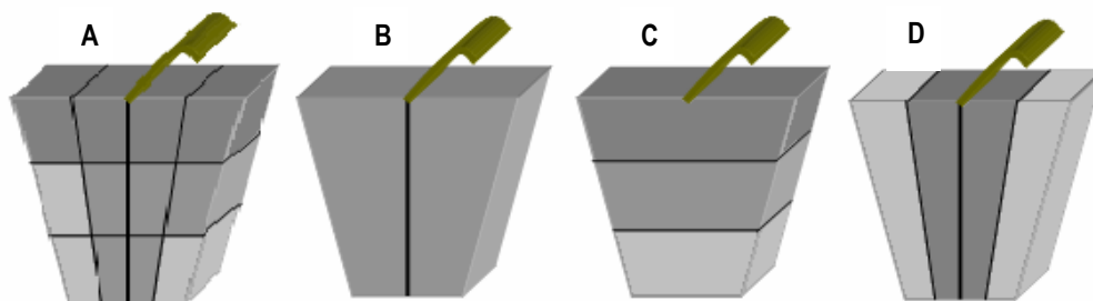
Figura I.5. Concentración de azúcares (°Brix) según intensidad de tonalidad en las distintas zonas del racimo. A: Partes individualizadas. B: Zonas Exterior-Interior. C: Tercios Superior-Medio-Inferior. D: Zonas Superficiales-no Superficiales (Yuste et al. 2009).
