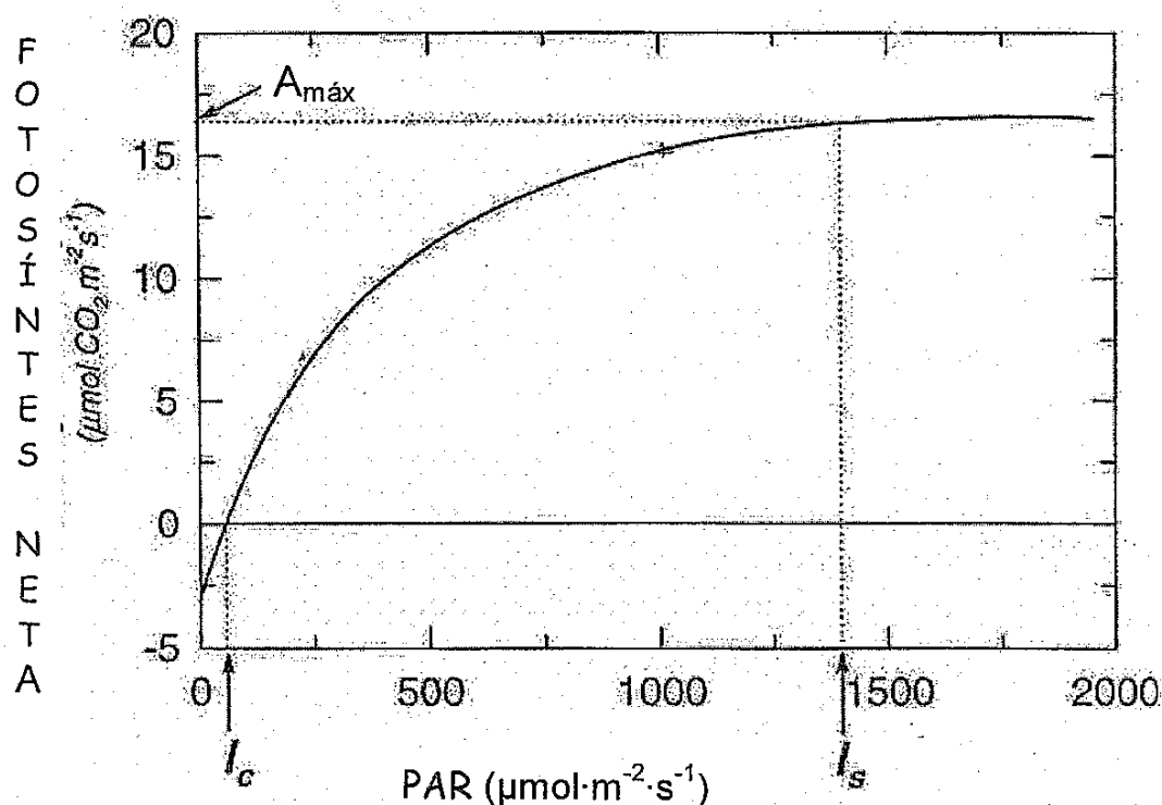
Figura I.4. Representación esquemática de la influencia de la iluminación (PAR) en la fotosíntesis neta de hojas adultas del cv. Chasselas, medida a temperatura óptima (25 a 30 °C). A_{\text{máx}} : asimilación neta máxima, I_s : índice de saturación luminosa. I_c : punto de compensación (Zufferey y Murisier 2000).
