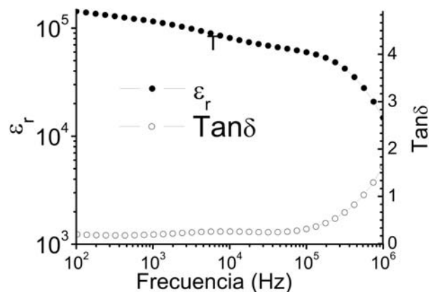
Fig. 3. Valores de permitividad dieléctrica y factor de pérdida para las muestras de CCTO.
