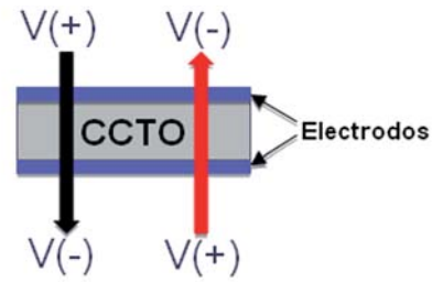
Fig. 2. Esquema de las mediciones macroscópicas de la muestra en CC.
