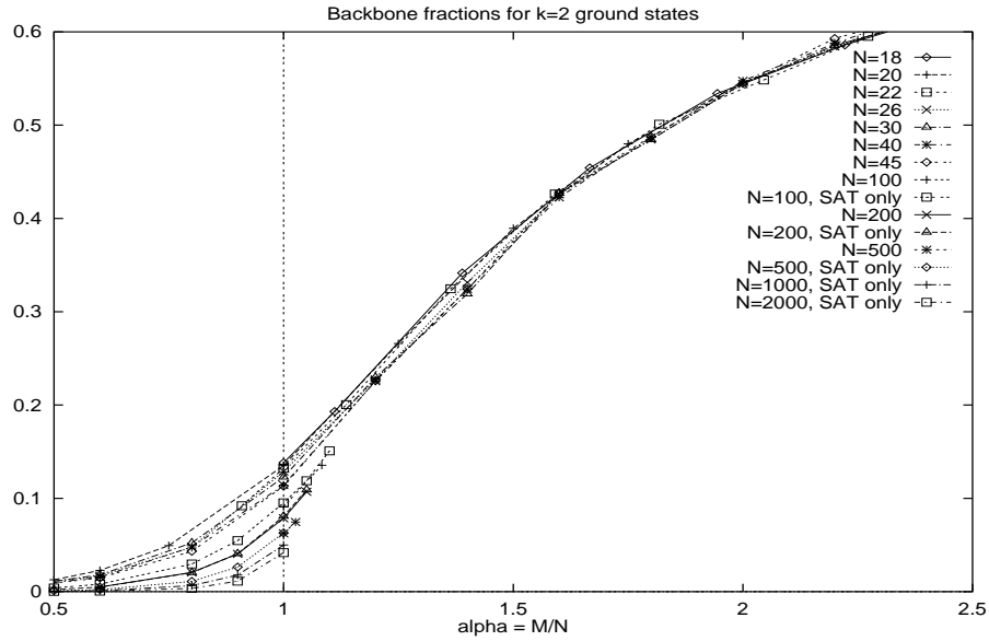
fig. 9a: Backbone fraction for K = 2 .
