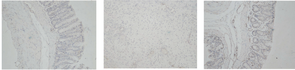
NS IA IA + PN (1.0 g/kg)
