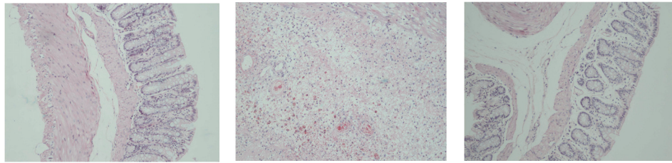
NS IA IA + PN (1.0 g/kg)
