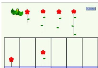
Figura 6: seriación (S1)
