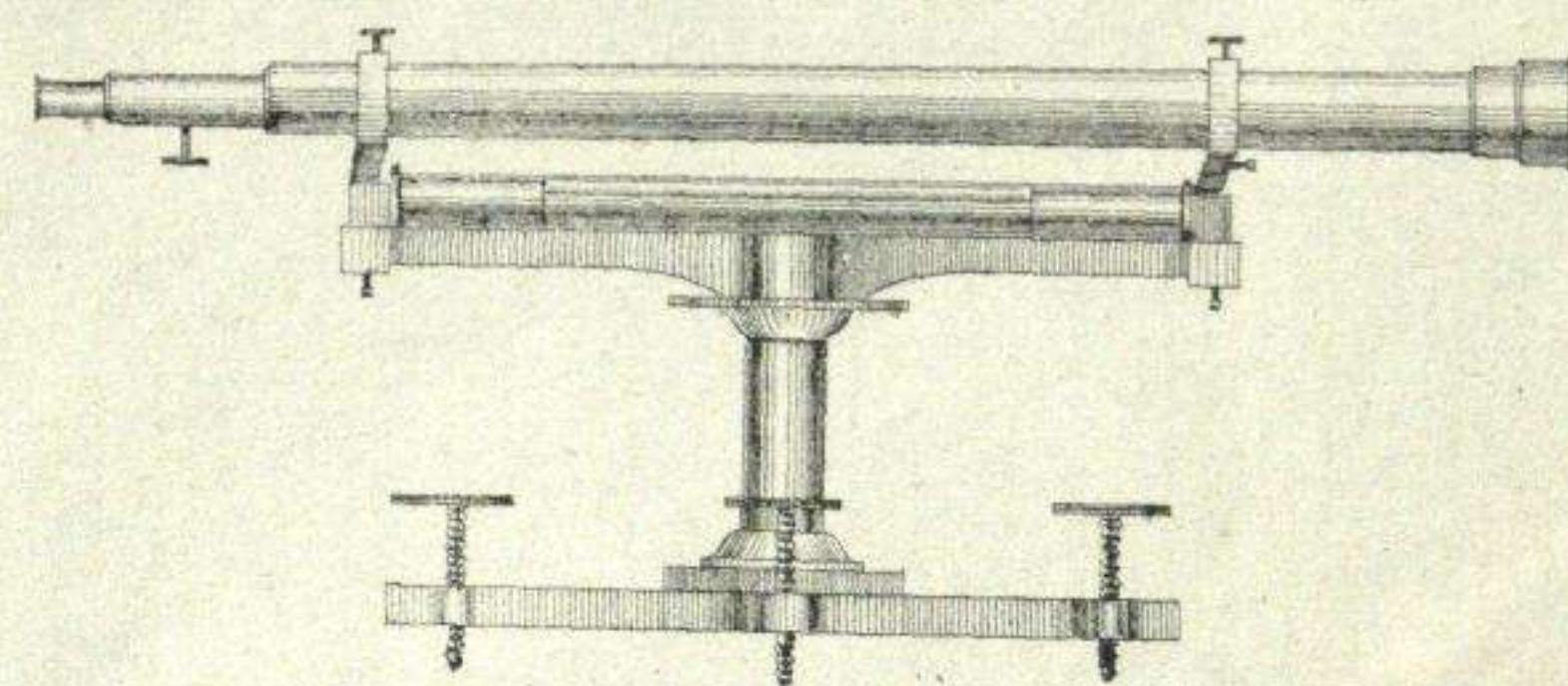
Nivel d' Egault. Fig. n.º 10.
