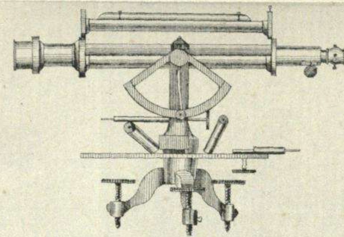
Nivel con circulo horizontal y arco de alturas. Fig. n.º 13. Sin circulo ni arco. , 11.
