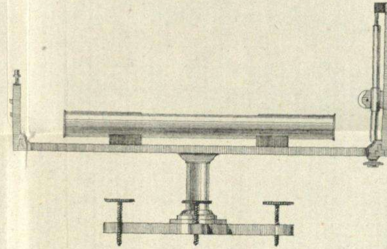
Eclimetro sin brújula. Fig. n.º 6.
