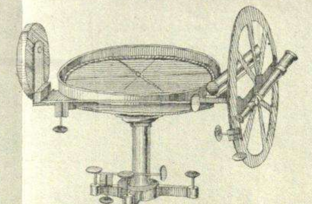
Brújula-Eclimetro. Fig. n.º 7.
