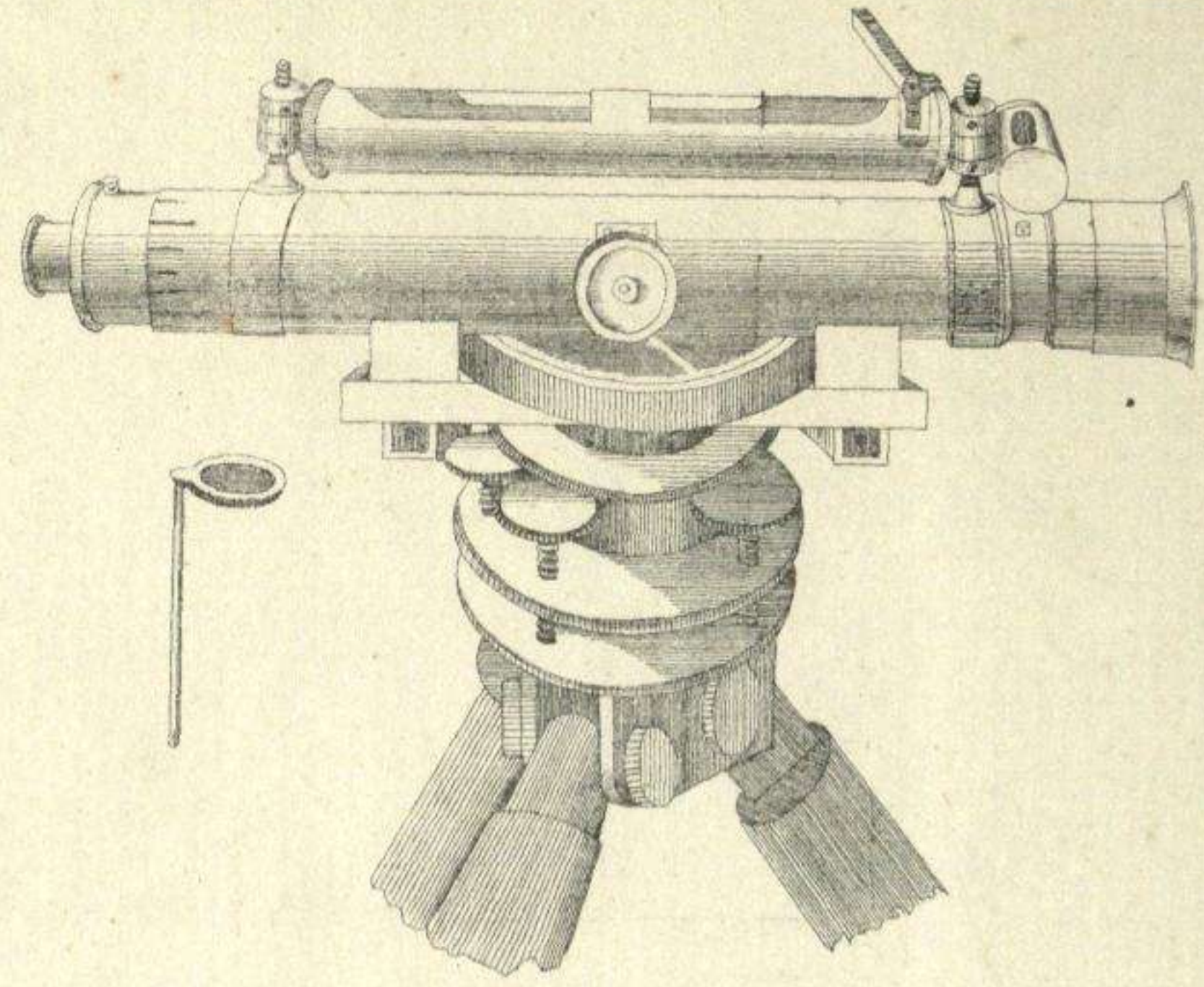
Nivel de Gravatt. Fig. n.º 14.
