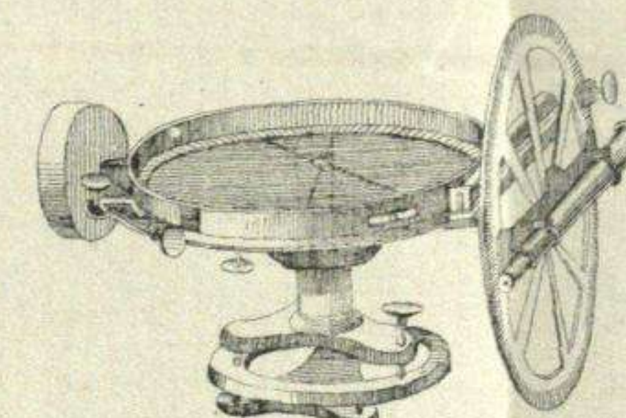
Brújula-Eclimetro. Fig. n.º 8.
