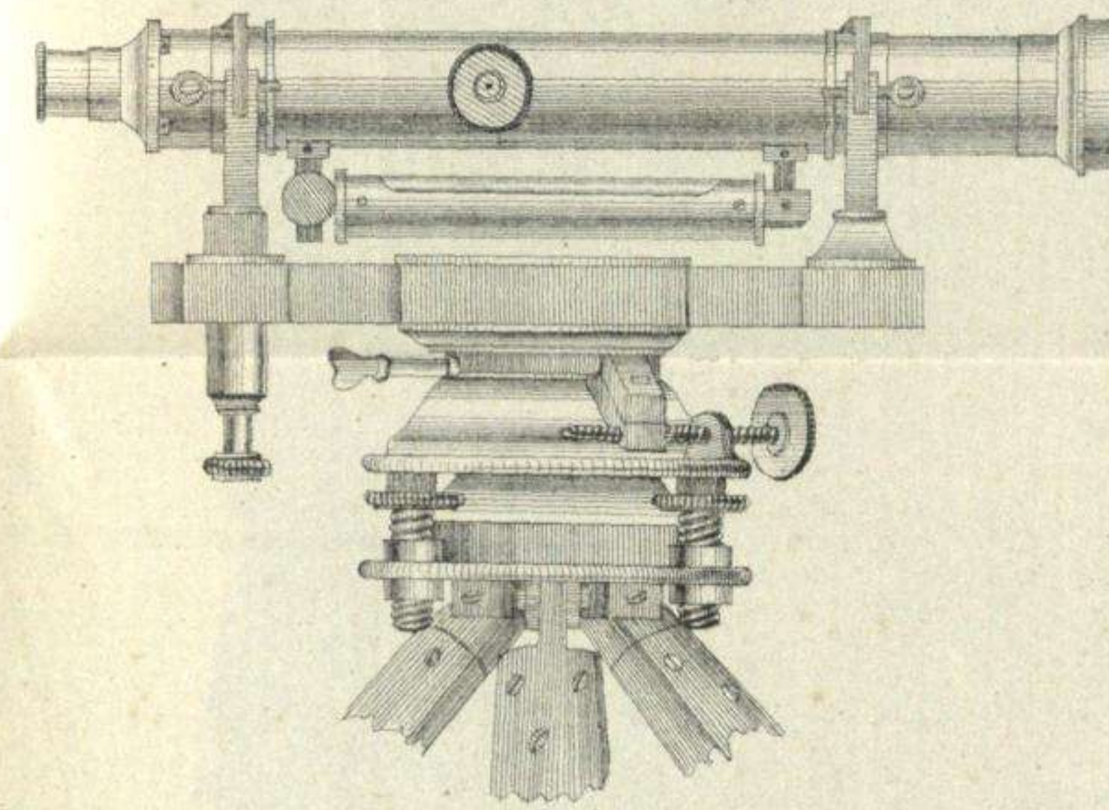
Nivel ingles de 4 tornillos. Fig. n.º 3.
