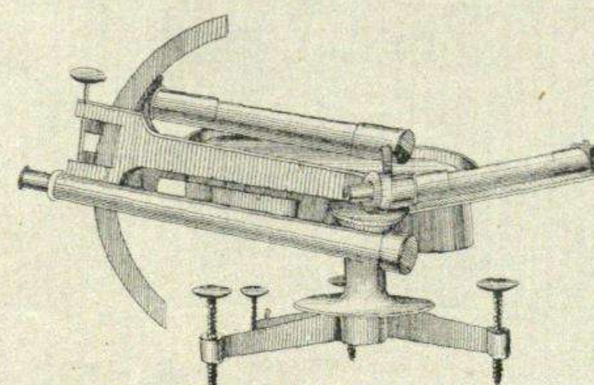
Brújula-Eclimetro. Fig. n.º 12.
