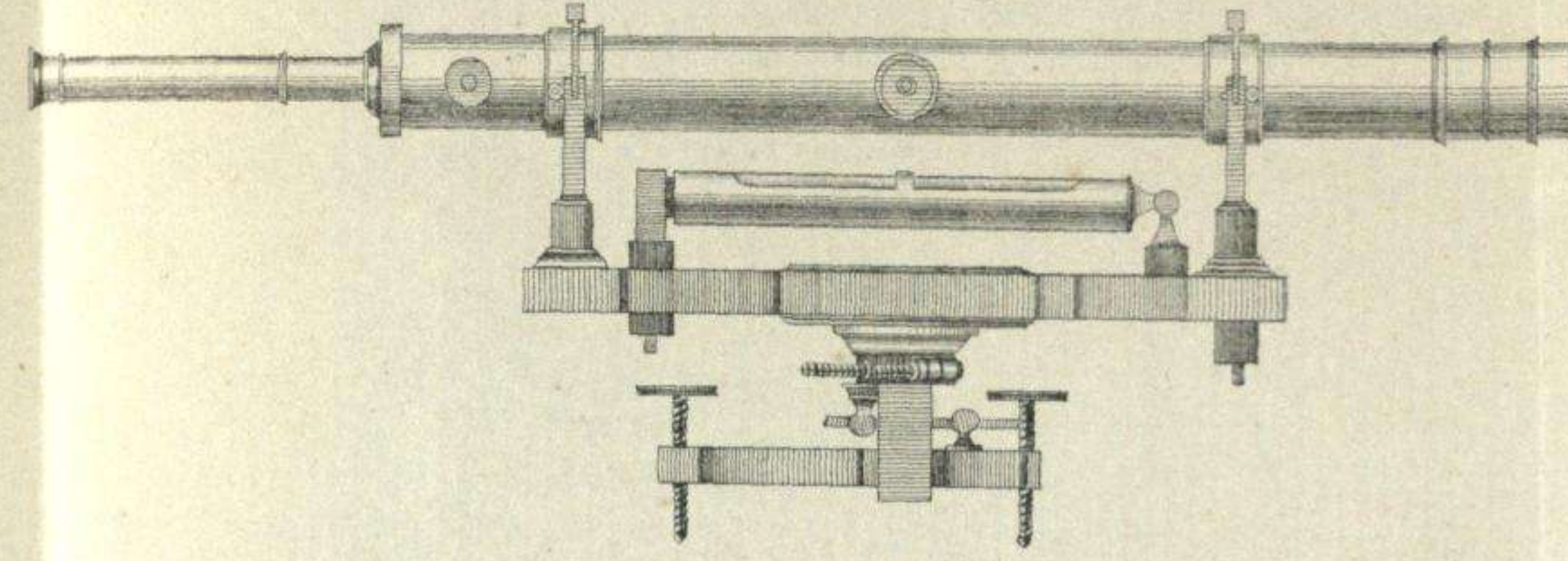
Nivel ingles perfeccionado. Fig. n.º 2.
