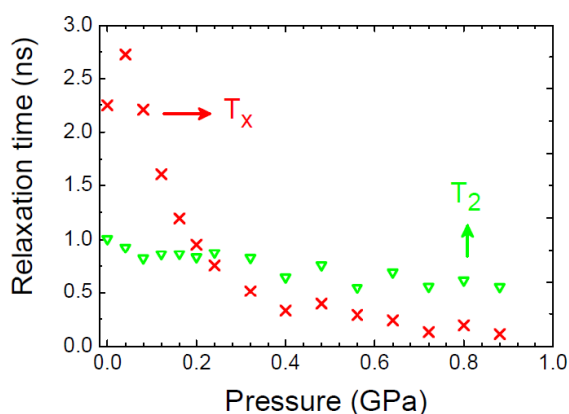
4. ábra: A rétegek közötti ( T_x ) és a rétegen belüli ( T_2 ) spinrelaxációs idő nyomásfüggése a \kappa -(BEDT-TTF) 2 Cu[N(CN) 2 ]Cl-ben 250 K-en. A két és háromdimenziós spintranszport közötti „cross-over” 0.2 GPa körül van.
