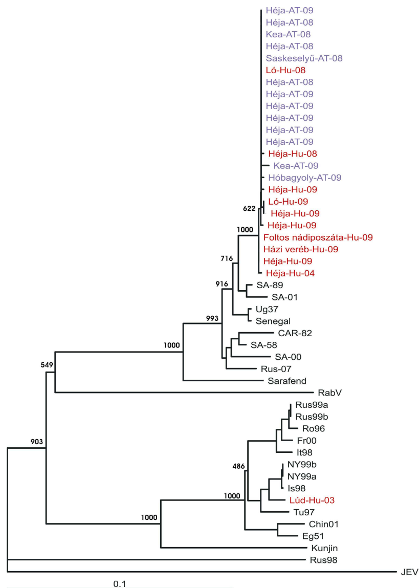
2. ábra: Az E fehérje régió részleges nukleotid szekvenciáinak Neighbor-Joining algoritmussal végzett filogenetikai analízise alapján készített törzsfá. A vizsgálataink során meghatározott szekvenciákat gazdafaj - ország kód (Hu: Magyarország, AT: Ausztria) - kimutatás éve (08: 2008, 09: 2009) kódokkal jelöltük. A magyarországi törzseket piros színnel, az ausztriai törzseket kék színnel emeltük ki. A génbanki szekvenciák kódjainak feloldását a függelék 2. táblázata tartalmazza. Az elágazódásoknál olvasható számok a bootstrap analízis értékeit mutatják (1000 ismétlés, csak a nagyobb elágazódásoknál kiírva). Az ábra bal alsó sarkában a lépték a genetikai távolságot mutatja.
