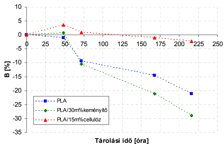
10. ábra Tömegváltozás 80°C-os enzimés bontás során
