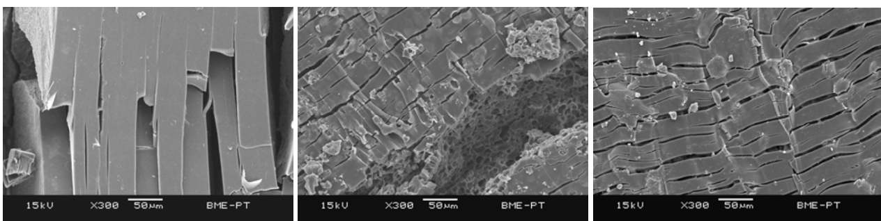
12. ábra PLA (a), PLA/30m% keményítő (b) és PLA/15m% cellulóz (c) felszíne 80°C-os enzimatis bontás után
