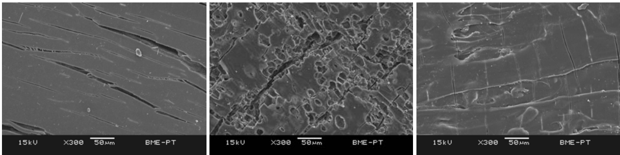
11. ábra PLA (a), PLA/30m% keményítő (b) és PLA/15m% cellulóz (c) felszíne 60°C-os enzimatis bontás után
