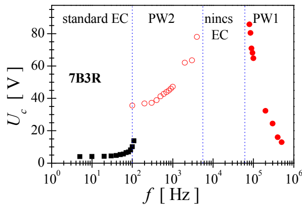
5. ábra. 7B3R eley elektrokonvekciós mintázatai U_c küszöbfeszültségének frekvenciafüggése.
