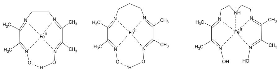
1. ábra. Az [\text{Fe}(\text{Hdmed})]^+ ; [\text{Fe}(\text{Hdmpd})]^+ ; [\text{Fe}(\text{H}_2\text{dmdt})]^{2+} komplexek szerkezete
