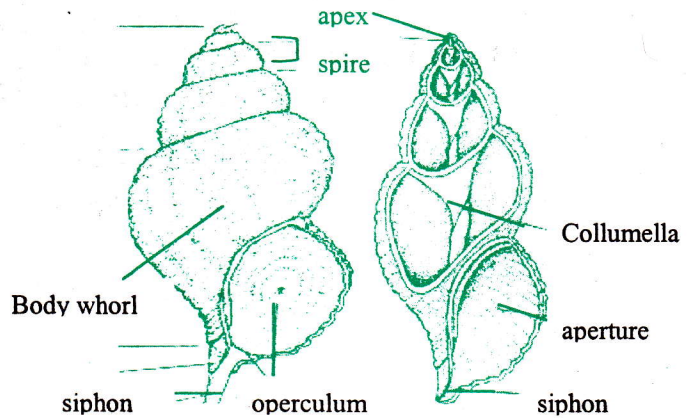
Gambar 1. Struktur dan karakter tipikal cangkang gastropoda (Pechenik, 1991).
