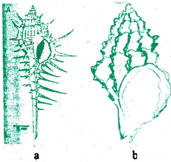
Gambar 3. Tipikal familia muricidae (a) menunjukkan bahwa cangkang mempunyai saluran siphon yang panjang, dengan sederetan spina menuju apex . (gambar bersumber dari Beesley et al (1998). (b) Chicoreus capucinus (skema oleh Karyanto, 2003).
