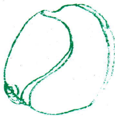
Gambar 6. Cangkang Haminoea sp. Cangkang tersebut memperlihatkan unit whorl dan spire yang mereduksi, serta apertura yang memanjang sehingga mengesankan struktur setangkup (skema oleh Karyanto, 2003)
