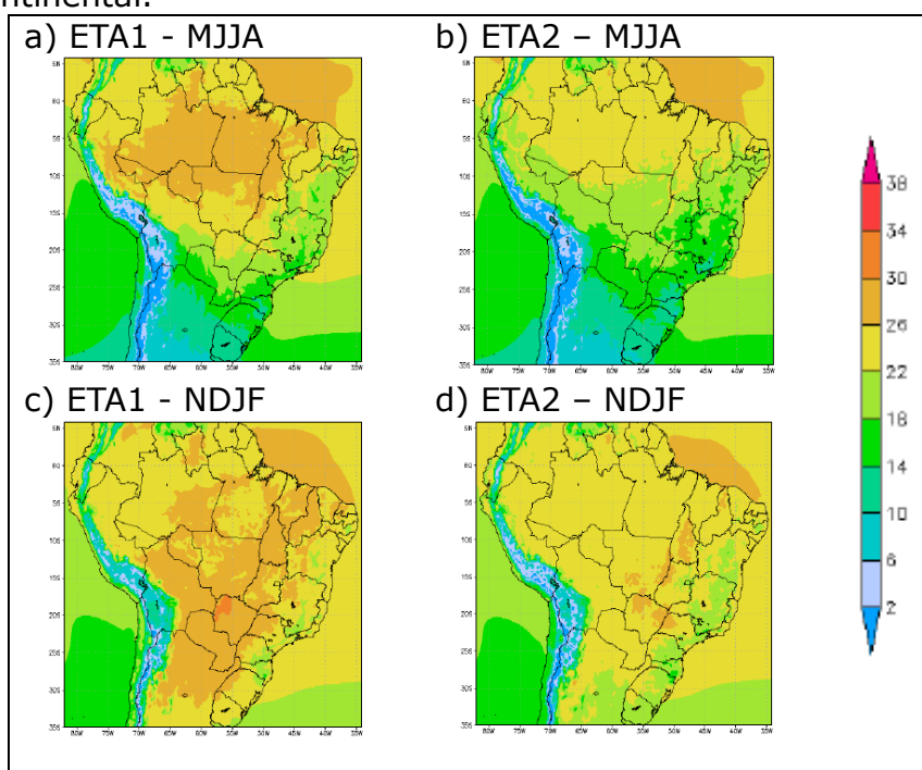
Figura 3. Temperatura a 2 metros da superfície simulada pelo modelo Eta (°C), nos experimentos ETA1 (a, c) e ETA2 (b, d), nas estações secas (a, b) e chuvosas (c, d) de 1979 a 2012
