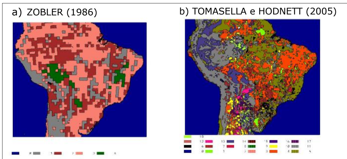
Figura 2. Tipos de solo interpolados para a grade do modelo Eta; a) ETA1 - Mapa com 9 tipos de solo (ZOBLER, 1986), b) ETA2 - Mapa com 26 tipos (TOMASELLA e HODNETT, 2005).
