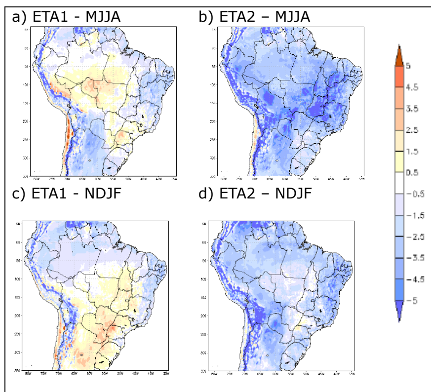
Figura 4. Erro da climatologia da temperatura a 2 metros da superfície (°C), em relação ao CRU, nos experimentos ETA1 (a, c) e ETA2 (b, d), nas estações secas (a, b) e chuvosas (c, d) de 1979 a 2012.
