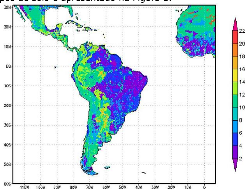
Figura 1. Mapa de solos incorporado no modelo Eta (com 26 tipos de solo) / Fonte: Tomasella e Hodnett (2005).
