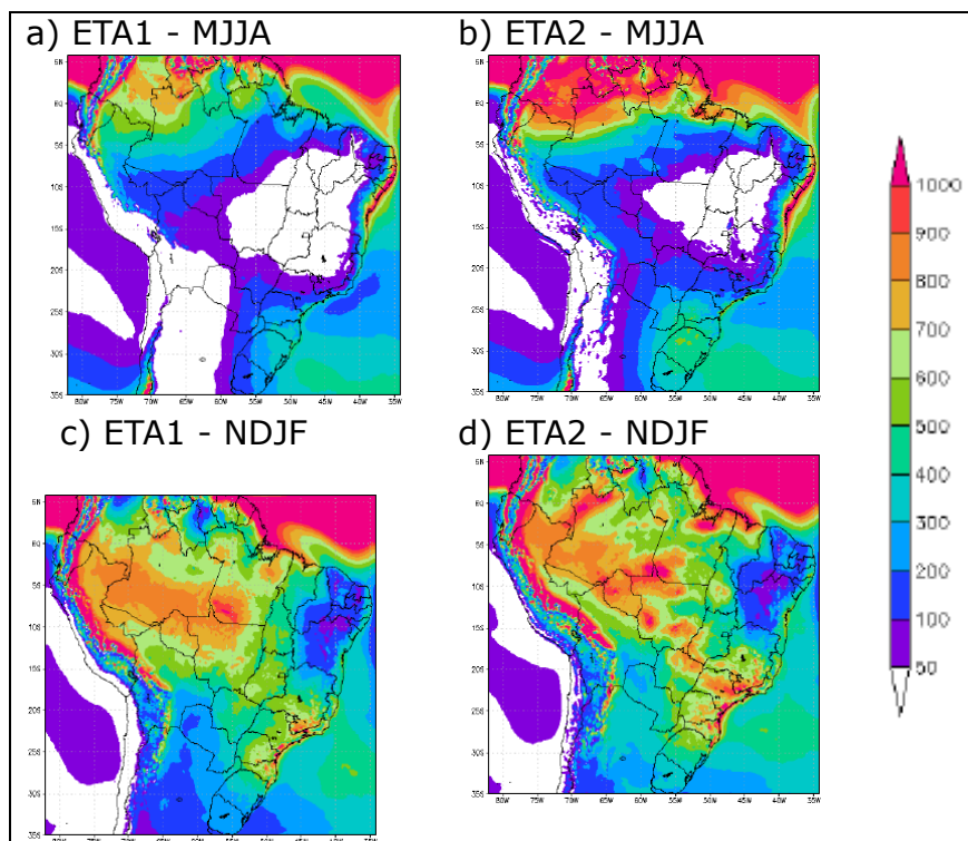
Figura 5. Precipitação simulada pelo modelo Eta (mm/estação), nos experimentos ETA1 (a, c) e ETA2 (b, d), nas estações secas (a, b) e chuvosas (c, d) de 1979 a 2012.
