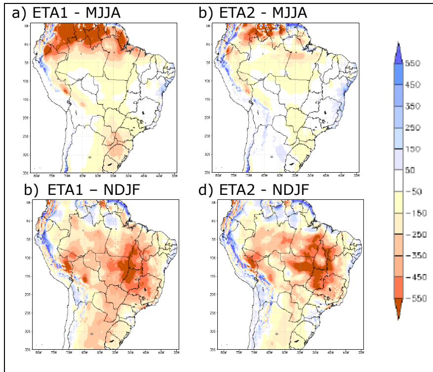
Figura 6. Erro da climatologia da precipitação (mm/estação), em relação ao CRU, nos experimentos ETA1 (a, c) e ETA2 (b, d), nas estações secas (a, b) e chuvosas (c, d) de 1979 a 2012.
