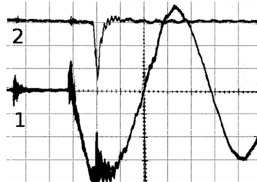
Рис. 2. Осциллограммы импульсов
